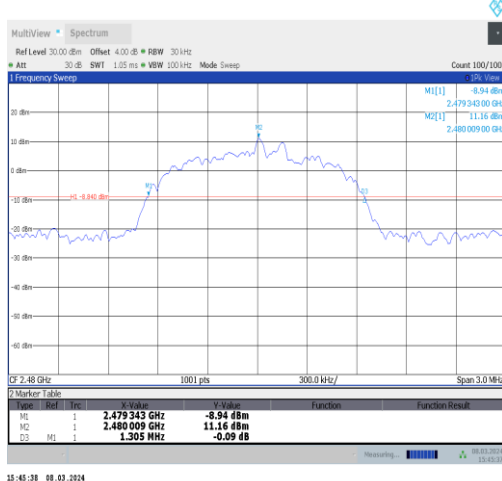
3DH5-Ant10-2480
