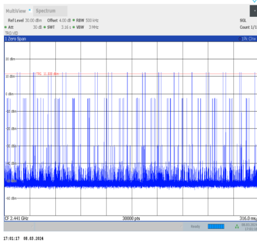
2DH1-Ant10-Hop-PASS
