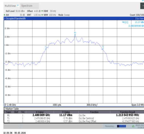
2DH5-Ant10-2480
