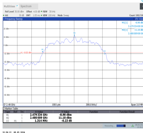
2DH5-Ant10-2480
