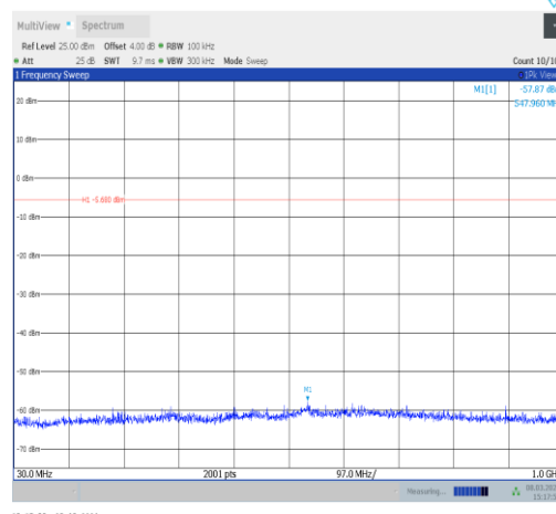
DH5-Ant10-2480-30~1000-PASS
