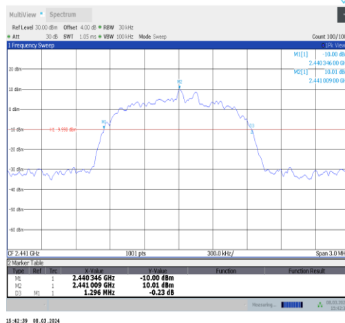
3DH5-Ant10-2441
