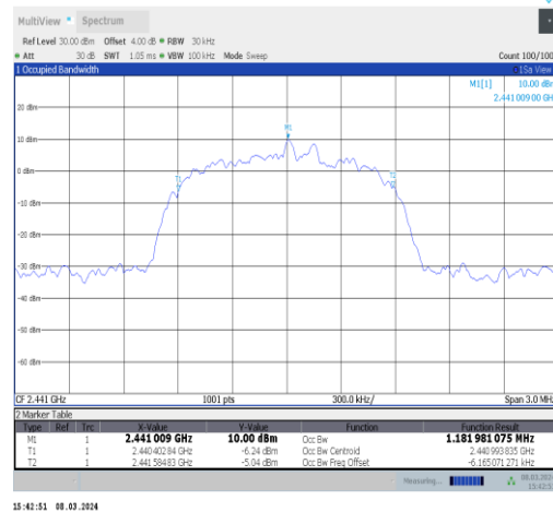
3DH5-Ant10-2441
