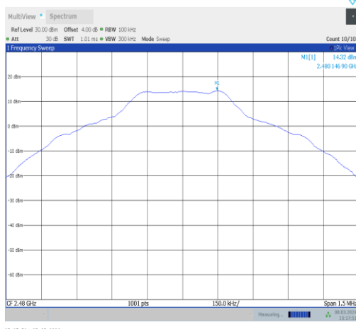
DH5-Ant10-2480-0~Reference-PASS
