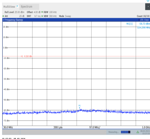
2DH5-Ant10-2402-30~1000-PASS
