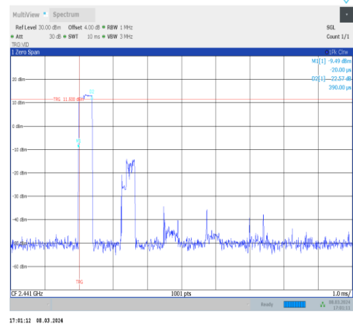
2DH1-Ant10-Hop-PASS
