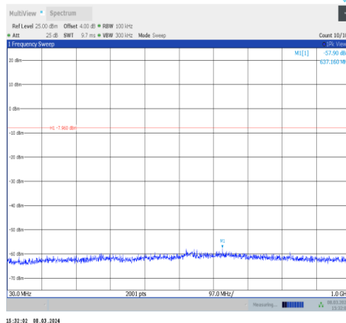
2DH5-Ant10-2441-30~1000-PASS
