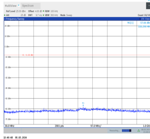
3DH5-Ant10-2402-30~1000-PASS
