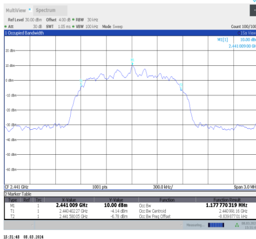
2DH5-Ant10-2441
