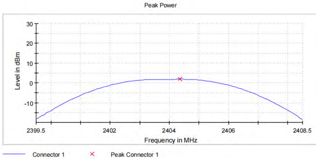
BLE_2M_Ant0_2404
