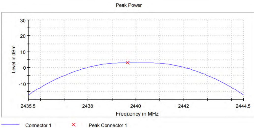
BLE_2M_Ant0_2440
