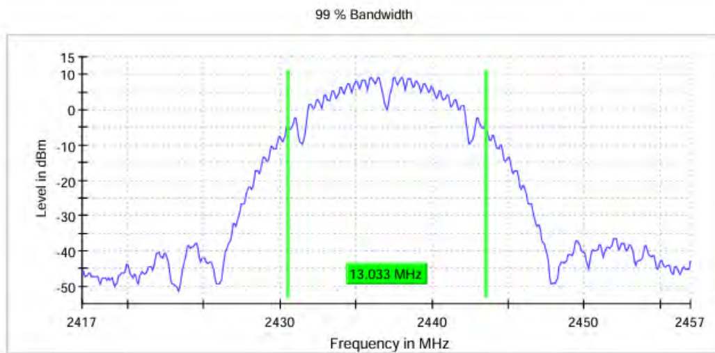
11B_Ant0_2437
