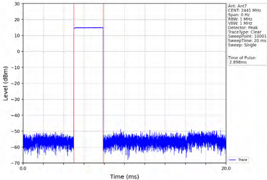
GFSK_DH5_HOPP_Ant7_NTNV
