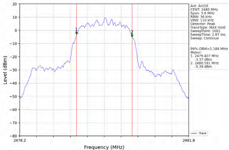
Pi/4DQPSK_2DH5_HCH_2480MHz_Ant16_NTNV
