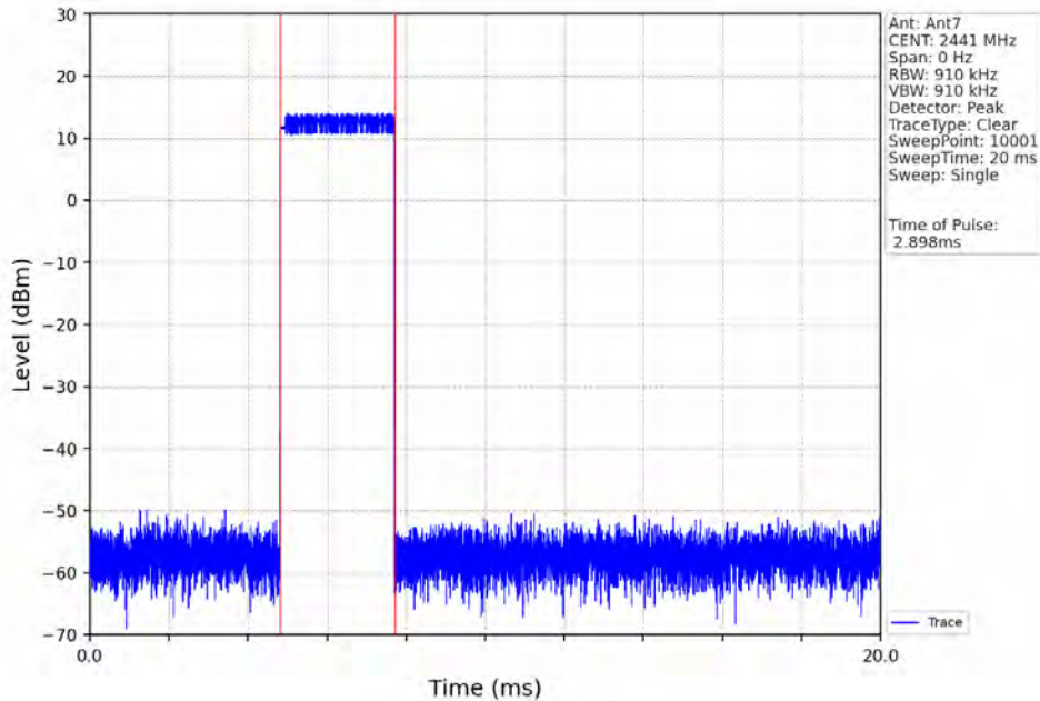
Pi/4DQPSK_2DH5_HOPP_Ant7_NTNV
