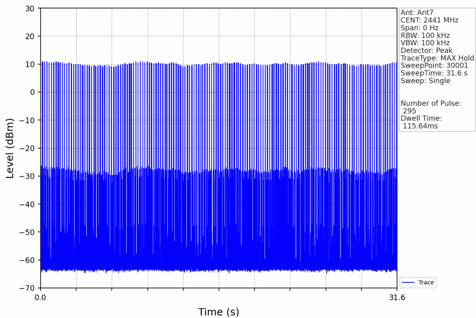
Pi/4DQPSK_2DH1_HOPP_Ant7_NTNV
