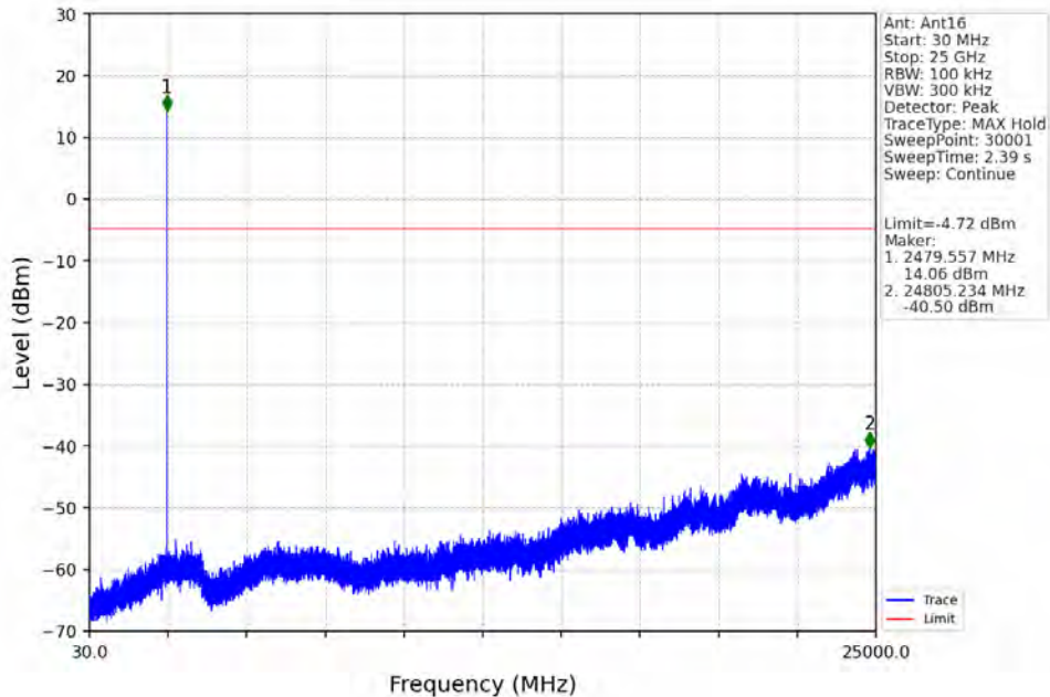
GFSK_DH5_HOPP_Ant16_NTNV
