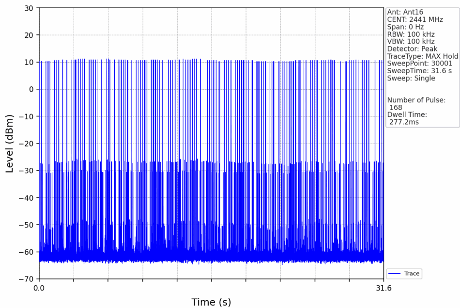
Pi/4DQPSK_2DH3_HOPP_Ant16_NTNV
