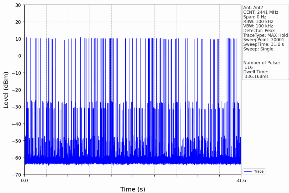
Pi/4DQPSK_2DH5_HOPP_Ant7_NTNV
