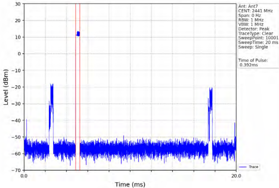
Pi/4DQPSK_2DH1_HOPP_Ant7_NTNV
