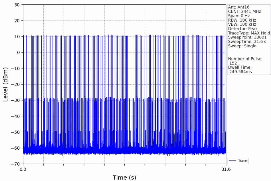
8DPSK_3DH3_HOPP_Ant16_NTNV
