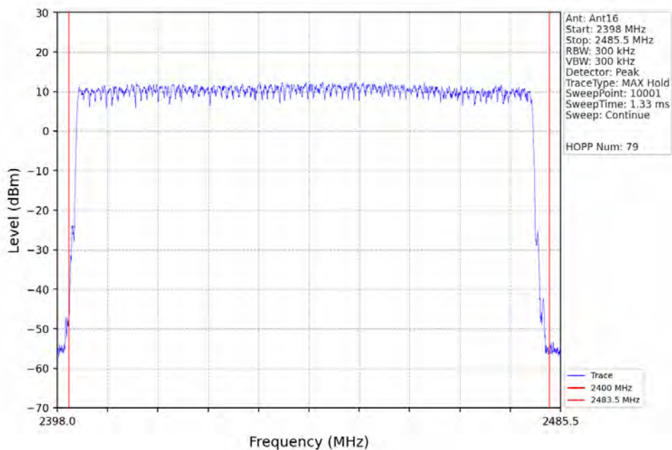
8DPSK_3DH5_HOPP_Ant16_NTNV
