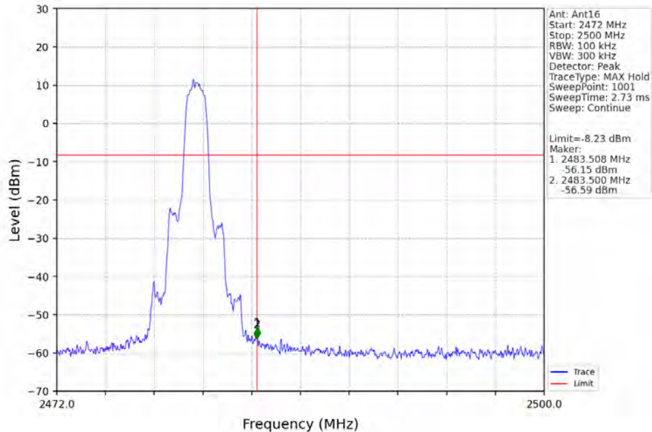
Pi/4DQPSK_2DH5_HCH_2480MHz_Ant16_NTNV
