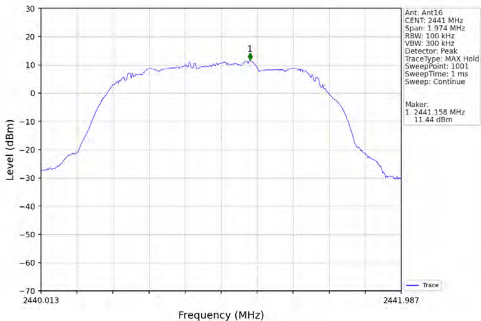
8DPSK_3DH5_MCH_2441MHz_Ant16_NTNV
