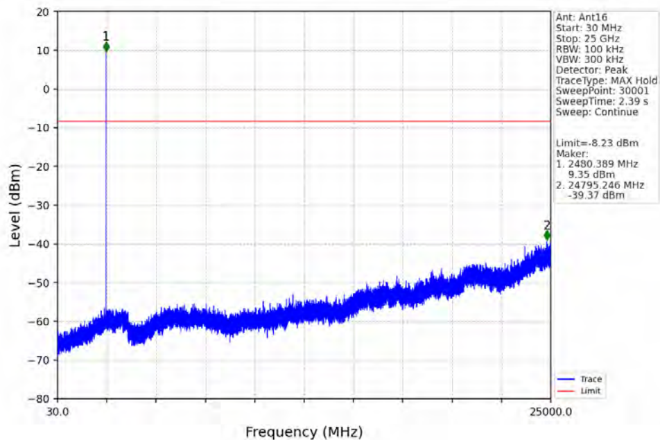
Pi/4DQPSK_2DH5_HCH_2480MHz_Ant16_NTNV
