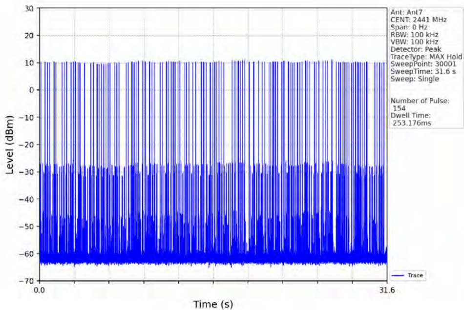
Pi/4DQPSK_2DH3_HOPP_Ant7_NTNV
