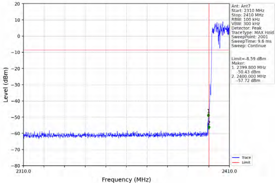
Pi/4DQPSK_2DH5_HOPP_Ant7_NTNV
