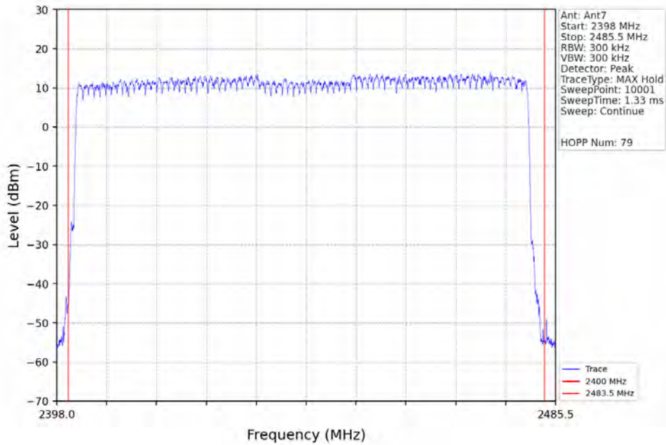
8DPSK_3DH5_HOPP_Ant7_NTNV
