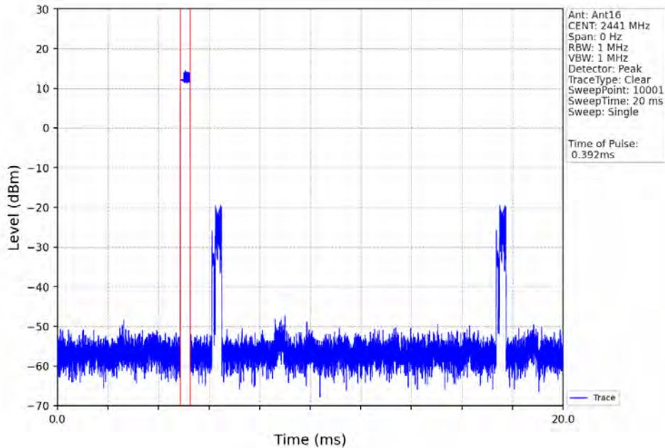
Pi/4DQPSK_2DH1_HOPP_Ant16_NTNV
