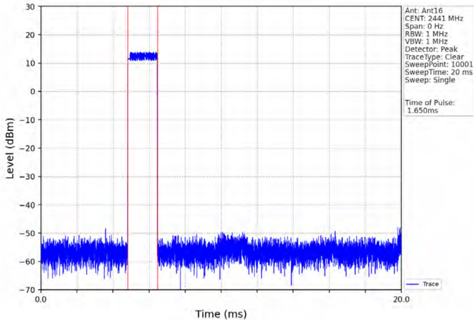
Pi/4DQPSK_2DH3_HOPP_Ant16_NTNV
