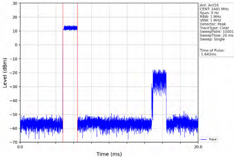
8DPSK_3DH3_HOPP_Ant16_NTNV
