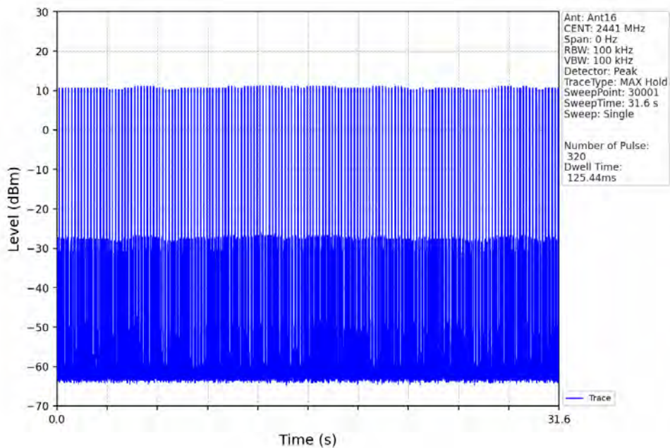
Pi/4DQPSK_2DH1_HOPP_Ant16_NTNV
