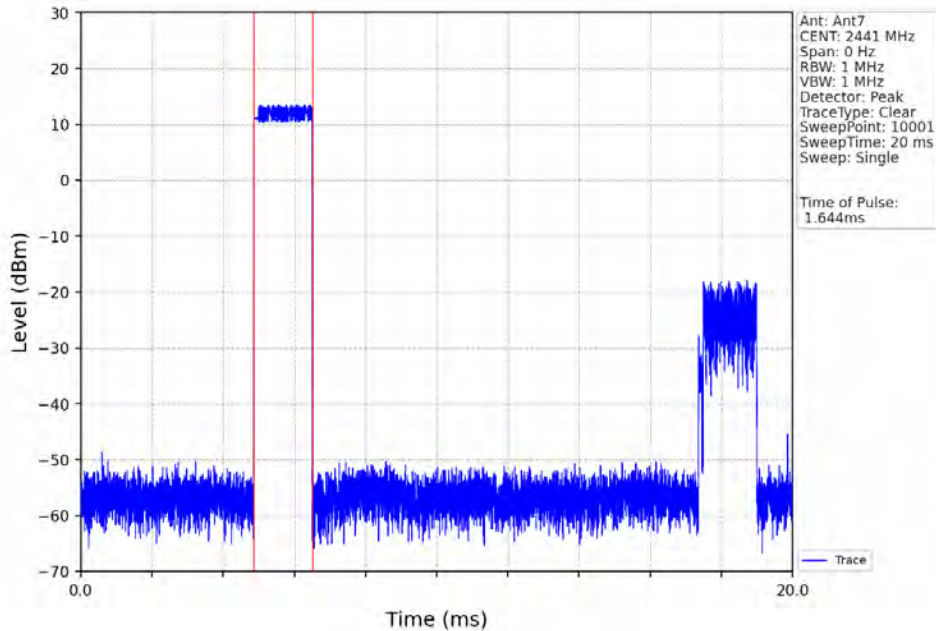
Pi/4DQPSK_2DH3_HOPP_Ant7_NTNV
