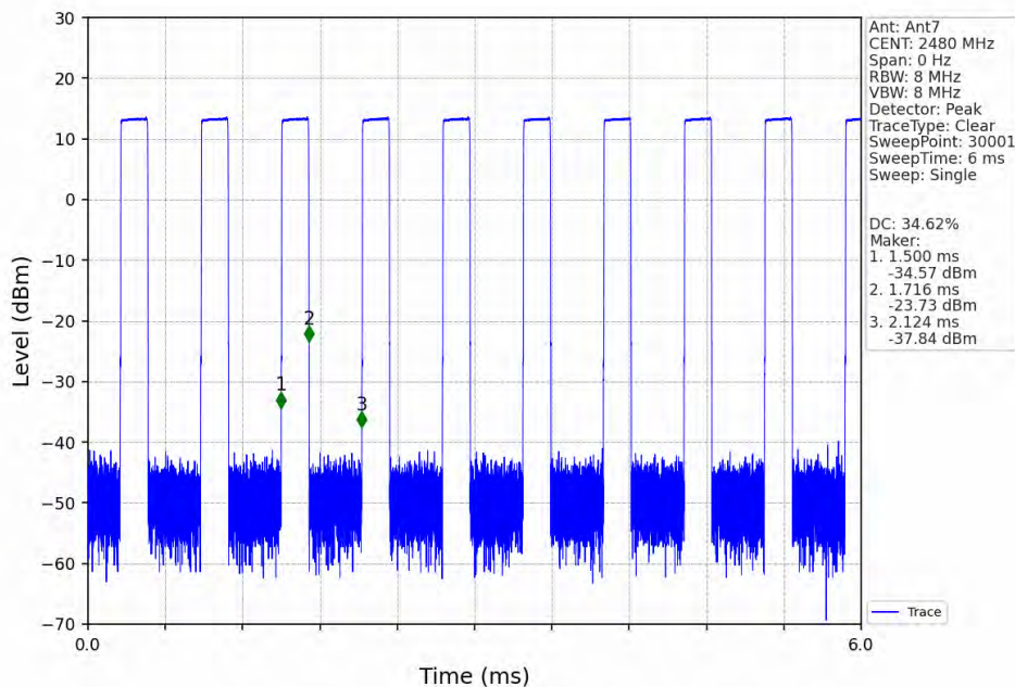
2M_HCH_2480MHz_Ant7_NTNV
