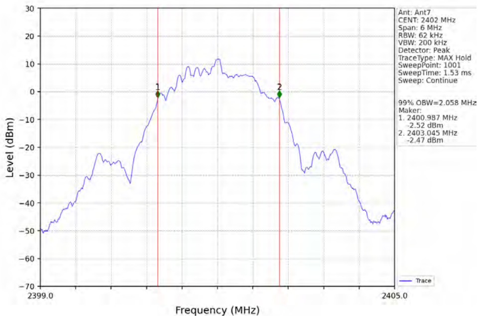
2M_LCH_2402MHz_Ant7_NTNV
