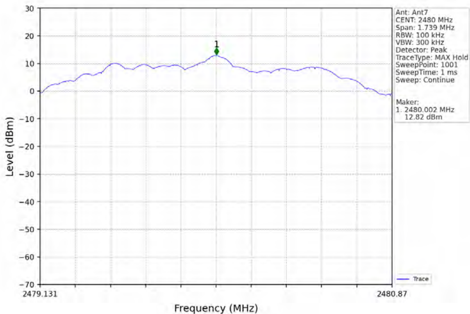
2M_HCH_2480MHz_Ant7_NTNV
