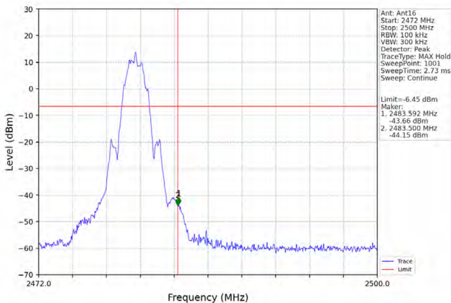
2M_HCH_2480MHz_Ant16_NTNV
