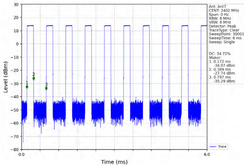
2M_LCH_2402MHz_Ant7_NTNV
