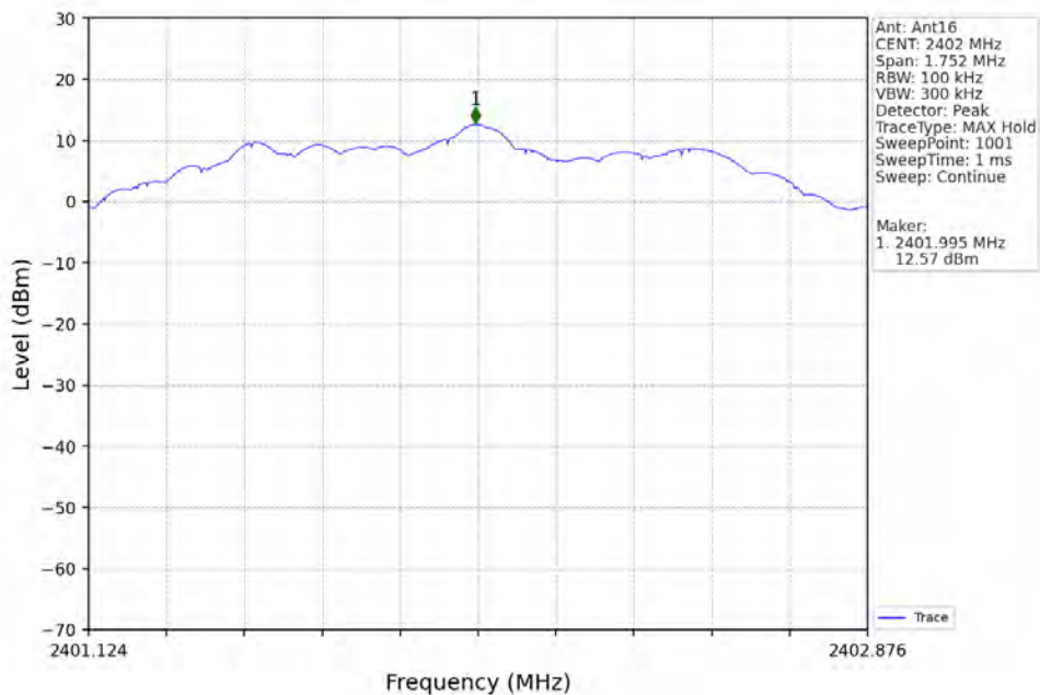
2M_LCH_2402MHz_Ant16_NTNV
