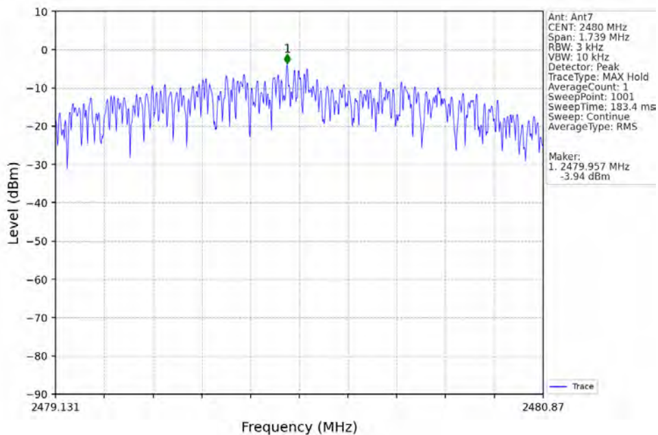
2M_HCH_2480MHz_Ant7_NTNV
