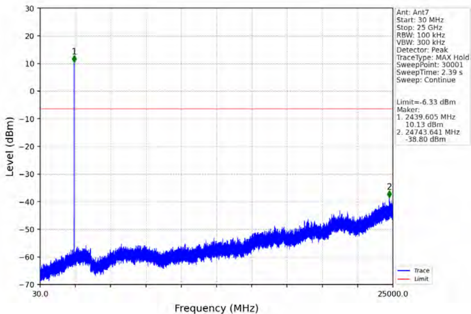
2M_MCH_2440MHz_Ant7_NTNV
