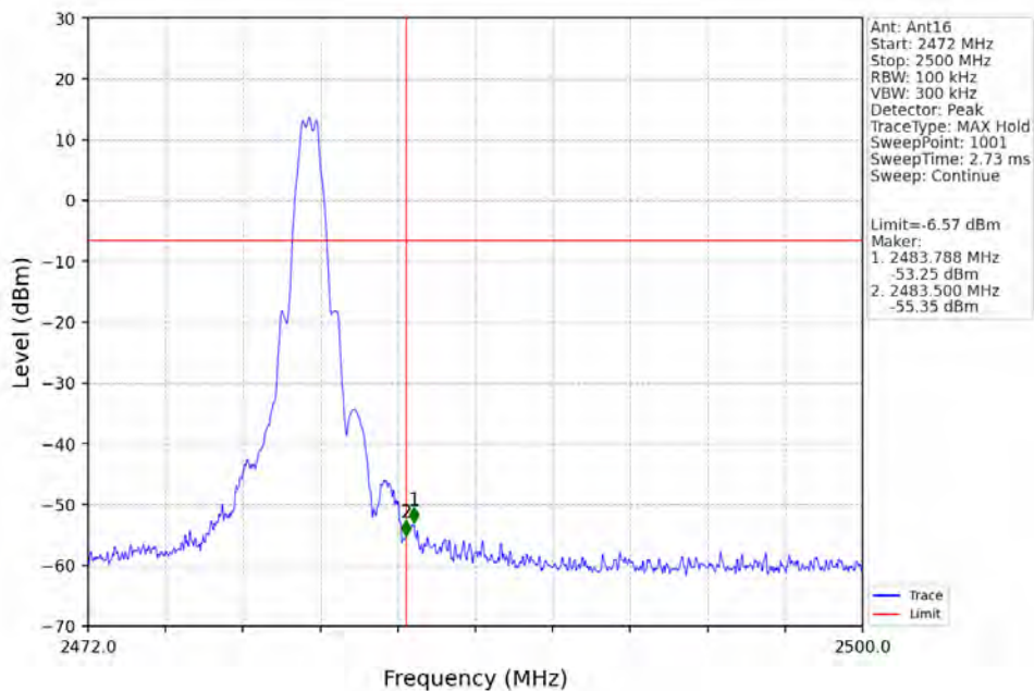
1M_HCH_2480MHz_Ant16_NTNV
