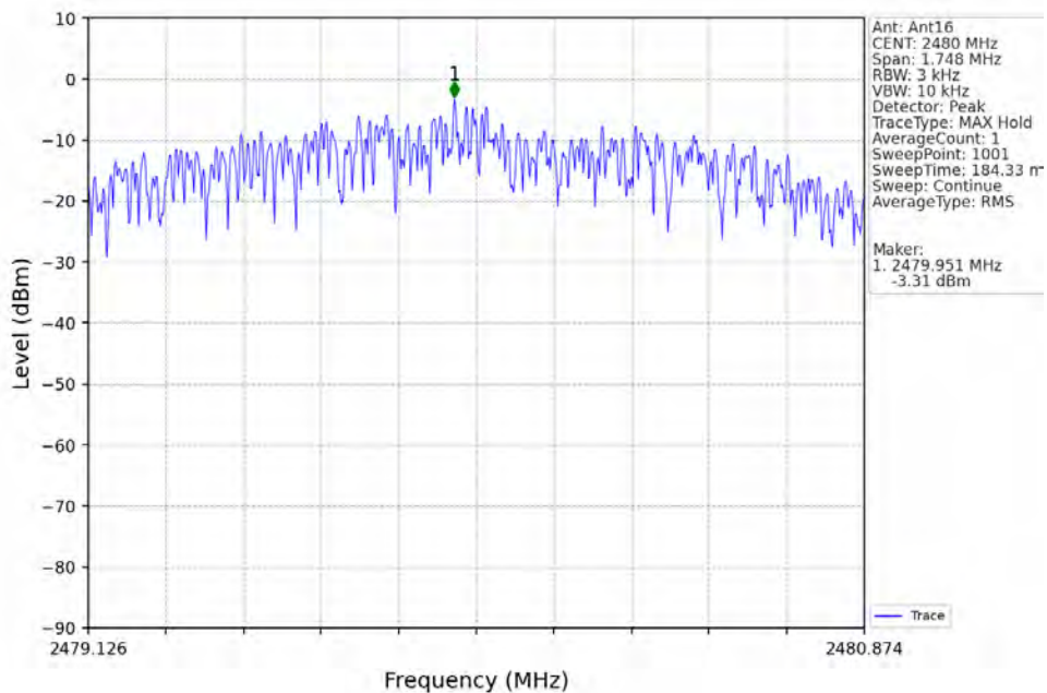
2M_HCH_2480MHz_Ant16_NTNV
