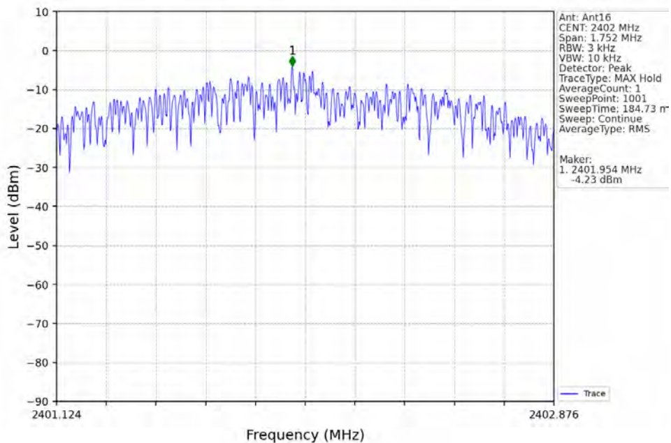
2M_LCH_2402MHz_Ant16_NTNV
