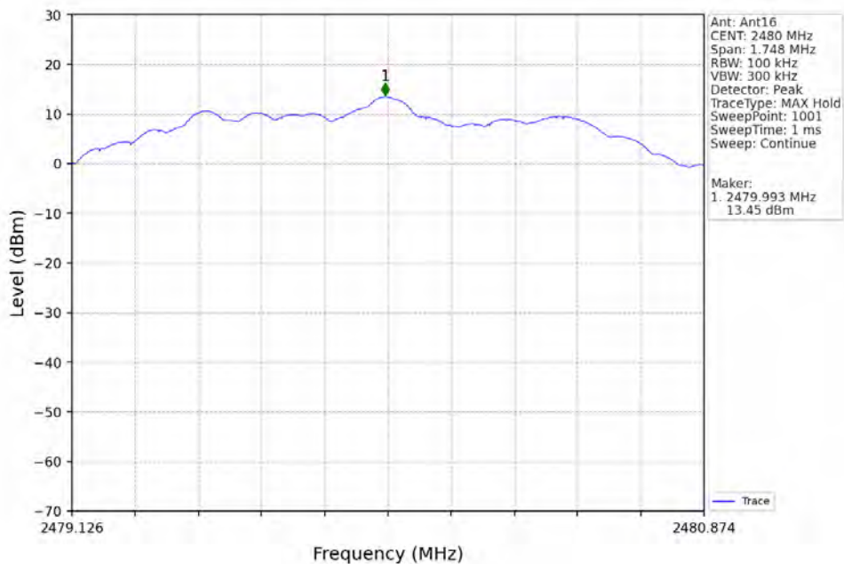
2M_HCH_2480MHz_Ant16_NTNV
