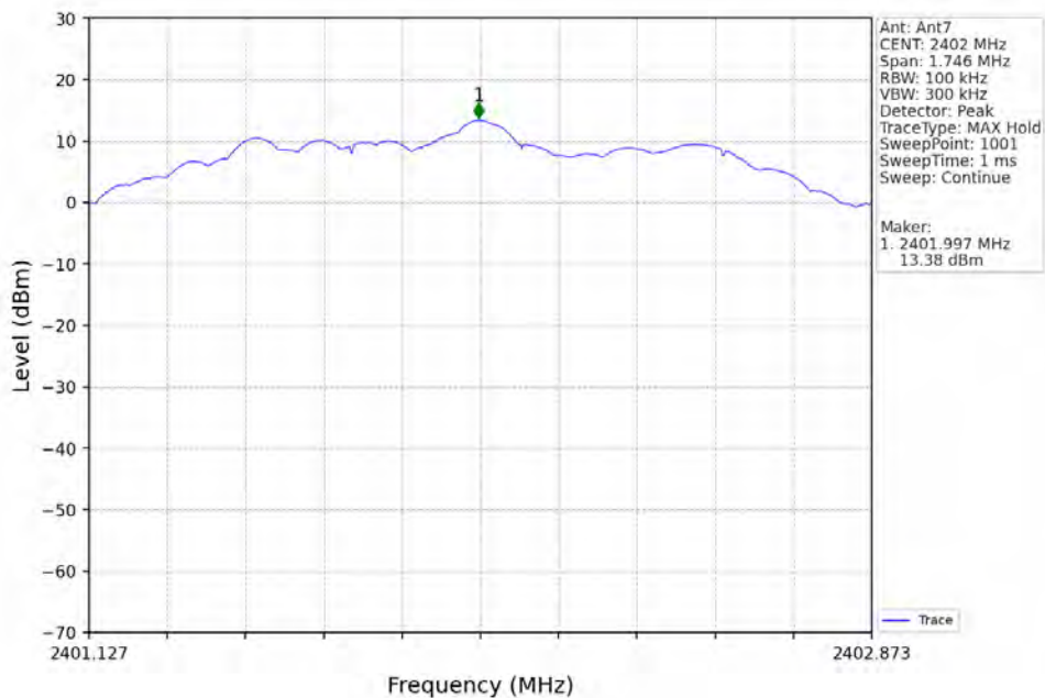
2M_LCH_2402MHz_Ant7_NTNV
