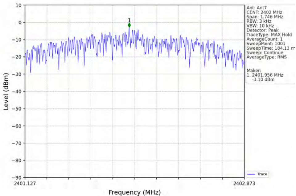
2M_LCH_2402MHz_Ant7_NTNV
