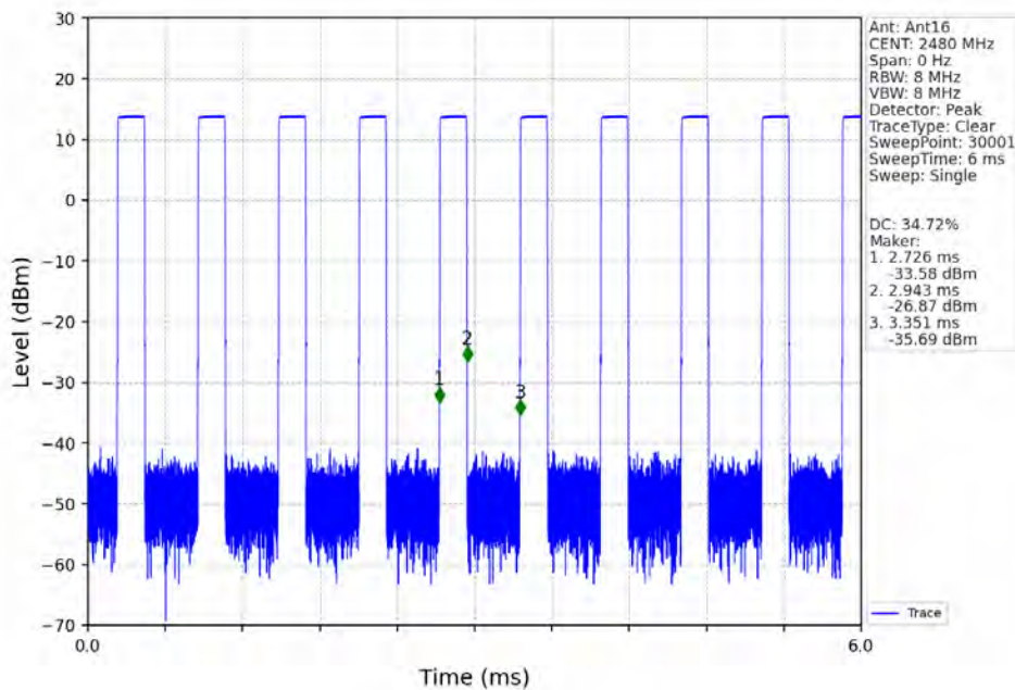
2M_HCH_2480MHz_Ant16_NTNV
