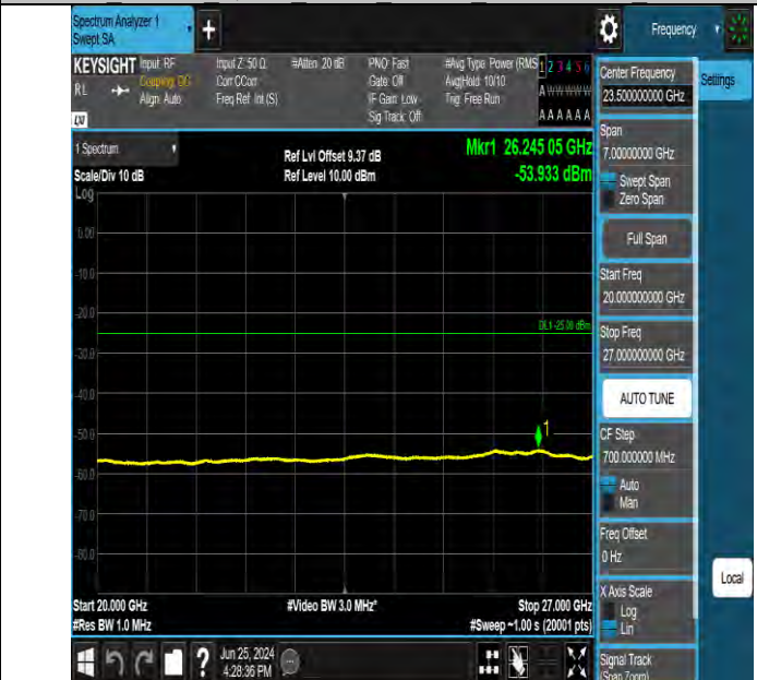
Band7 15MHz QPSK 21100 1RB#0 20000~27000 20000~27000
