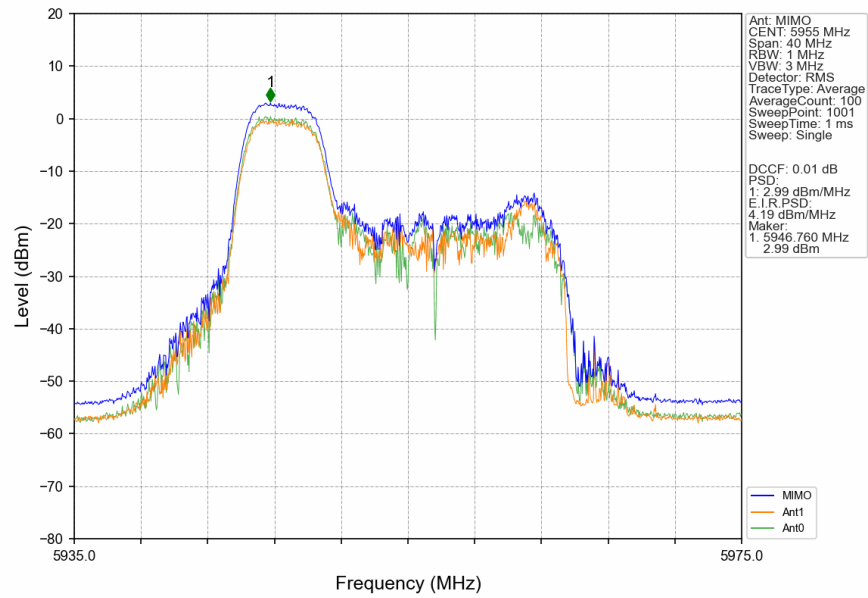
802.11be(EHT20) LCH 5955MHz RU52 Left MIMO NTN
