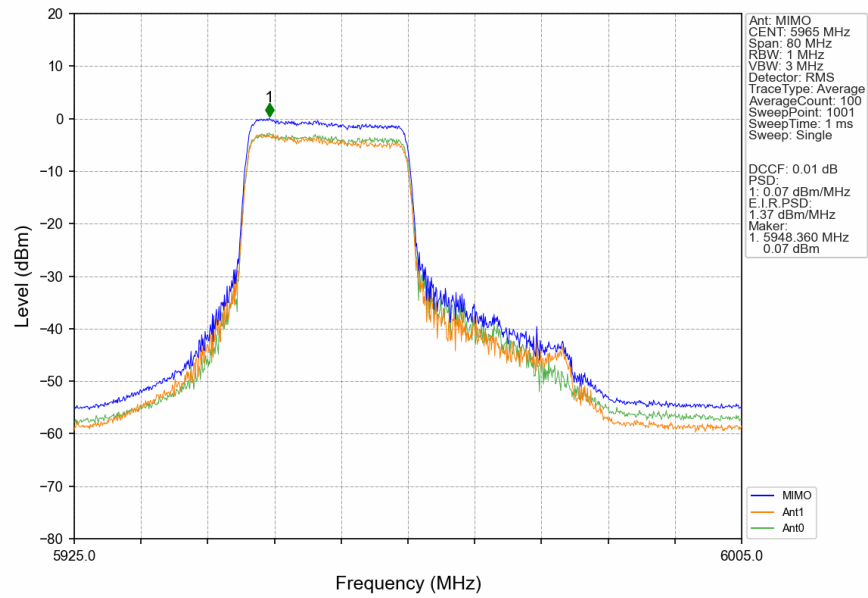
802.11be(EHT40) LCH_5965MHz_RU242_Left_MIMO_NTNV
