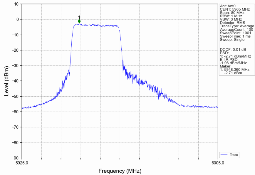
802.11be(EHT40) LCH_5965MHz_RU242_Left_MIMO_NTNV
