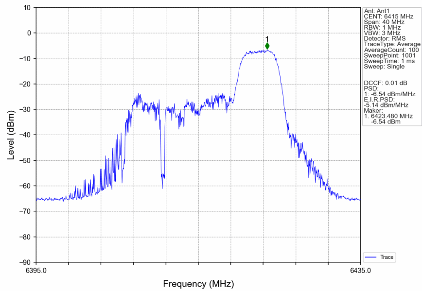
802.11be(EHT20)_HCH_6415MHz_RU52_Right_Ant1_NTNV
