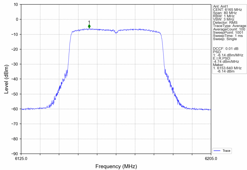
802.11be(EHT40)_MCH_6165MHz_RU484_Left_Ant1_NTNV
