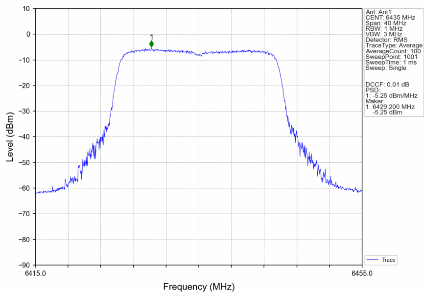
802.11be(EHT20)_LCH_6435MHz_RU242_Left_Ant1_NTNV
