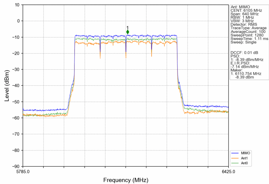
802.11be(EHT320)_LCH_6105MHz_4xRU996_Left_MIMO_NTNV
