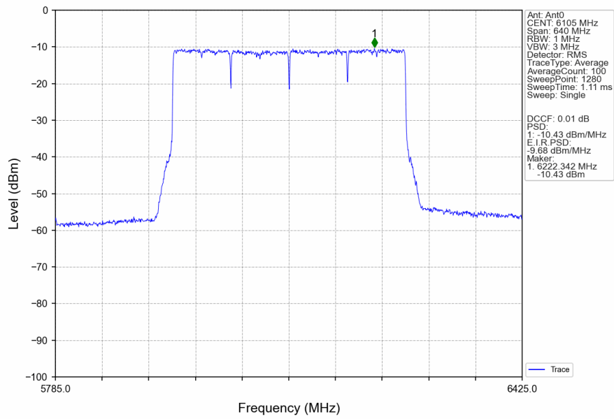
802.11be(EHT320)_LCH_6105MHz_4xRU996_Left_MIMO_NTNV
