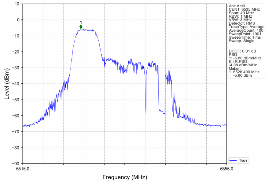
802.11be(EHT20)_LCH_6535MHz_RU52_Left_MIMO_NTNV
