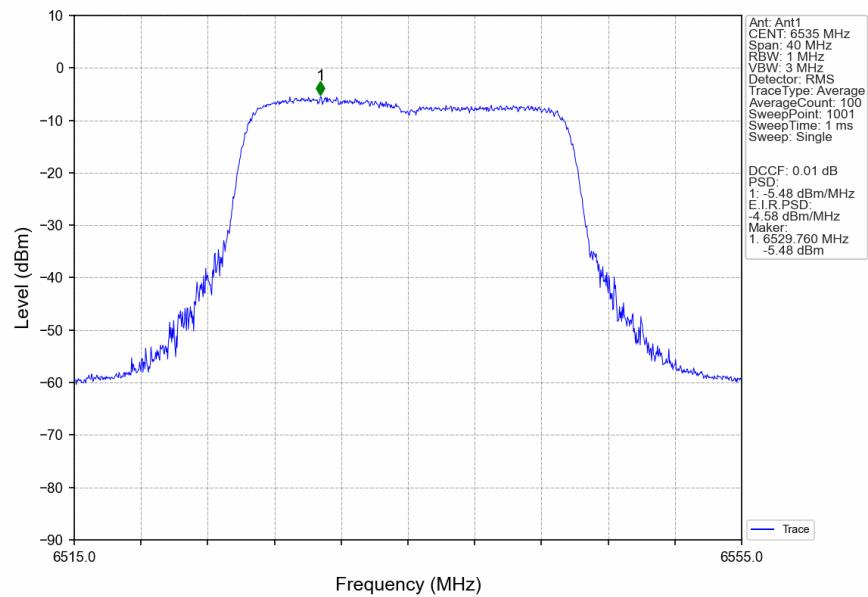
802.11be(EHT20)_LCH_6535MHz_RU242_Left_Ant1_NTNV
