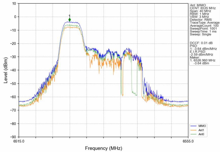
802.11be(EHT20)_LCH_6535MHz_RU52_Left_MIMO_NTNV
