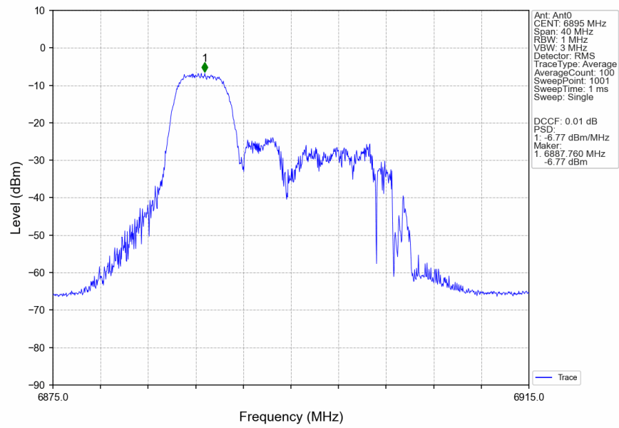
802.11be(EHT20)_LCH_6895MHz_RU52_Left_MIMO_NTNV
