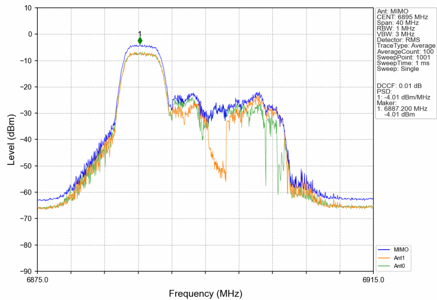
802.11be(EHT20)_LCH_6895MHz_RU52_Left_MIMO_NTNV
