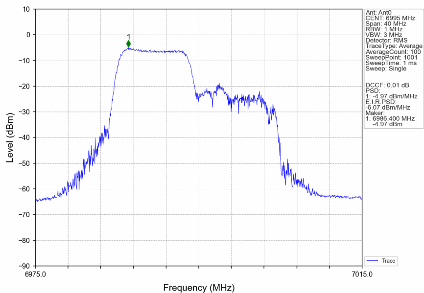
802.11be(EHT20)_MCH_6995MHz_RU106_Left_MIMO_NTNV
