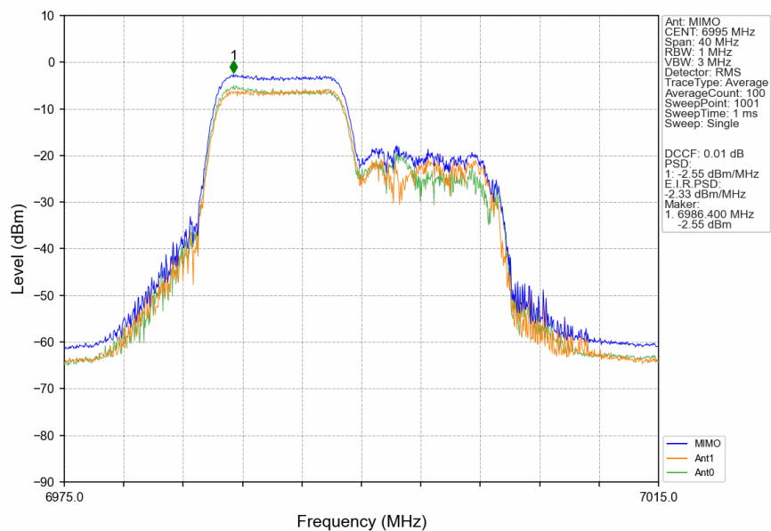
802.11be(EHT20)_MCH_6995MHz_RU106_Left_MIMO_NTNV
