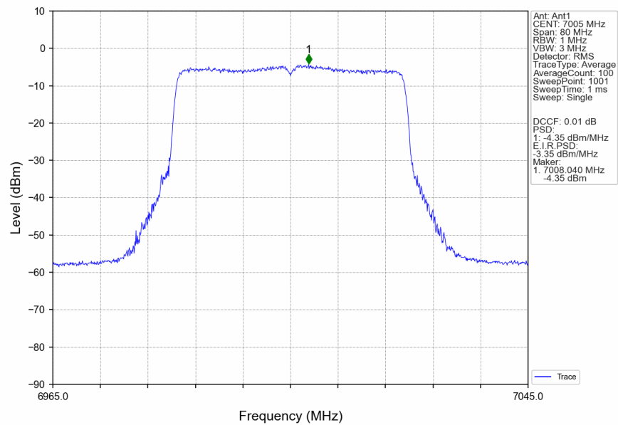
802.11be(EHT40)_MCH_7005MHz_RU484_Left_Ant1_NTNV
