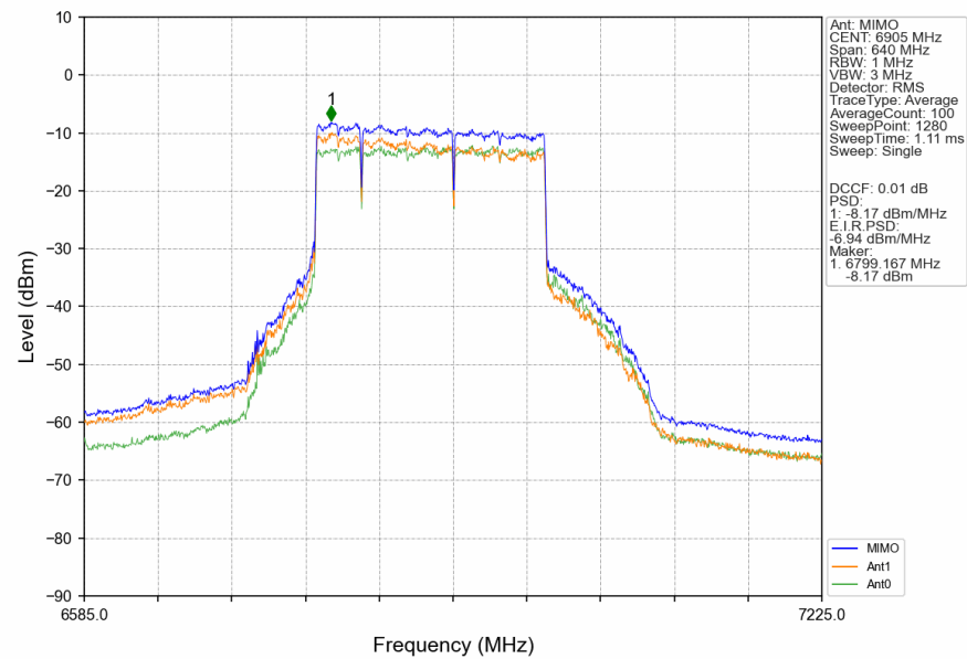
802.11be(EHT320)_HCH_6905MHz_2xRU996_Right_MIMO_NTNV
