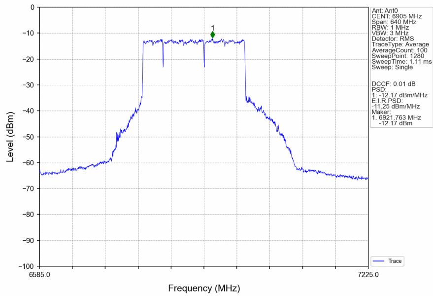
802.11be(EHT320)_HCH_6905MHz_2xRU996_Right_MIMO_NTNV
