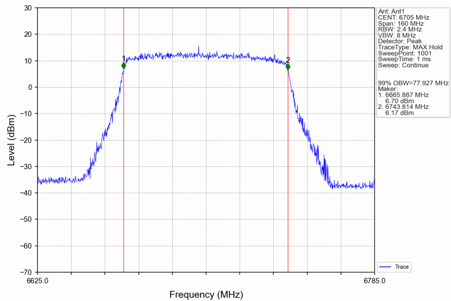
802.11be(EHT80)_MCH_6705MHz_RU996_Left_Ant1_NTNV
