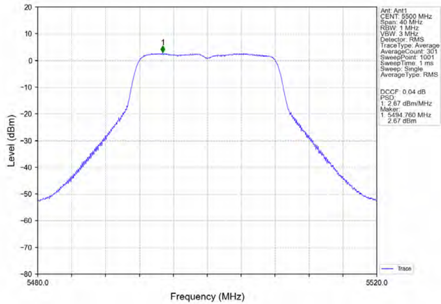
802.11a LCH_5500MHz_Ant1_NTNV
