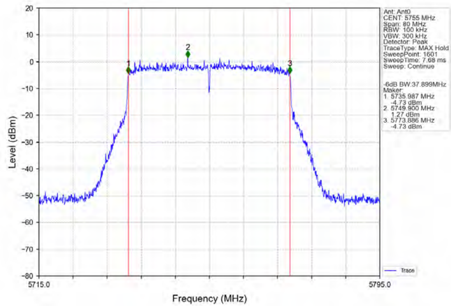
802.11ax(HEW40)_LCH_5755MHz_RU484_Left_Ant0_NTNV
