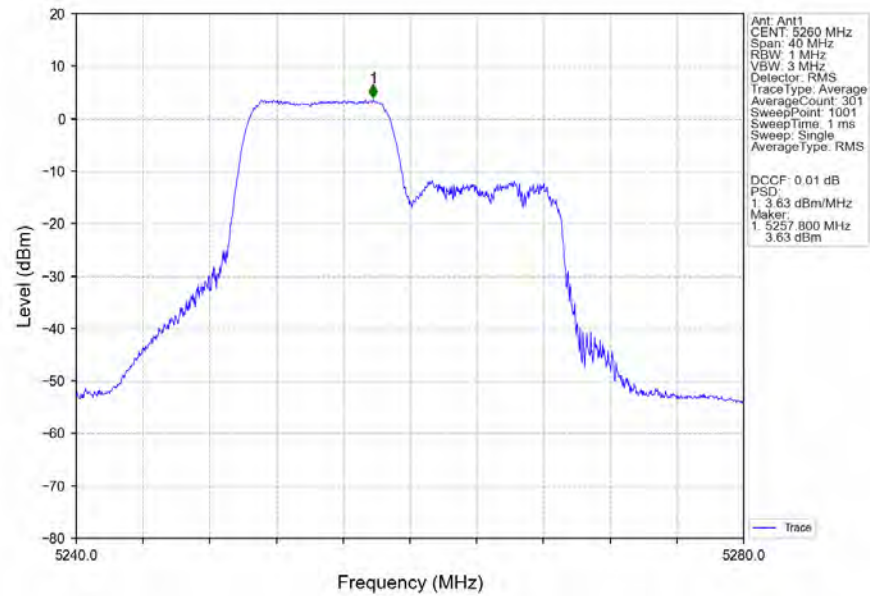
802.11be(EHT20)_LCH_5260MHz_RU106_Left_MIMO_NTNV
