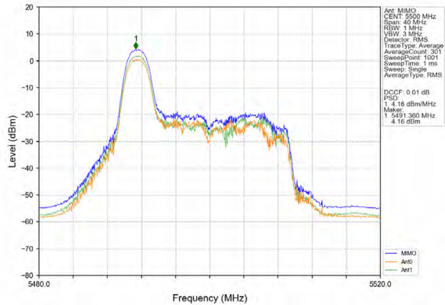
802.11be(EHT20) LCH_5500MHz_RU52_Left_Ant0_NTNV
