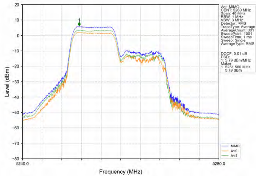
802.11be(EHT20)_LCH_5260MHz_RU106_Left_MIMO_NTNV
