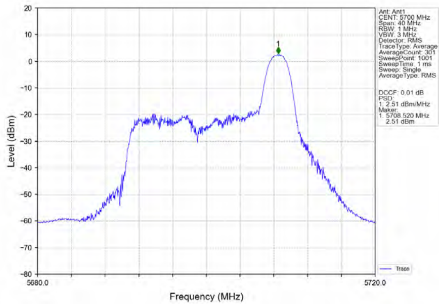
802.11be(EHT20) HCH_5700MHz_RU26_Right_Ant1_NTNV
