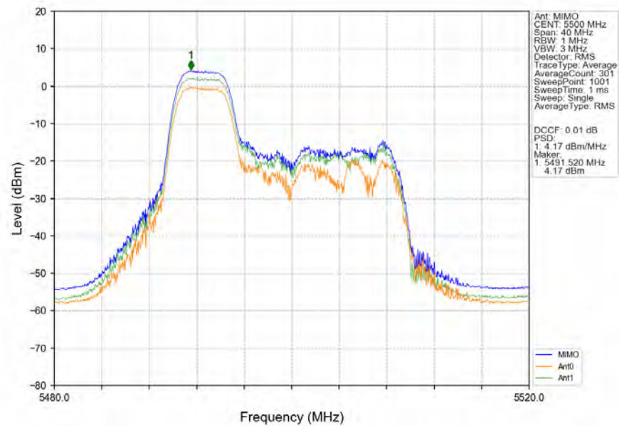
802.11be(EHT20) LCH_5500MHz_RU52_Left_MIMO_NTNV
