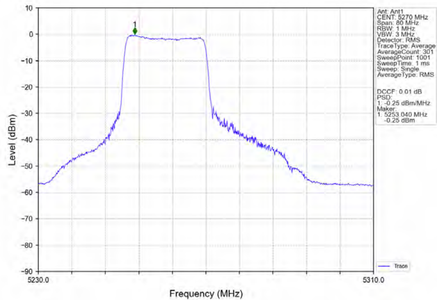
802.11be(EHT40) LCH_5270MHz_RU242_Left_Ant1_NTNV
