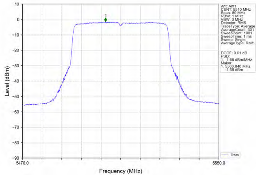
802.11be(EHT40)_LCH_5510MHz_RU484_Left_MIMO_NTNV
