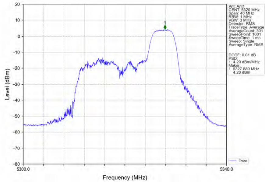
802.11be(EHT20) HCH_5320MHz_RU52_Right_Ant1_NTNV
