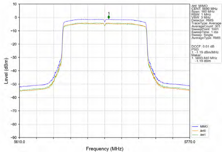
802.11be(EHT80)_HCH_5690MHz_RU996_Left_MIMO_NTNV
