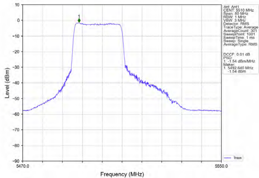
802.11be(EHT40) LCH_5510MHz_RU242_Left_Ant1_NTNV
