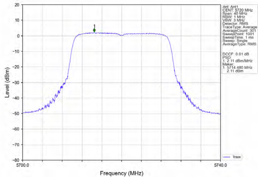
802.11be(EHT20) HCH 5720MHz RU242 Left Ant1 NTN
