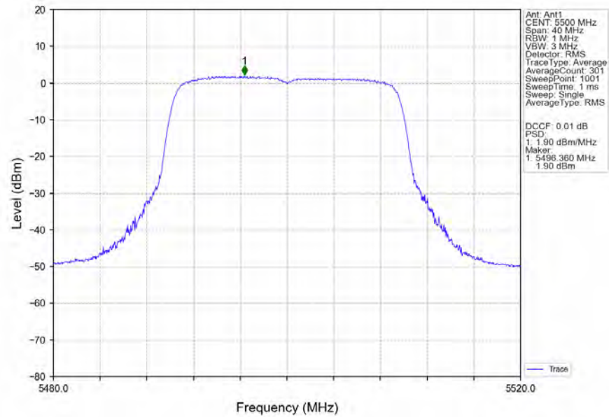
802.11be(EHT20) LCH_5500MHz_RU242_Left_MIMO_NTNV
