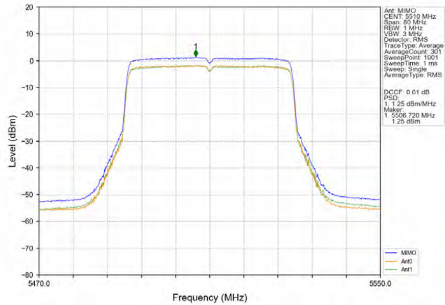
802.11be(EHT40)_LCH_5510MHz_RU484_Left_MIMO_NTNV
