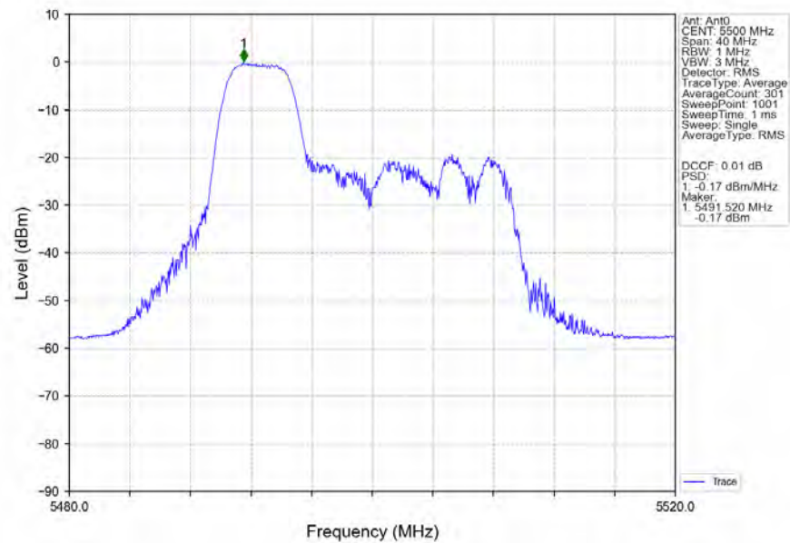
802.11be(EHT20) LCH_5500MHz_RU52_Left_Ant0_NTNV
