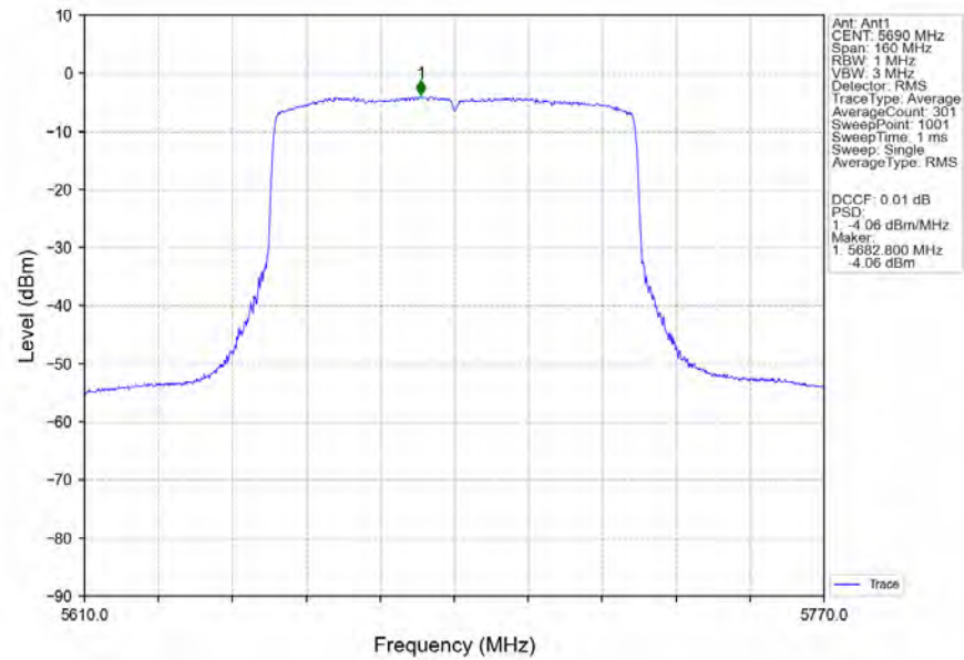
802.11be(EHT80)_HCH_5690MHz_RU996_Left_MIMO_NTNV
