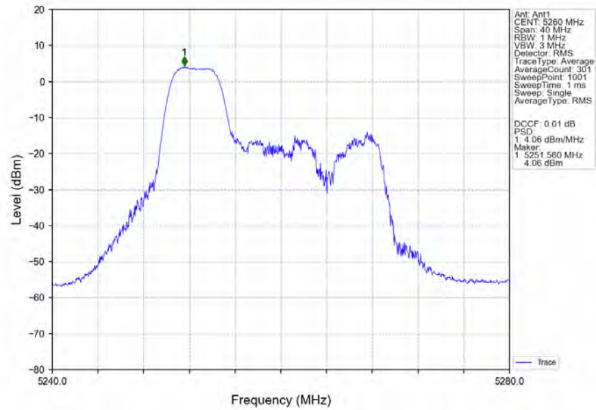
802.11be(EHT20)_LCH_5260MHz_RU52_Left_Ant1_NTNV
