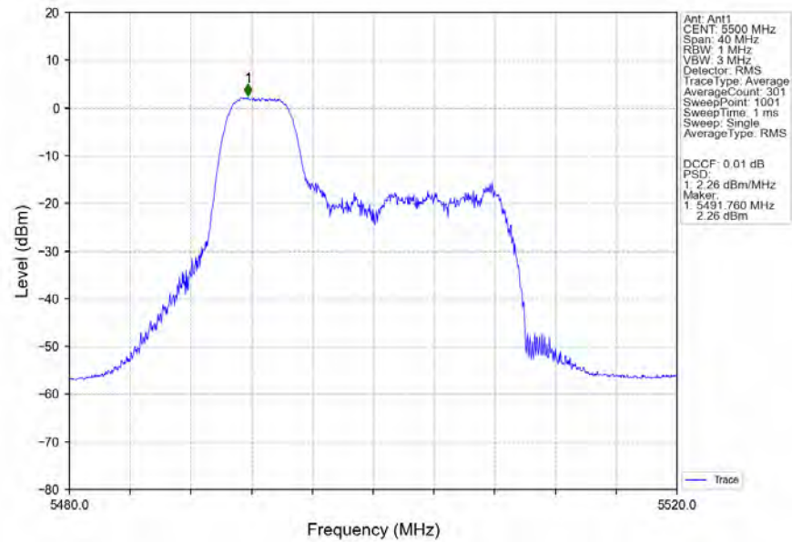
802.11be(EHT20) LCH_5500MHz_RU52_Left_MIMO_NTNV
