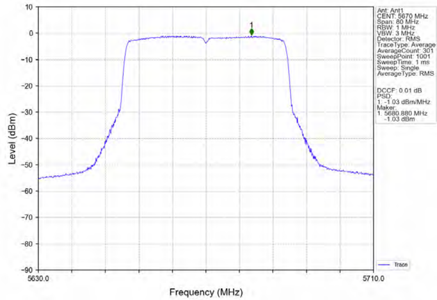
802.11be(EHT40)_HCH_5670MHz_RU484_Left_MIMO_NTNV
