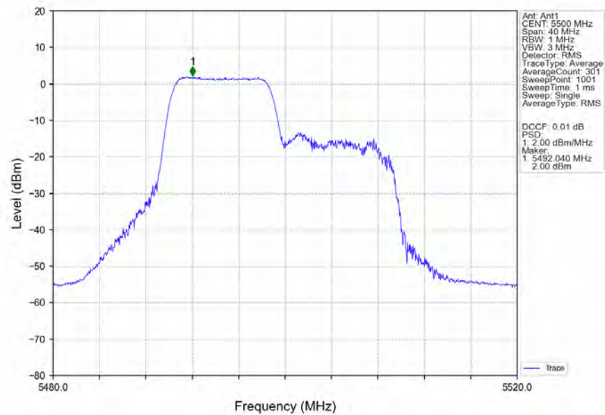
802.11be(EHT20) LCH_5500MHz_RU106_Left_Ant1_NTNV
