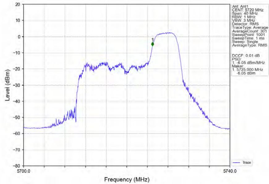
802.11be(EHT20) HCH_5720MHz_RU52_Right_Ant1_NTNV
