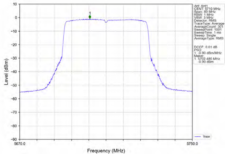
802.11be(EHT40) HCH_5710MHz_RU484_Left_Ant1_NTNV
