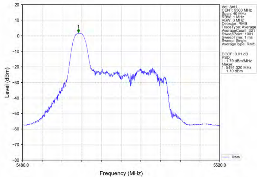
802.11be(EHT20)_LCH_5500MHz_RU26_Left_Ant1_NTNV
