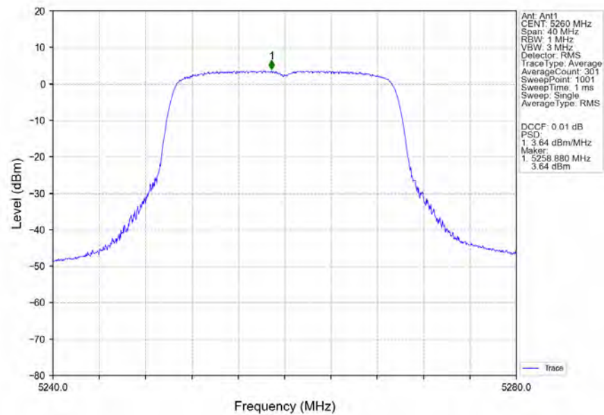
802.11be(EHT20)_LCH_5260MHz_RU242_Left_Ant1_NTNV
