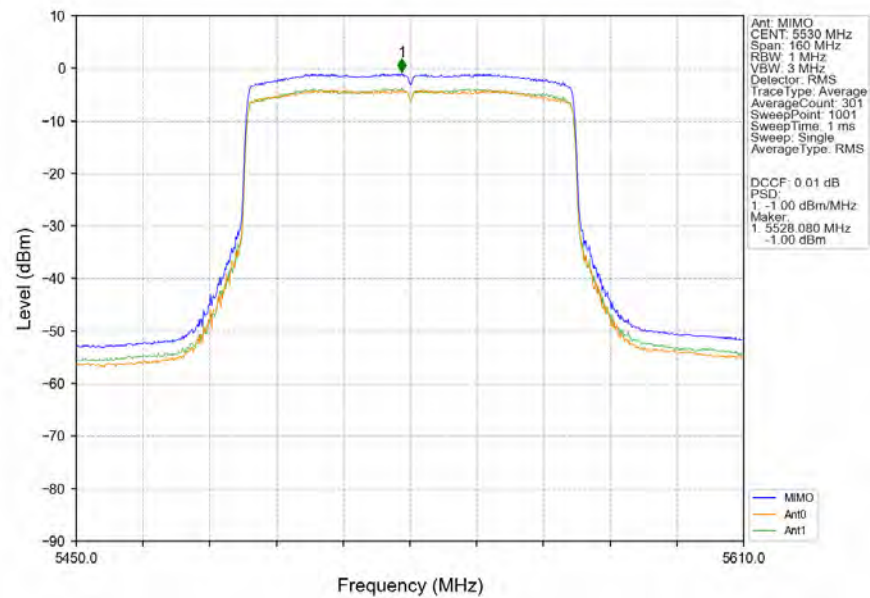
802.11be(EHT80) LCH_5530MHz_RU996_Left_MIMO_NTNV
