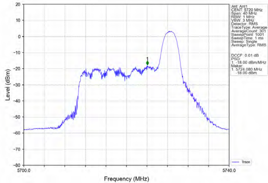
802.11be(EHT20)_HCH_5720MHz_RU26_Right_MIMO_NTNV
