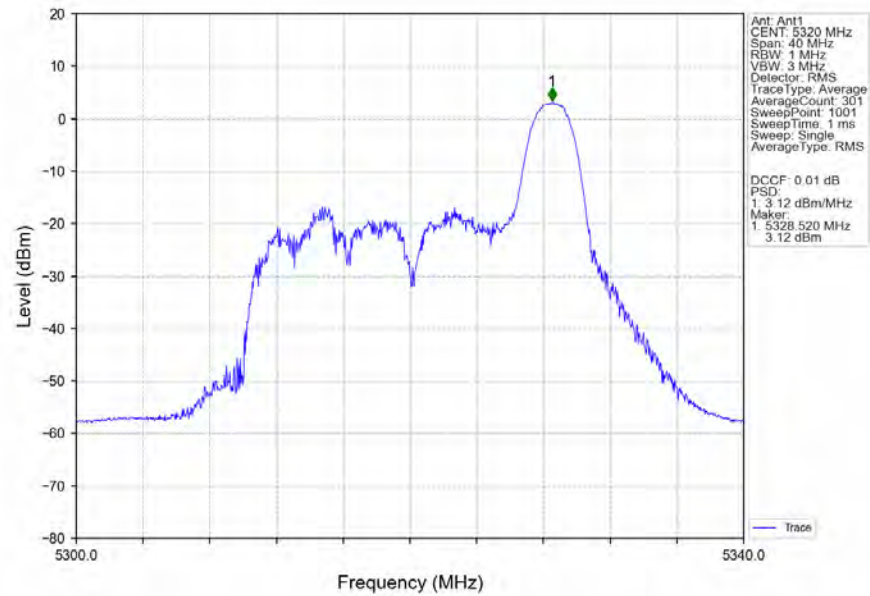
802.11be(EHT20)_HCH_5320MHz_RU26_Right_MIMO_NTNV
