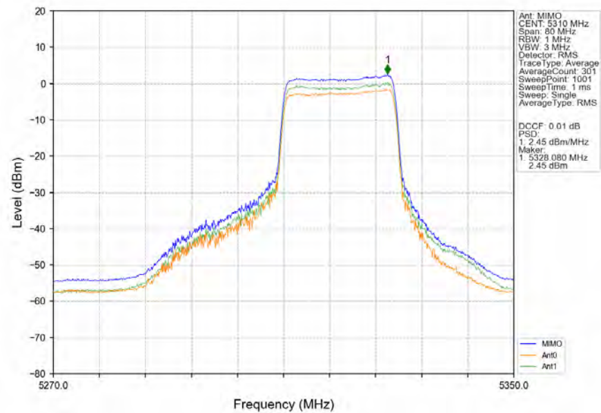
802.11be(EHT40) HCH 5310MHz RU242 Right MIMO NTN
