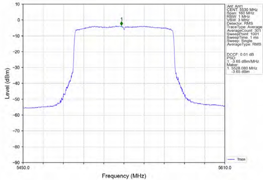
802.11be(EHT80) LCH_5530MHz_RU996_Left_MIMO_NTNV
