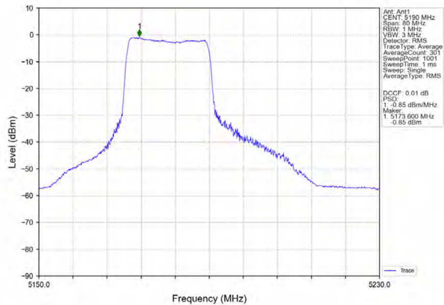
802.11be(EHT40) LCH_5190MHz_RU242_Left_Ant1_NTNV
