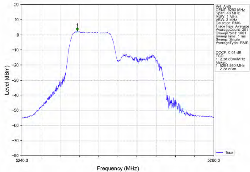
802.11be(EHT20) LCH_5260MHz_RU106_Left_Ant0_NTNV
