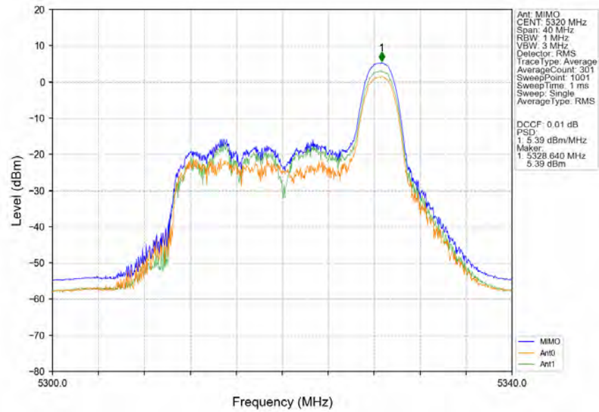
802.11be(EHT20)_HCH_5320MHz_RU26_Right_MIMO_NTNV
