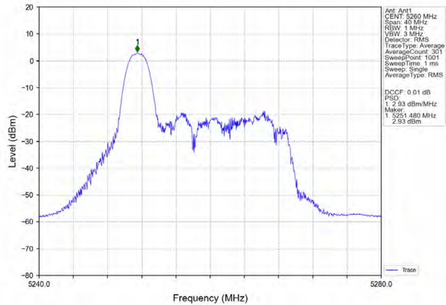
802.11be(EHT20) LCH_5260MHz_RU26_Left_MIMO_NTNV
