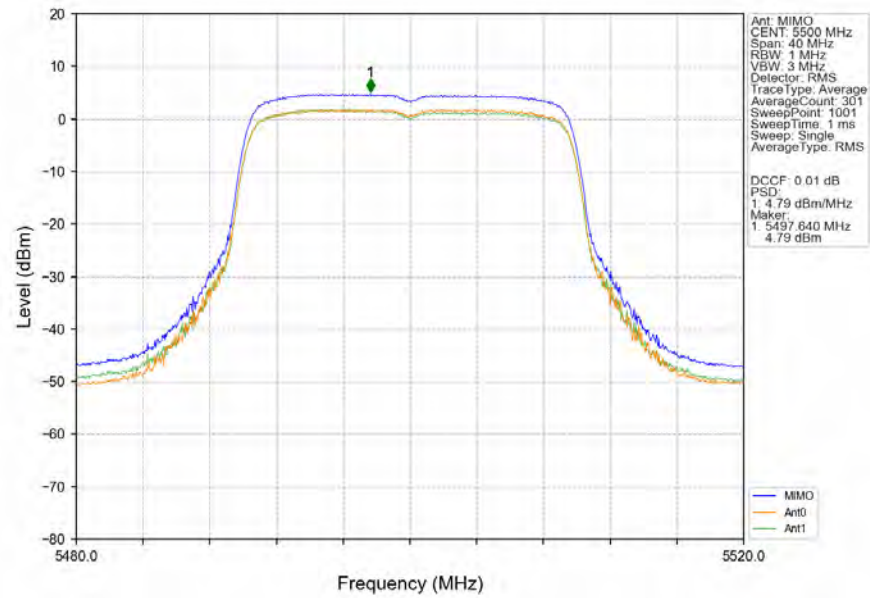
802.11be(EHT20) LCH_5500MHz_RU242_Left_MIMO_NTNV
