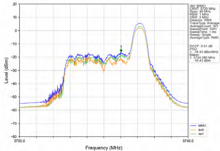
802.11be(EHT20)_HCH_5720MHz_RU26_Right_MIMO_NTNV
