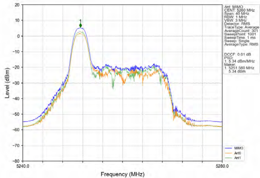
802.11be(EHT20) LCH_5260MHz_RU26_Left_MIMO_NTNV
