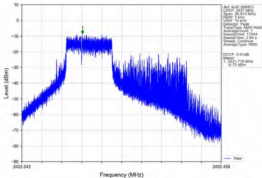
802.11be(EHT20)_MCH_2437MHz_26+52 / _Ant2 (MIMO) NTN
