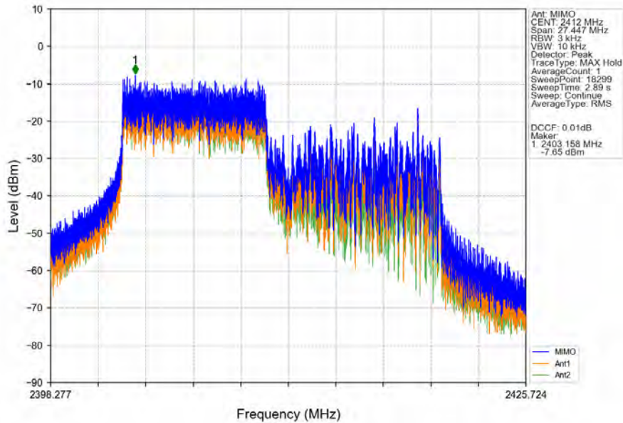
802.11be(EHT20)_LCH_2412MHz_RU242_Left_Ant2 (MIMO)_NTNV
