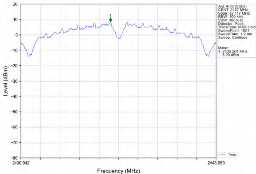
802.11b_MCH_2437MHz_Ant0 (SISO)_NTNV
