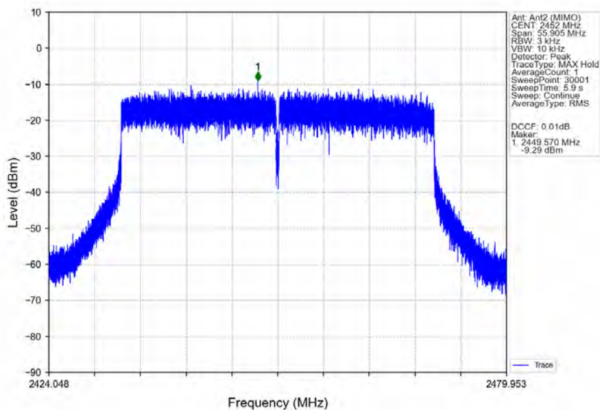
802.11ax(HEW40)_HCH_2452MHz_RU484_Left_Ant2 (MIMO)_NTNV
