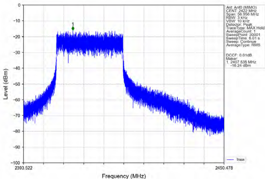
802.11be(EHT40)_LCH_2422MHz_RU242_Left_MIMO_NTNV
