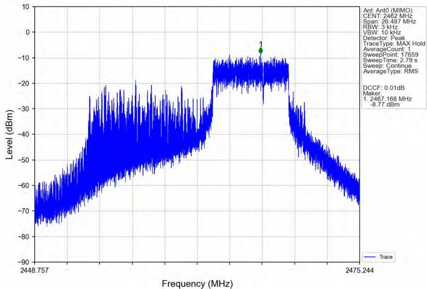
802.11be(EHT20)_HCH_2462MHz_26+52_/_Ant0 (MIMO)_NTNV
