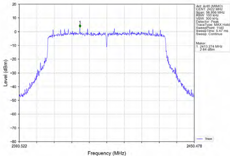
802.11be(EHT40)_LCH_2422MHz_RU484_Left_Ant0 (MIMO)_NTNV
