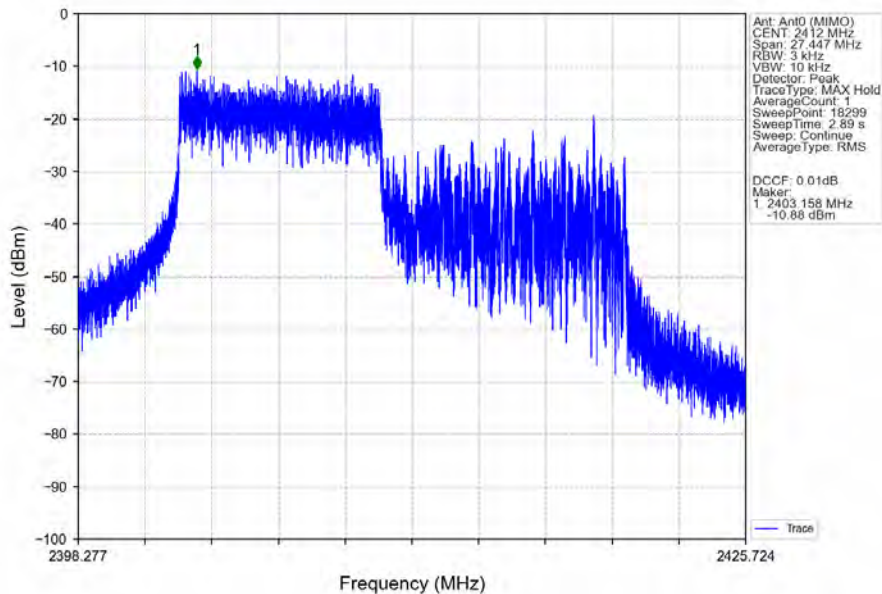
802.11be(EHT20)_LCH_2412MHz_RU106_Left_Ant0 (MIMO)_NTNV
