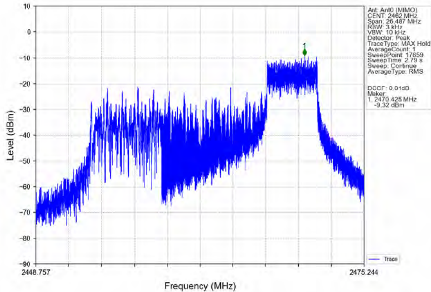
802.11be(EHT20)_HCH_2462MHz_RU52_Right_MIMO_NTNV
