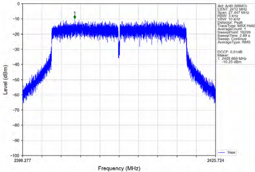
802.11be(EHT20)_LCH_2412MHz_RU242_Left_MIMO_NTNV
