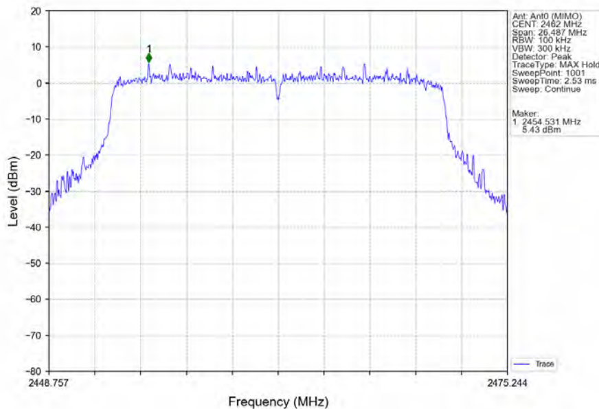
802.11be(EHT20)_HCH_2462MHz_RU242_Left_Ant0 (MIMO)_NTNV
