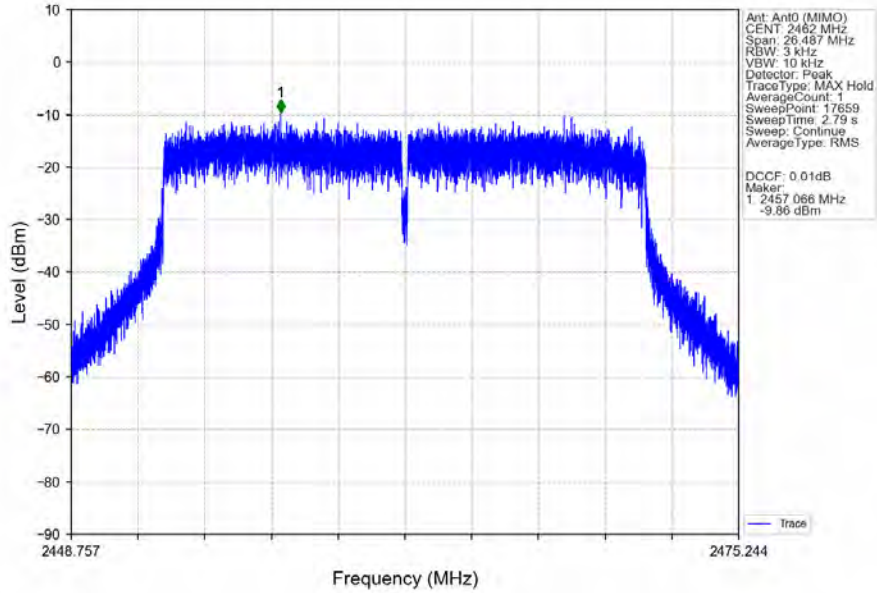
802.11be(EHT20)_HCH_2462MHz_RU242_Left_MIMO_NTNV
