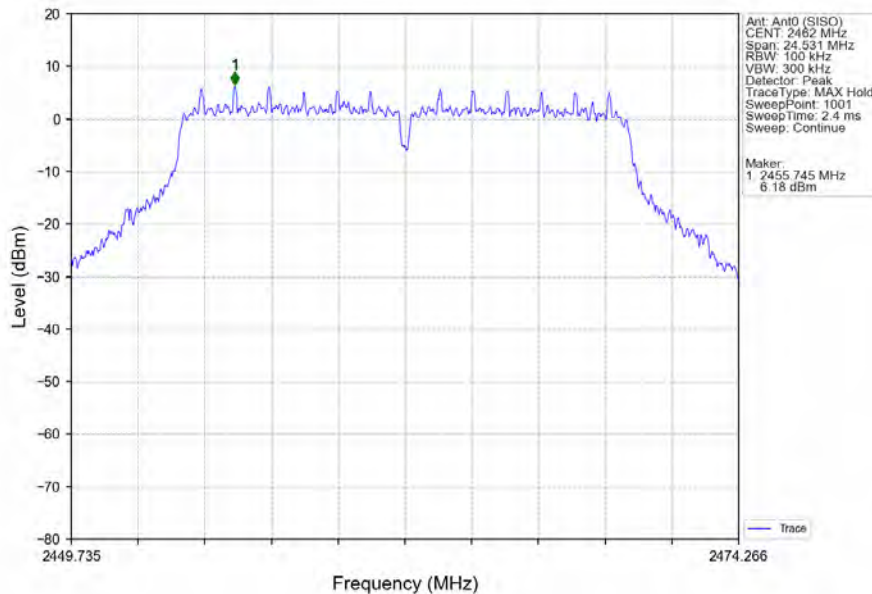
802.11g_HCH_2462MHz_Ant0 (SISO)_NTNV
