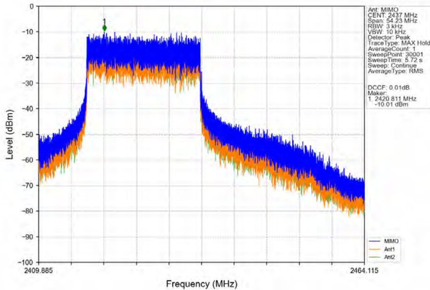
802.11be(EHT40)_MCH_2437MHz_RU484_Left_Ant2(MIMO)_NTNV
