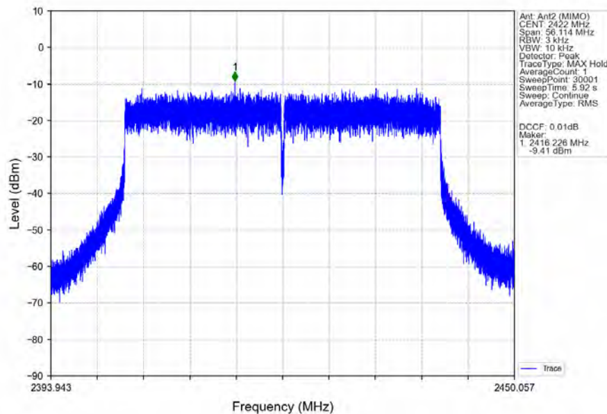
802.11ax(HEW40)_LCH_2422MHz_RU484_Left_Ant2(MIMO)_NTNV
