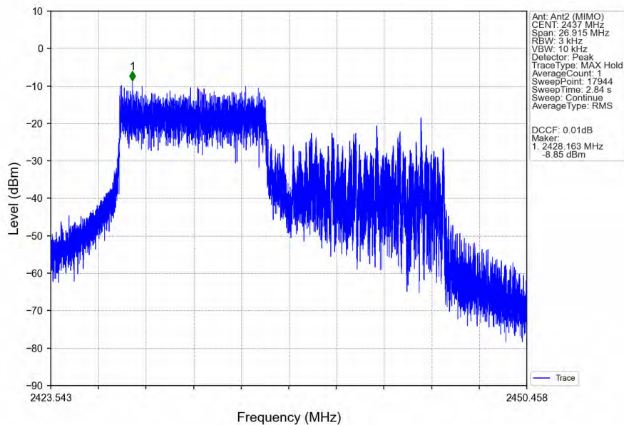
802.11be(EHT20)_MCH_2437MHz_RU106_Left_Ant2 (MIMO)_NTNV
