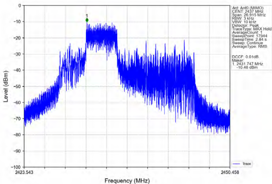
802.11be(EHT20)_MCH_2437MHz_RU52_Mid_Ant0 (MIMO)_NTNV
