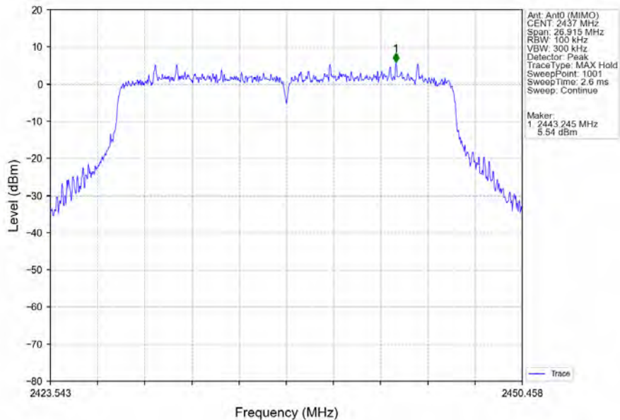
802.11be(EHT20)_MCH_2437MHz_RU242_Left_Ant0 (MIMO)_NTNV
