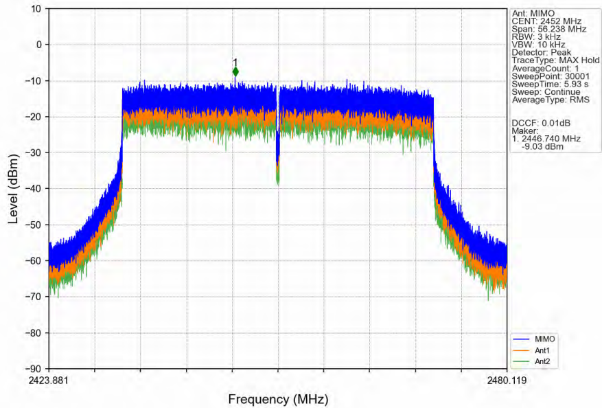
802.11be(EHT40)_HCH_2452MHz_26+106_/_Ant2 (MIMO)_NTNV
