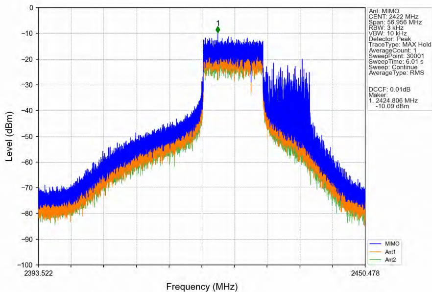
802.11be(EHT40)_LCH_2422MHz_26+106_/_MIMO_NTNV
