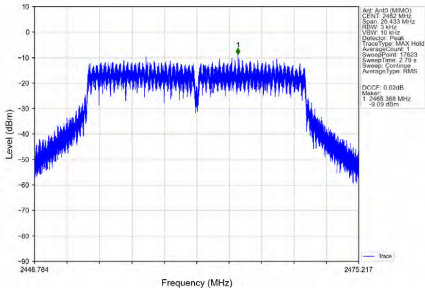
802.11n(HT20)_HCH_2462MHz_Ant0 (MIMO)_NTNV
