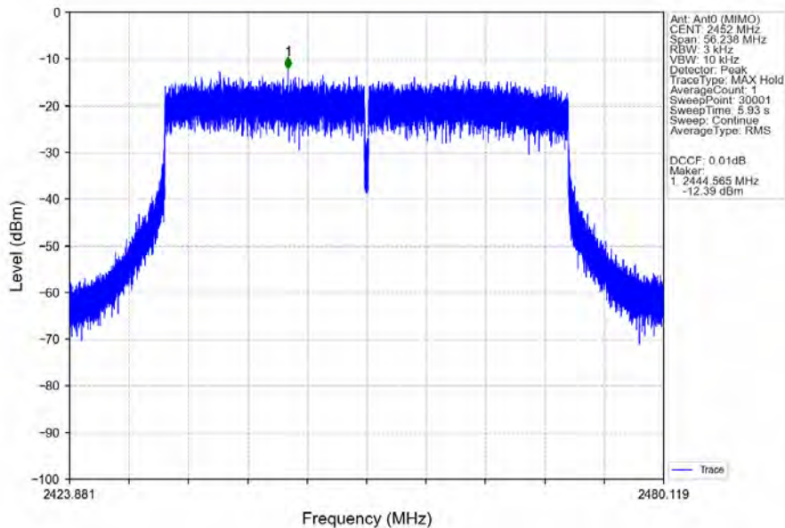
802.11be(EHT40)_HCH_2452MHz_RU484_Left_Ant0 (MIMO)_NTNV
