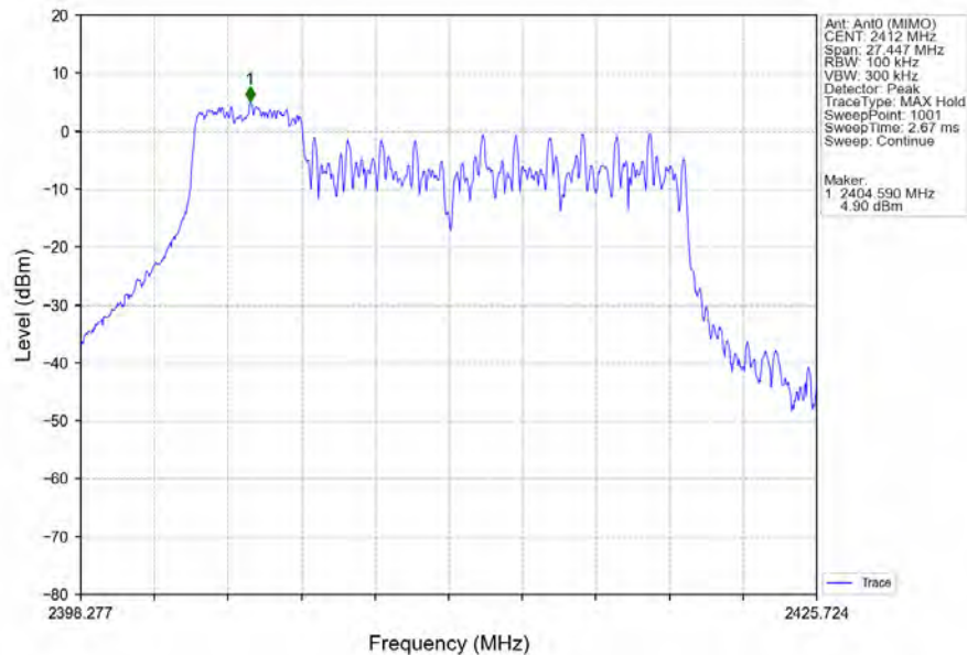
802.11be(EHT20)_LCH_2412MHz_RU52_Left_Ant0 (MIMO)_NTNV
