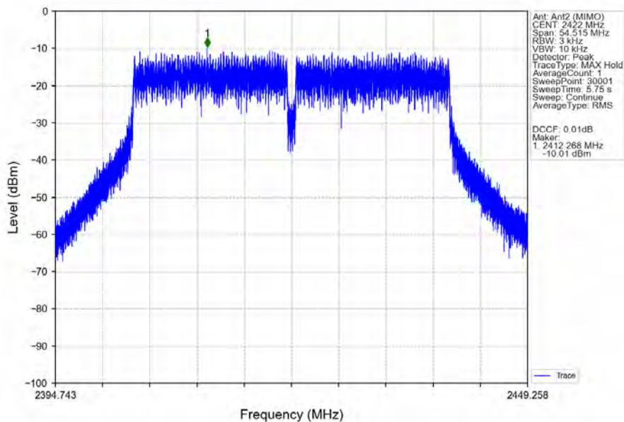
802.11n(HT40)_LCH_2422MHz_Ant2 (MIMO)_NTNV
