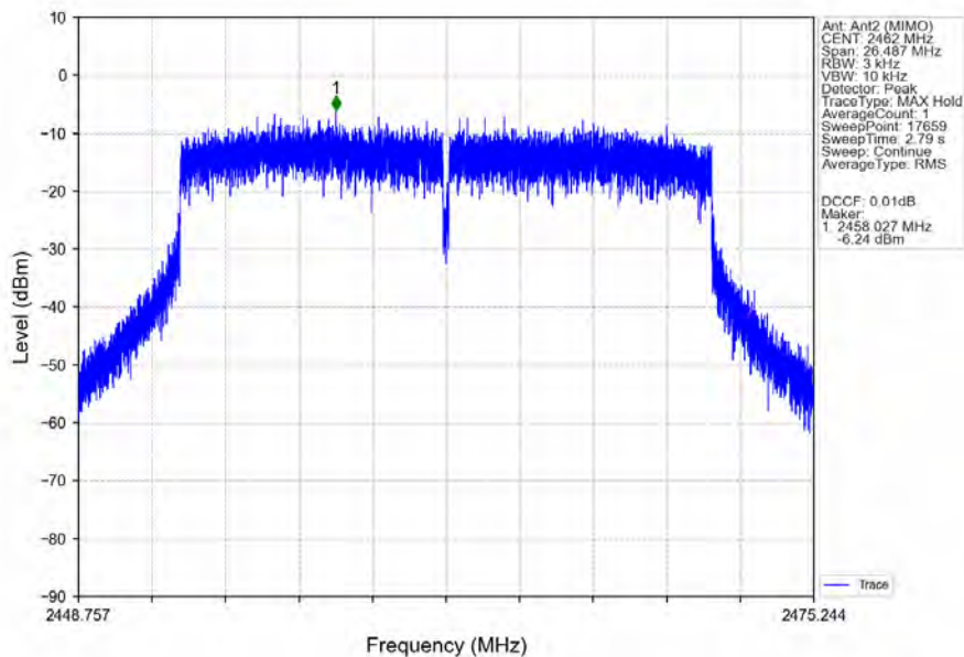
802.11be(EHT20)_HCH_2462MHz_RU242_Left_Ant2 (MIMO)_NTNV
