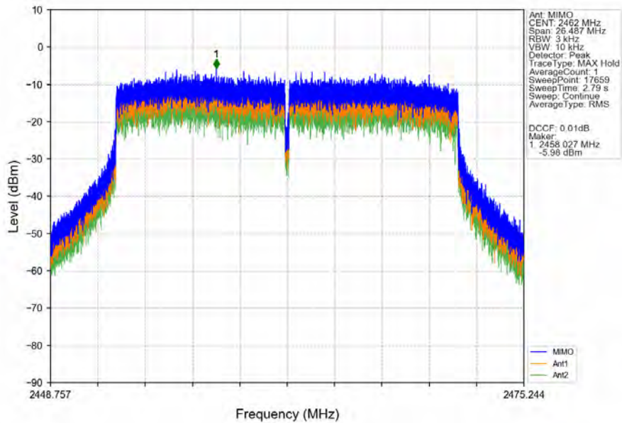
802.11be(EHT20)_HCH_2462MHz_RU242_Left_MIMO_NTNV
