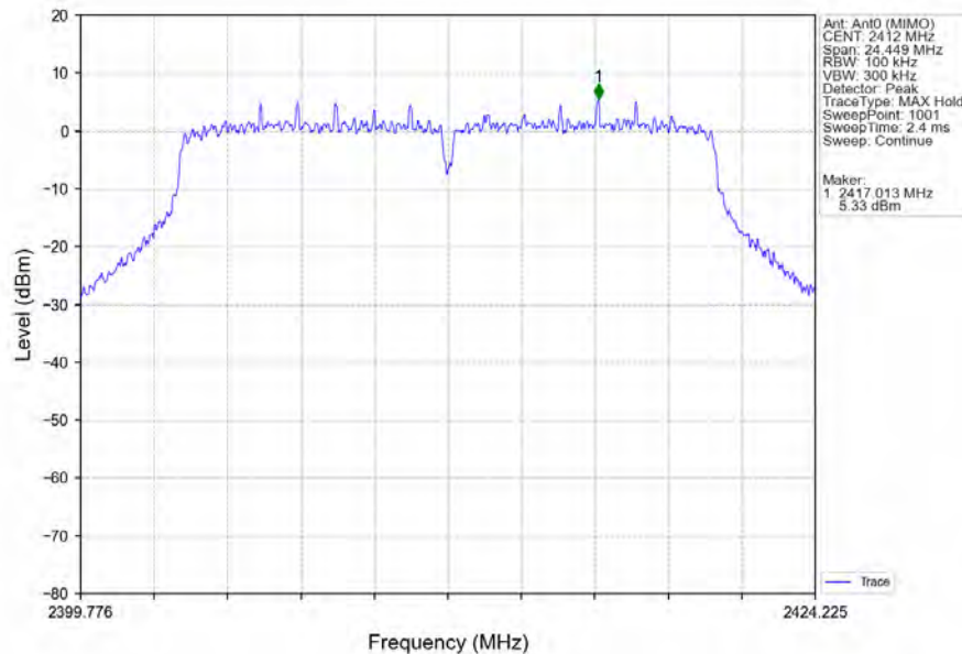
802.11n(HT20)_LCH_2412MHz_Ant0 (MIMO)_NTNV
