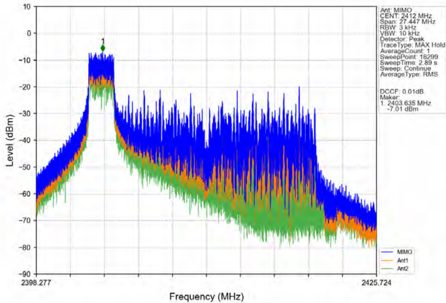
802.11be(EHT20)_LCH_2412MHz_RU52_Left_Ant2 (MIMO) NTN
