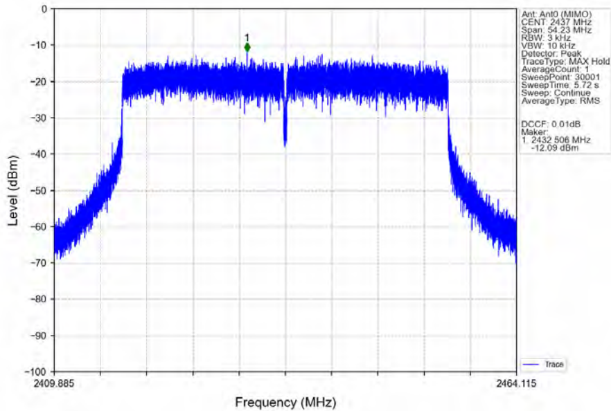
802.11be(EHT40)_MCH_2437MHz_RU484_Left_MIMO_NTNV
