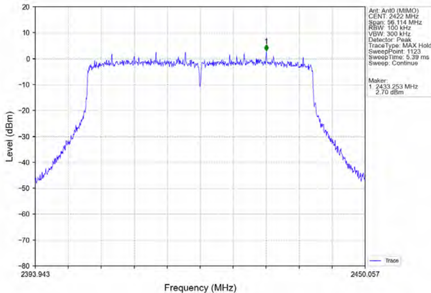
802.11ax(HEW40)_LCH_2422MHz_RU484_Left_Ant0 (MIMO)_NTNV
