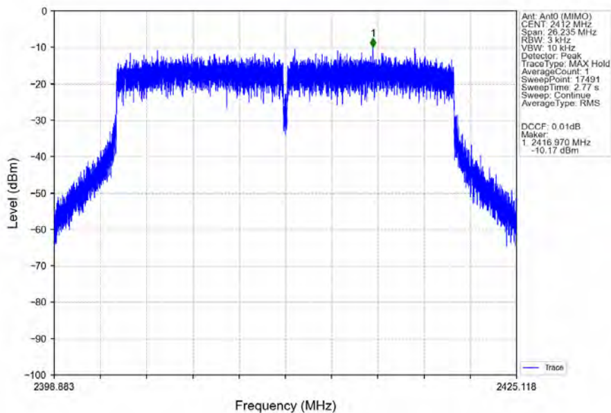
802.11ax(HEW20)_LCH_2412MHz_RU242_Left_Ant0 (MIMO)_NTNV
