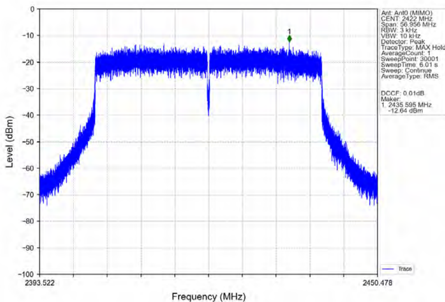
802.11be(EHT40)_LCH_2422MHz_RU484_Left_Ant0 (MIMO)_NTNV
