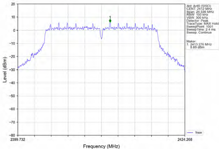
802.11g_LCH_2412MHz_Ant0 (SISO)_NTNV
