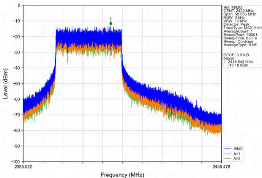
802.11be(EHT40)_LCH_2422MHz_RU242_Left_MIMO_NTNV
