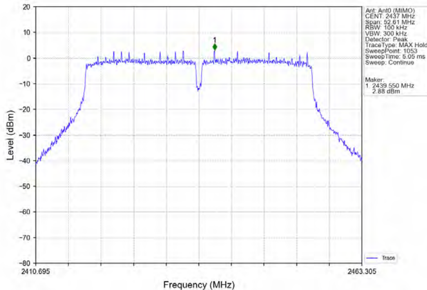
802.11n(HT40)_MCH_2437MHz_Ant0 (MIMO)_NTNV
