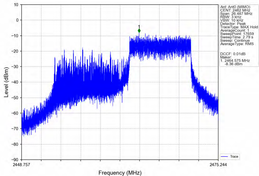
802.11be(EHT20)_HCH_2462MHz_RU106_Right_Ant0 (MIMO)_NTNV
