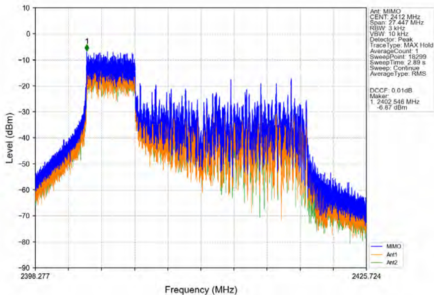
802.11be(EHT20)_LCH_2412MHz_RU52_Left MIMO_NTNV
