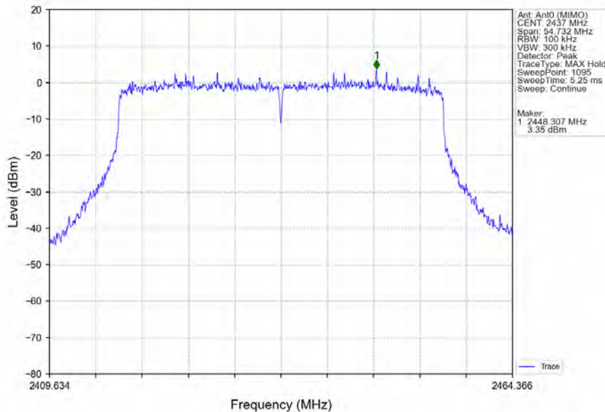
802.11ax(HEW40)_MCH_2437MHz_RU484_Left_Ant0 (MIMO)_NTNV
