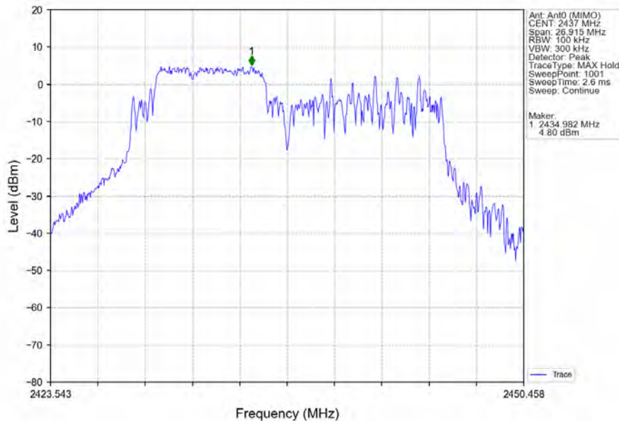
802.11be(EHT20)_MCH_2437MHz_26+52_/_Ant0 (MIMO)_NTNV
