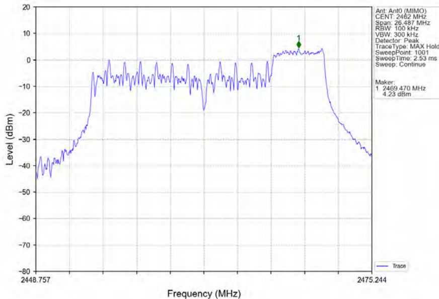
802.11be(EHT20)_HCH_2462MHz_RU52_Right_Ant0 (MIMO)_NTNV
