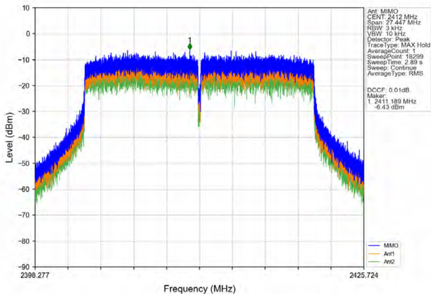
802.11be(EHT20)_LCH_2412MHz_RU242_Left_MIMO_NTNV
