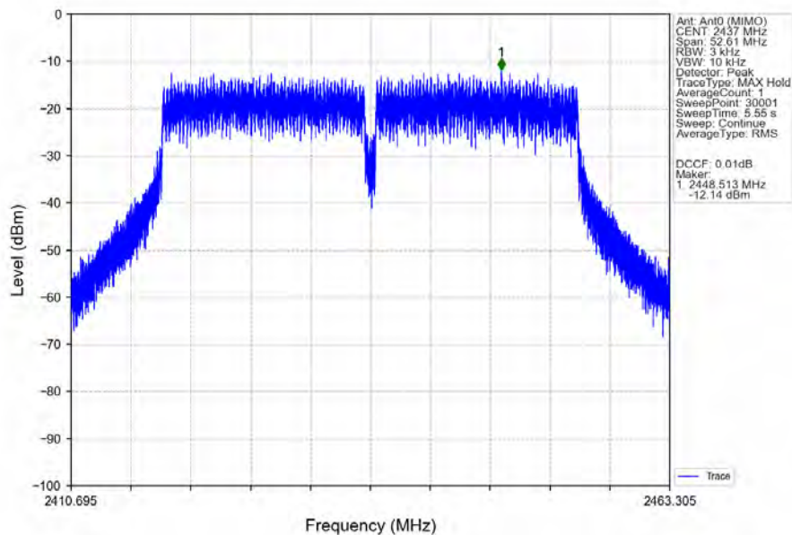
802.11n(HT40)_MCH_2437MHz_Ant0 (MIMO)_NTNV
