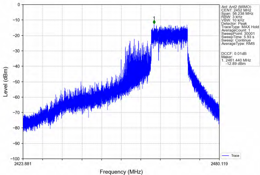
802.11be(EHT40)_HCH_2452MHz_26+106_/_Ant2 (MIMO)_NTNV
