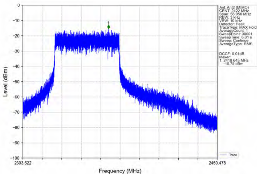
802.11be(EHT40)_LCH_2422MHz_RU242_Left_Ant2 (MIMO)_NTNV
