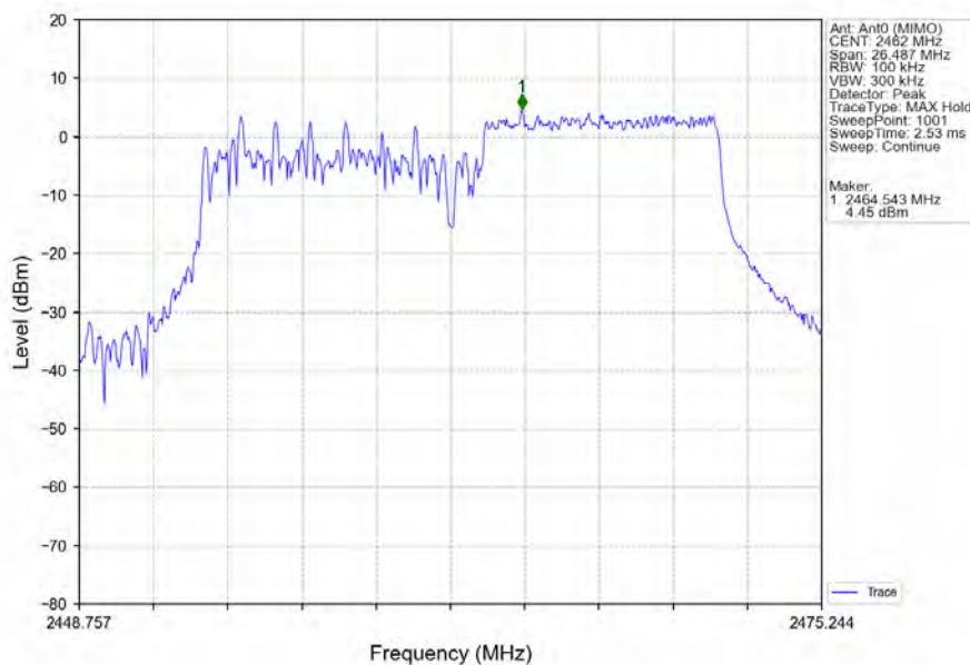
802.11be(EHT20)_HCH_2462MHz_RU106_Right_Ant0 (MIMO)_NTNV
