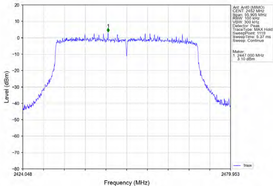
802.11ax(HEW40)_HCH_2452MHz_RU484_Left_Ant0 (MIMO)_NTNV
