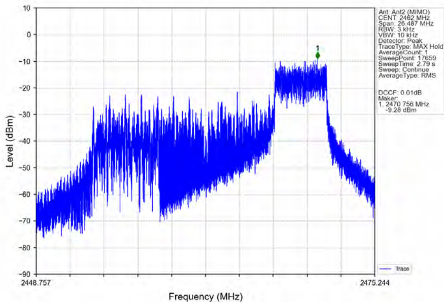
802.11be(EHT20)_HCH_2462MHz_RU52_Right_Ant2 (MIMO)_NTNV
