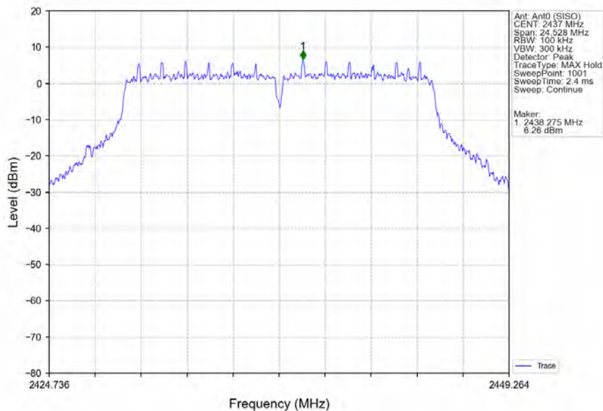
802.11g_MCH_2437MHz_Ant0 (SISO)_NTNV
