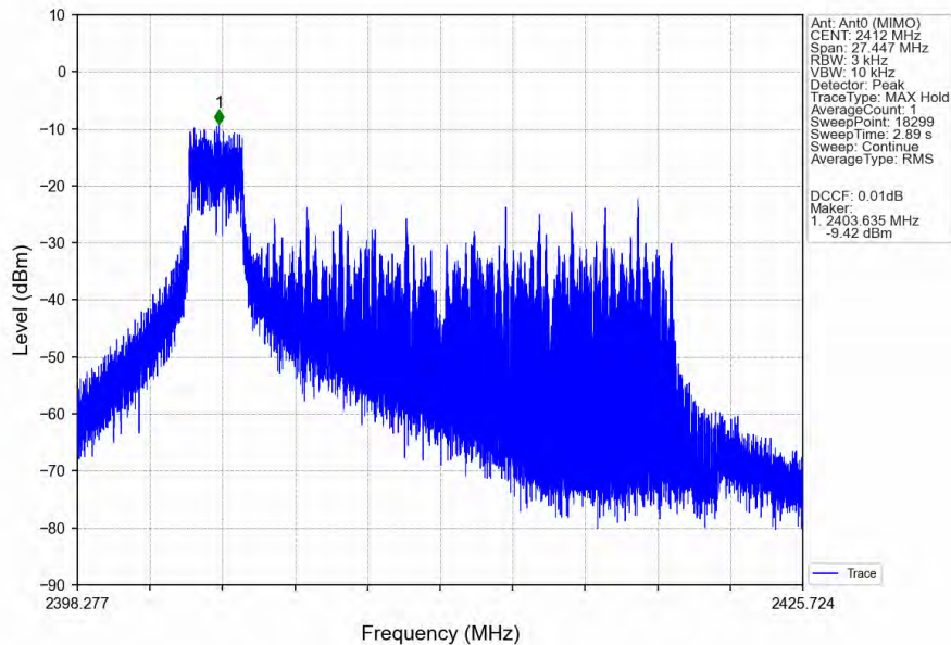
802.11be(EHT20)_LCH_2412MHz_RU26_Left_Ant0 (MIMO)_NTNV
