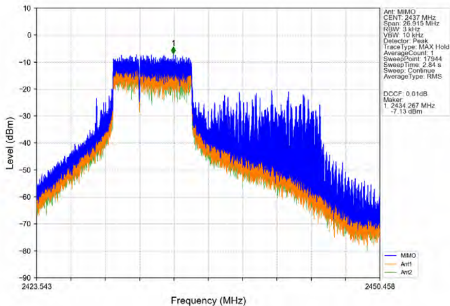
802.11be(EHT20)_MCH_2437MHz_26+52_/_MIMO_NTNV
