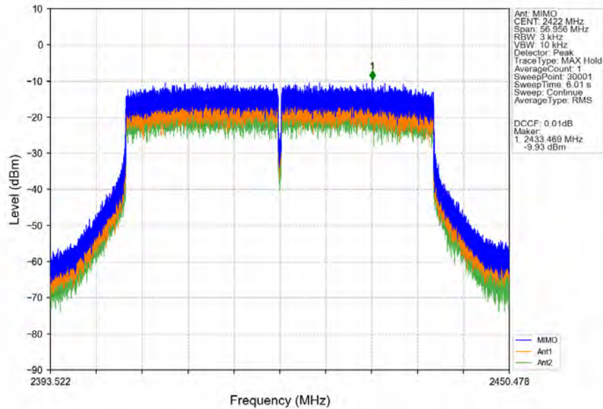
802.11be(EHT40)_LCH_2422MHz_26+106 / _Ant2 (MIMO) NTN
