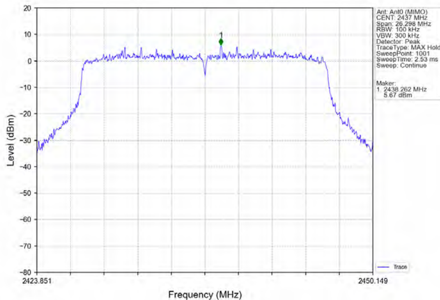
802.11ax(HEW20)_MCH_2437MHz_RU242_Left_Ant0 (MIMO)_NTNV
