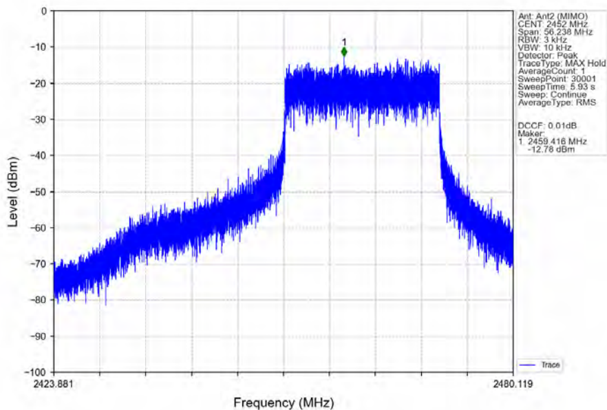
802.11be(EHT40)_HCH_2452MHz_RU242_Right_Ant2 (MIMO)_NTNV
