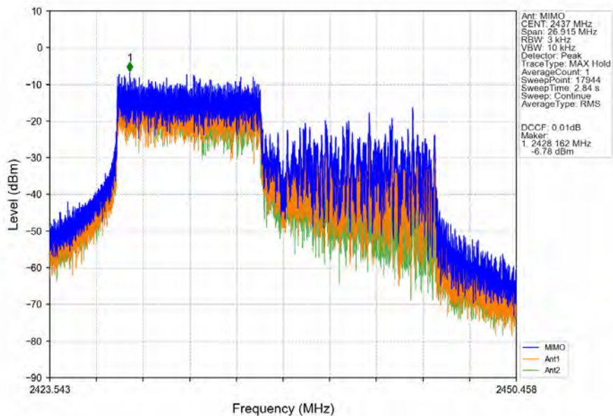
802.11be(EHT20)_MCH_2437MHz_RU106_Left_MIMO_NTNV
