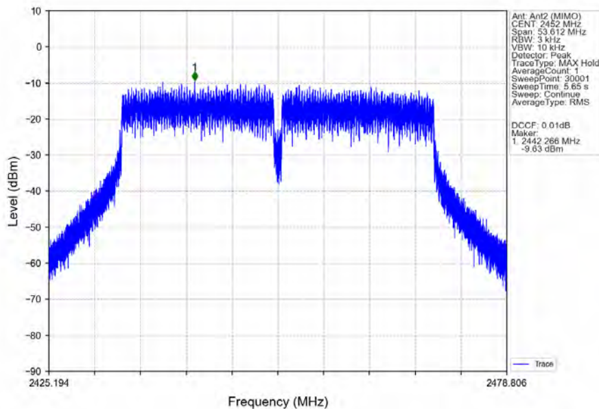
802.11n(HT40)_HCH_2452MHz_Ant2 (MIMO)_NTNV
