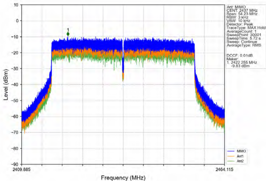
802.11be(EHT40)_MCH_2437MHz_RU484_Left_MIMO_NTNV
