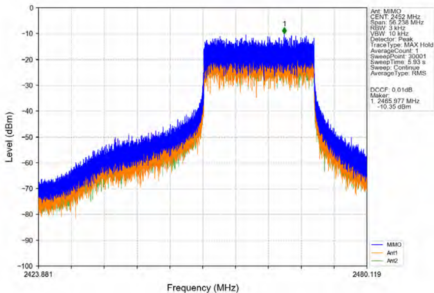
802.11be(EHT40)_HCH_2452MHz_RU242_Right MIMO_NTNV
