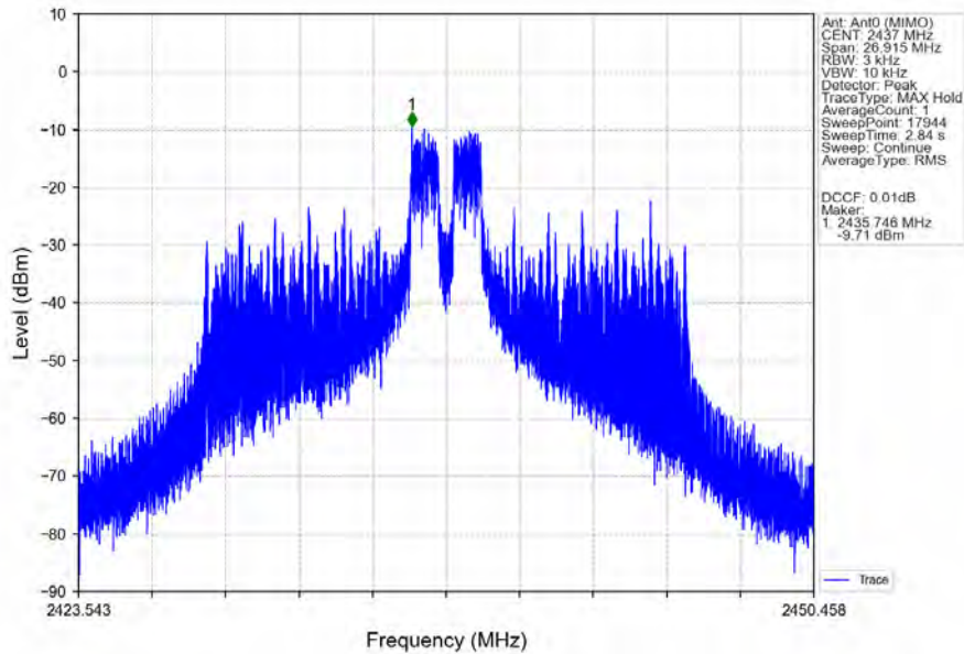
802.11be(EHT20)_MCH_2437MHz_RU26_Mid_MIMO_NTNV
