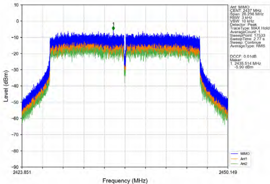
802.11ax(HEW20)_MCH_2437MHz_RU242_Left_MIMO_NTNV
