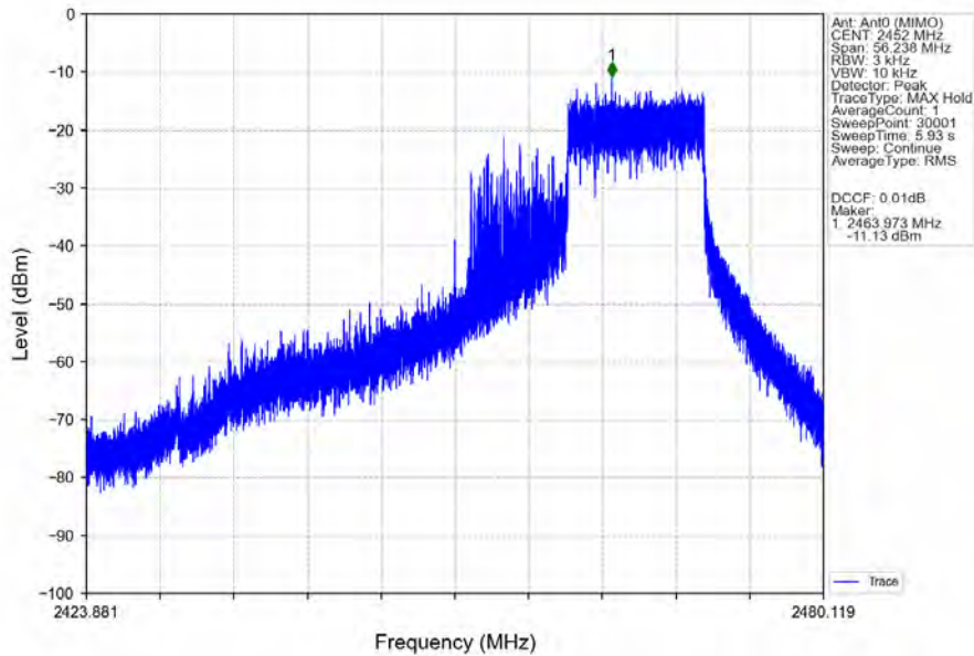
802.11be(EHT40)_HCH_2452MHz_26+106_/_MIMO_NTNV
