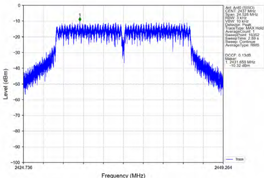
802.11g_MCH_2437MHz_Ant0 (SISO)_NTNV
