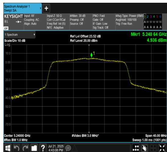
11AX20MIMO-Ant10-5260-PASS
