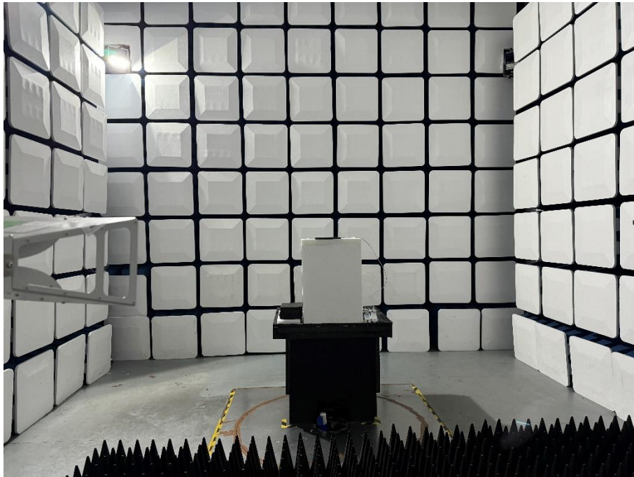
Above 1GHz-BT/WIFI
