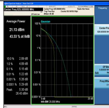
Band26(824-849)-3MHz-QPSK-26805-15RB#0-PASS
