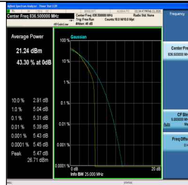
Band26(824-849)-3MHz-QPSK-26915-15RB#0-PASS
