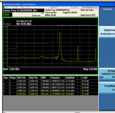
Band38-20MHz-QPSK-37850-1RB#0-PASS
