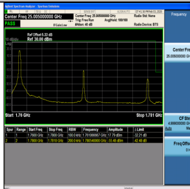
Band66-20MHz-QPSK-132572-1RB#99-PASS
