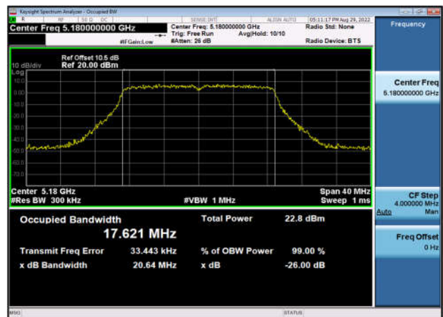
U-NII-1 99% OBW & 26dB EBW-802.11ac(20MHz) ,5180MHz,Ant1
