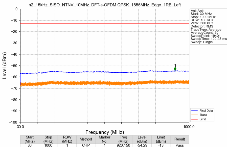
n2_15kHz_SISO_NTNV_10MHz_DFT-s-OFDM QPSK_1855MHz_Edge_1RB_Left
