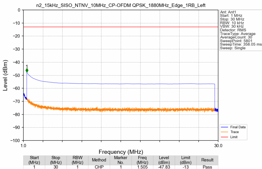
n2_15kHz_SISO_NTNV_10MHz_CP-OFDM QPSK_1880MHz_Edge_1RB_Left
