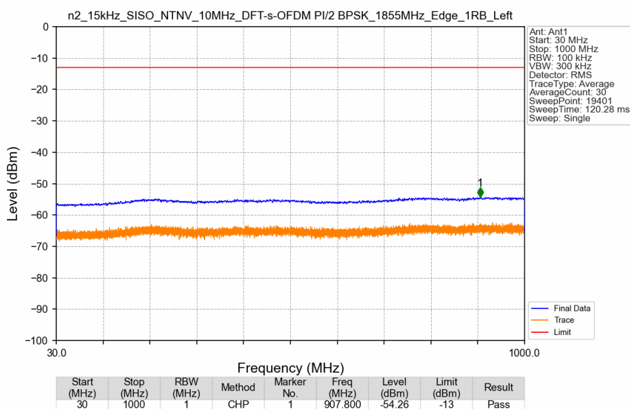
n2_15kHz_SISO_NTNV_10MHz_DFT-s-OFDM PI/2 BPSK_1855MHz_Edge_1RB_Left
