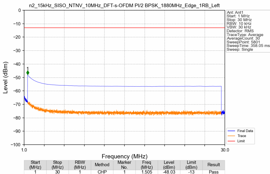
n2_15kHz_SISO_NTNV_10MHz_DFT-s-OFDM PI/2 BPSK_1880MHz_Edge_1RB_Left
