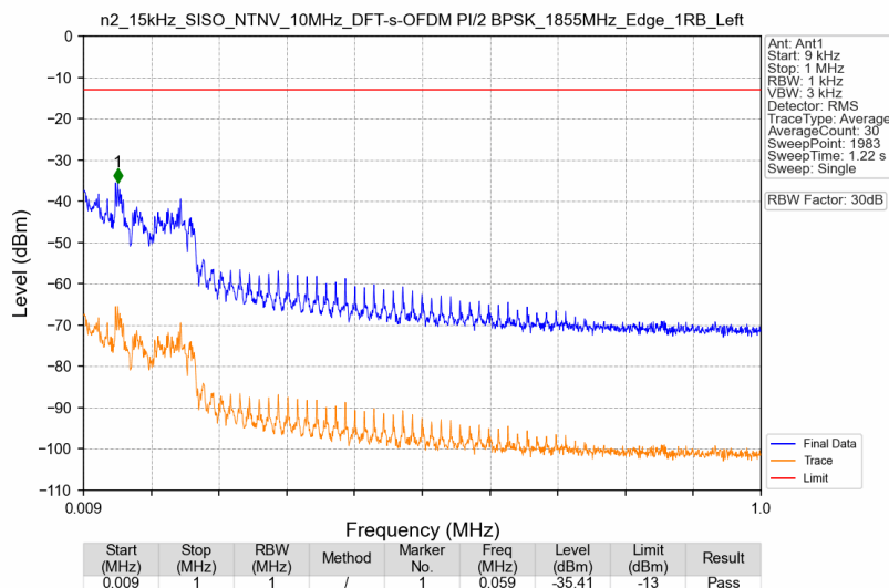
n2_15kHz_SISO_NTNV_10MHz_DFT-s-OFDM PI/2 BPSK_1855MHz_Edge_1RB_Left
