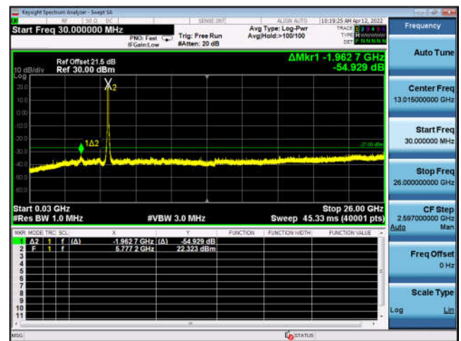
U-NII-3 ,802.11ax-HE80, 5775MHz, Ant4
