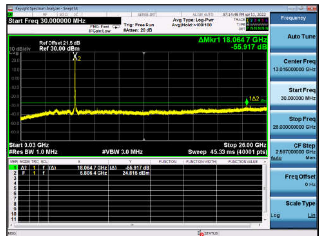
U-NII-3 ,802.11ax-HE40, 5795MHz, Ant3
