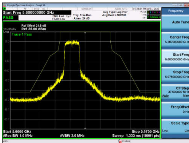
U-NII-3 ,802.11ax-HE40, 5795MHz, Ant3
