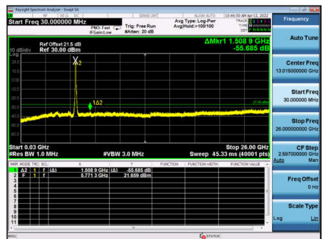
U-NII-3 ,802.11ax-HE80, 5775MHz, Ant5
