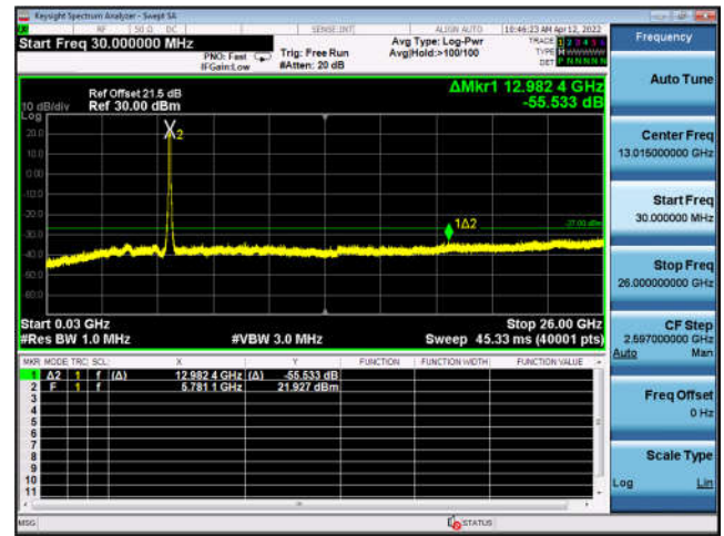
U-NII-3 ,802.11ax-HE80, 5775MHz, Ant5
