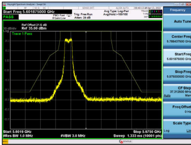
U-NII-3 ,802.11ax-HE20, 5785MHz, Ant5
