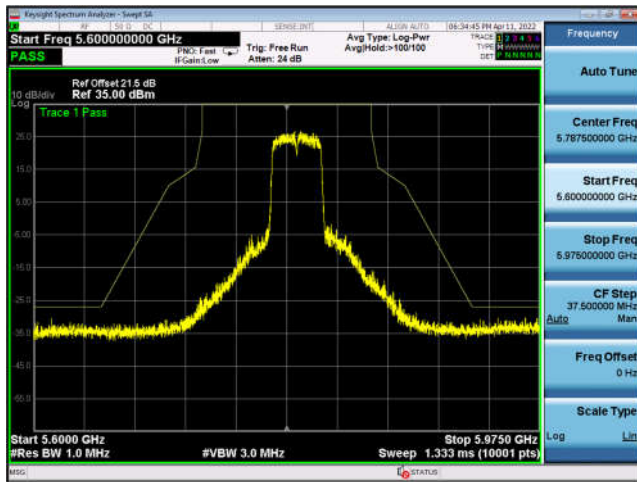
U-NII-3 ,802.11ax-HE40, 5755MHz, Ant3
