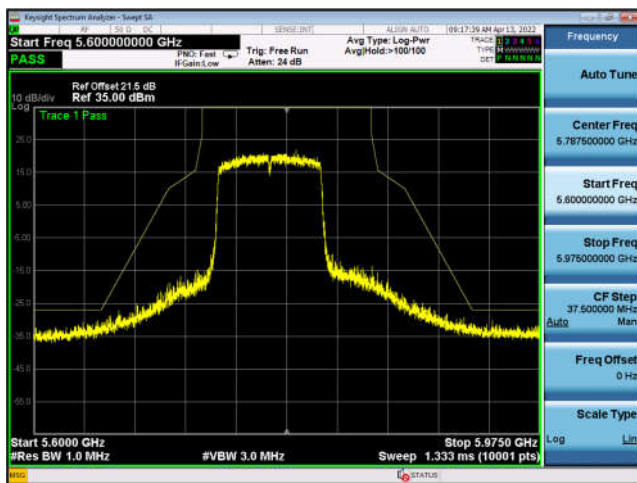
U-NII-3 ,802.11ax-HE80, 5775MHz, Ant4
