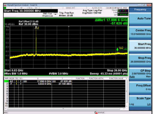
U-NII-3 ,802.11ax-HE20, 5825MHz, Ant5
