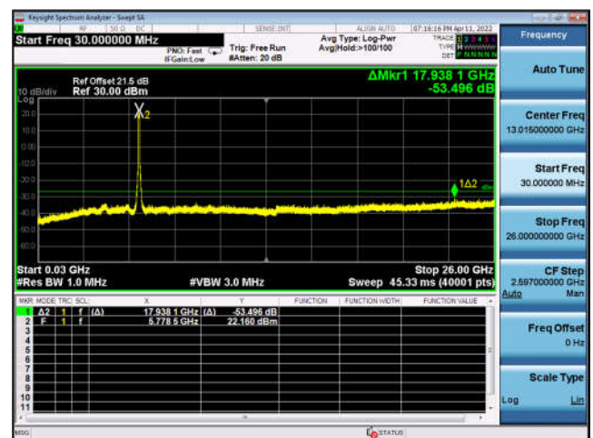
U-NII-3 ,802.11ax-HE80, 5775MHz, Ant3
