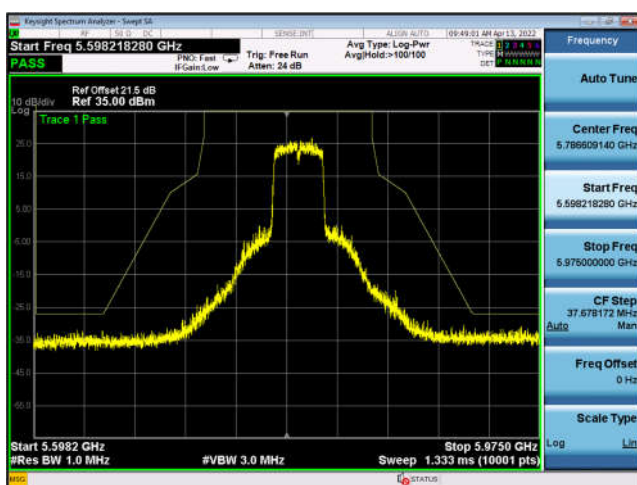
U-NII-3 ,802.11ax-HE40, 5795MHz, Ant5
