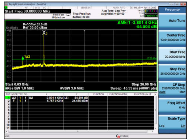
U-NII-3 ,802.11ax-HE40, 5755MHz, Ant3
