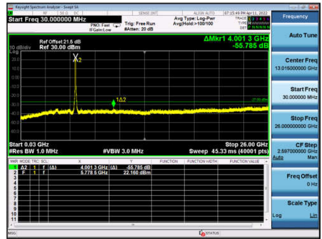
U-NII-3 ,802.11ax-HE80, 5775MHz, Ant3
