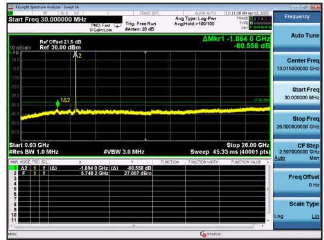
U-NII-3 ,802.11ax-HE20, 5785MHz, Ant4
