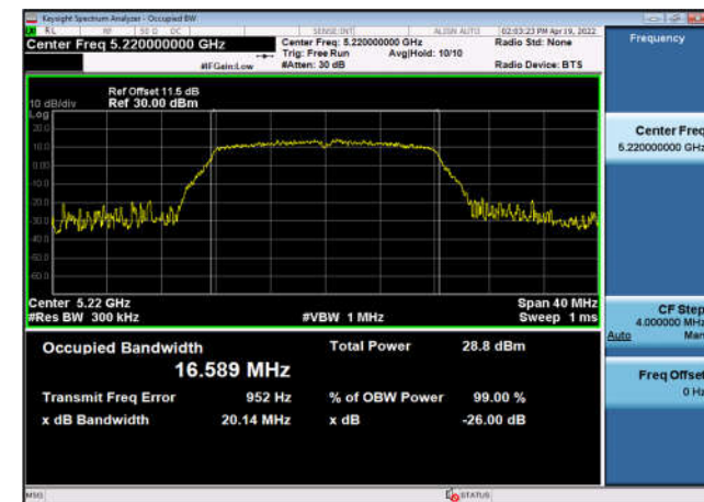
U-NII-1 99% OBW & 26 EBW-802.11a(20MHz) ,5220MHz,Ant5
