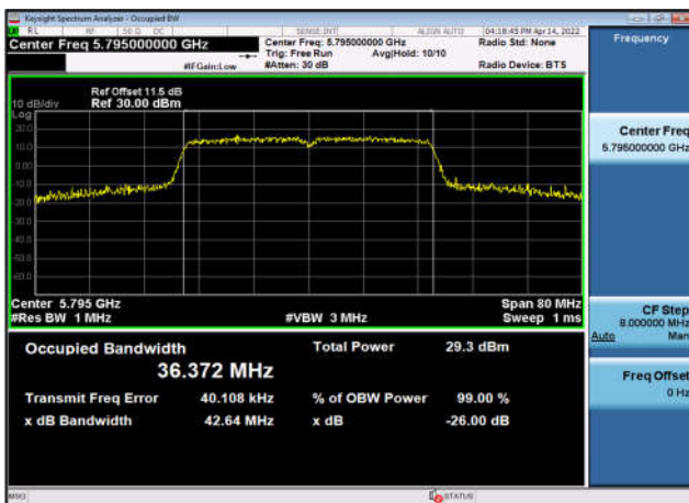
U-NII-3 99% OBW & 26 EBW-802.11ac(40MHz) ,5795MHz,Ant2
