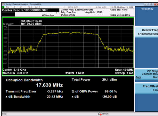
U-NII-1 99% OBW & 26 EBW-802.11ax(20MHz) ,5180MHz,Ant4
