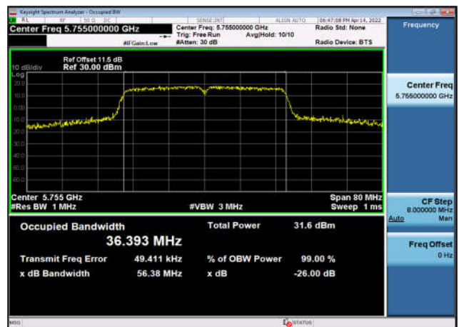
U-NII-3 99% OBW & 26 EBW-802.11ax(40MHz) ,5755MHz,Ant3
