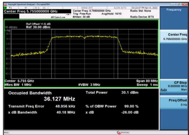
U-NII-3 99% OBW & 26 EBW-802.11ax(40MHz) ,5755MHz,Ant0
