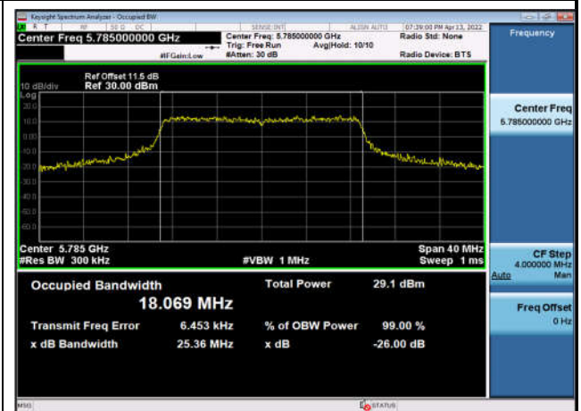
U-NII-3 99% OBW & 26 EBW-802.11ac(20MHz) ,5785MHz,Ant4
