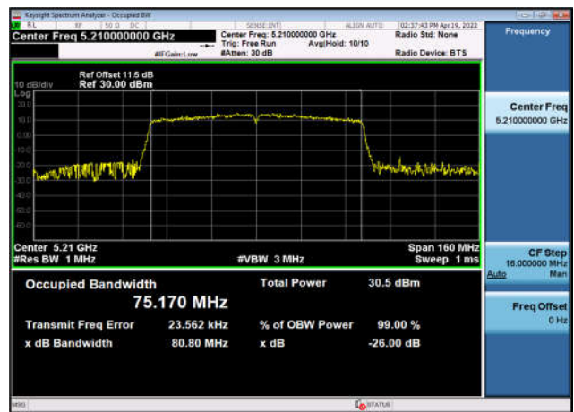
U-NII-1 99% OBW & 26 EBW-802.11ac(80MHz) ,5210MHz,Ant5
