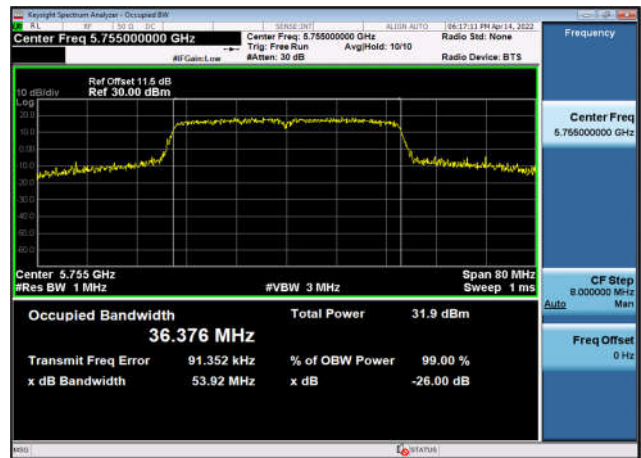
U-NII-3 99% OBW & 26 EBW-802.11ac(40MHz) ,5755MHz,Ant3
