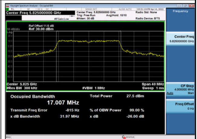
U-NII-3 99% OBW & 26 EBW-802.11a(20MHz) ,5825MHz,Ant2
