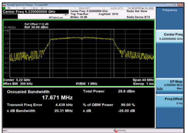
U-NII-1 99% OBW & 26 EBW-802.11n(20MHz) ,5220MHz,Ant5
