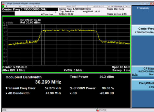
U-NII-3 99% OBW & 26 EBW-802.11n(40MHz) ,5795MHz,Ant0
