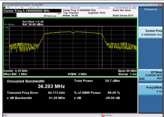
U-NII-1 99% OBW & 26 EBW-802.11n(40MHz) ,5190MHz,Ant4
