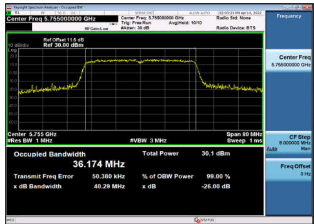
U-NII-3 99% OBW & 26 EBW-802.11ac(40MHz) ,5755MHz,Ant0
