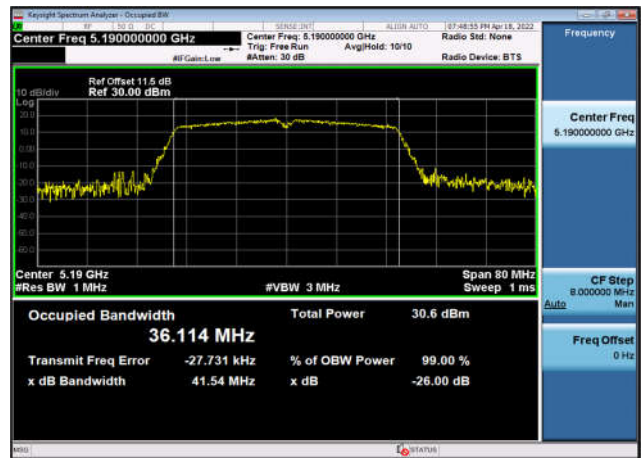
U-NII-1 99% OBW & 26 EBW-802.11ac(40MHz) ,5190MHz,Ant3
