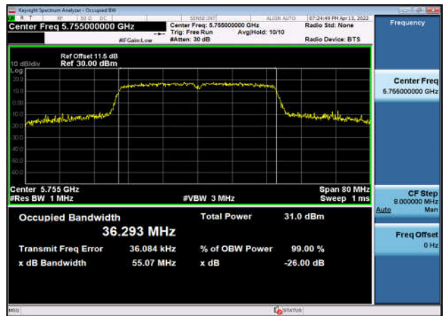
U-NII-3 99% OBW & 26 EBW-802.11n(40MHz) ,5755MHz,Ant4
