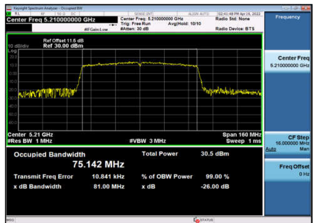
U-NII-1 99% OBW & 26 EBW-802.11ax(80MHz) ,5210MHz,Ant5
