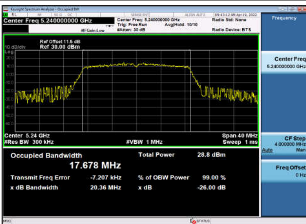
U-NII-1 99% OBW & 26 EBW-802.11n(20MHz) ,5240MHz,Ant4
