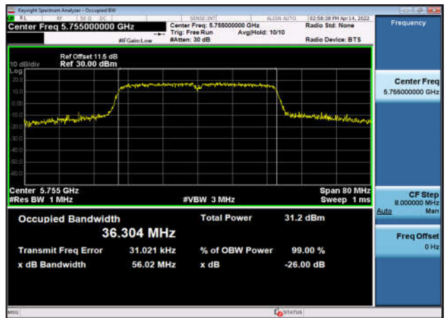
U-NII-3 99% OBW & 26 EBW-802.11n(40MHz) ,5755MHz,Ant1
