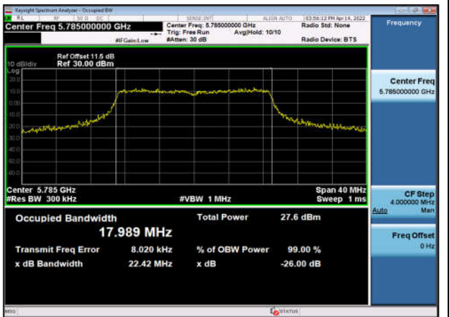
U-NII-3 99% OBW & 26 EBW-802.11n(20MHz) ,5785MHz,Ant2
