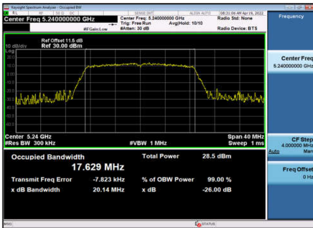
U-NII-1 99% OBW & 26 EBW-802.11ac(20MHz) ,5240MHz,Ant3
