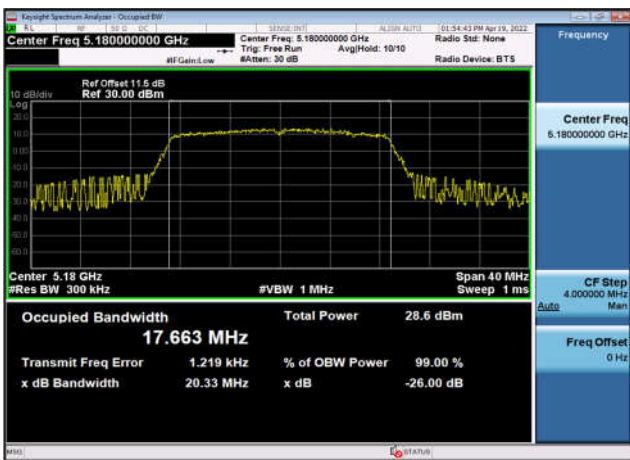
U-NII-1 99% OBW & 26 EBW-802.11n(20MHz) ,5180MHz,Ant5
