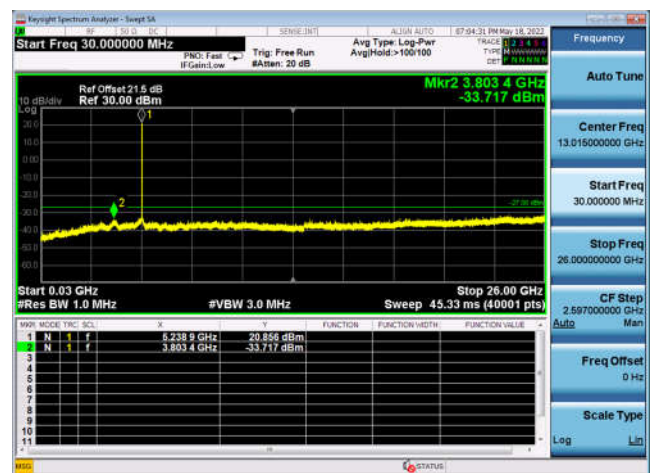
U-NII-1 ,802.11ax-HE20, 5240MHz, Ant5
