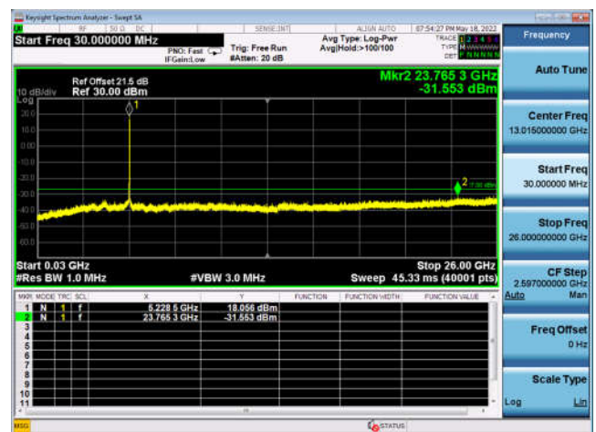
U-NII-1 ,802.11ax-HE40, 5230MHz, Ant4
