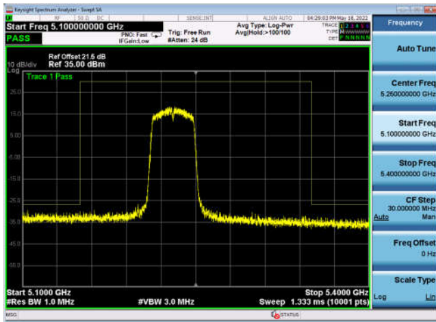
U-NII-1 ,802.11ax-HE40, 5190MHz, Ant4
