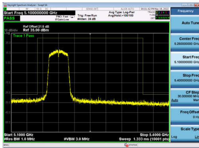
U-NII-1 ,802.11ax-HE40, 5230MHz, Ant5
