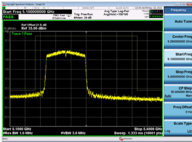
U-NII-1 ,802.11ax-HE80, 5210MHz, Ant4
