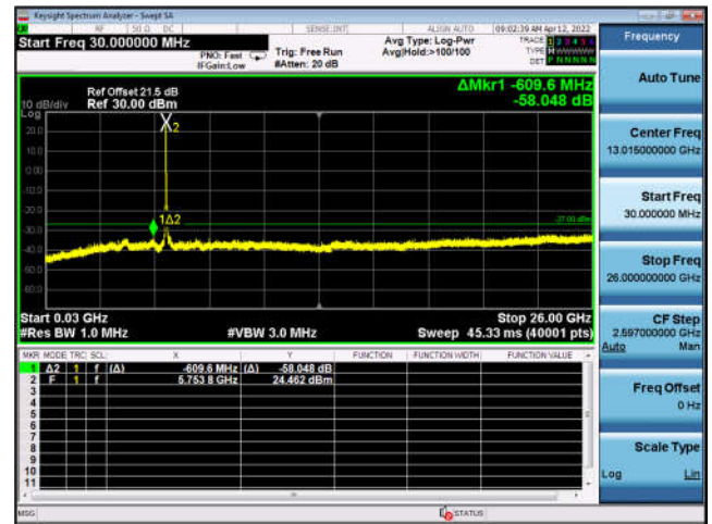
U-NII-3 ,802.11n-HT40, 5795MHz, Ant0
