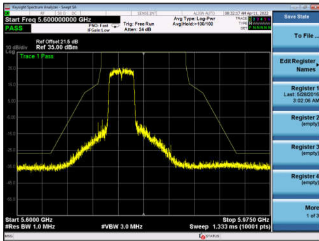
U-NII-3 ,802.11n-HT40, 5795MHz, Ant0
