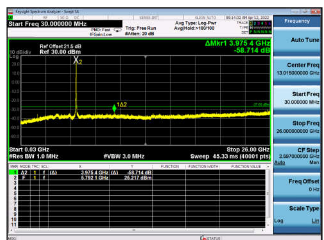
U-NII-3 ,802.11ax-HE40, 5795MHz, Ant0
