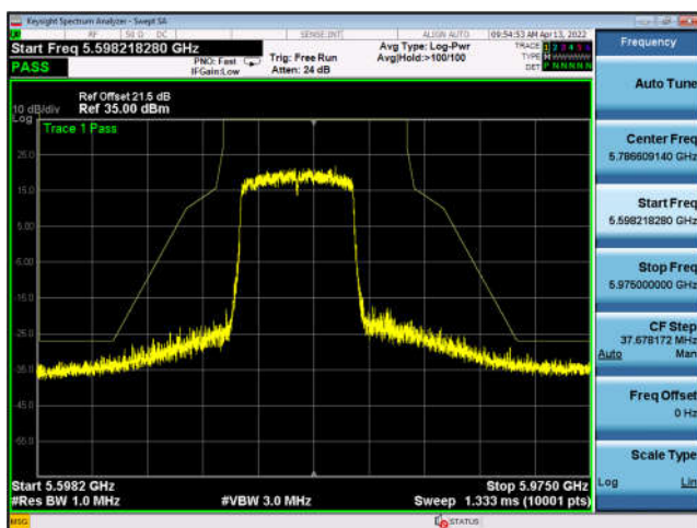
U-NII-3 ,802.11ax-HE80, 5775MHz, Ant0
