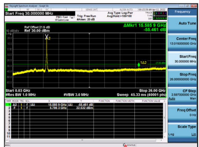
U-NII-3 ,802.11ax-HE80, 5775MHz, Ant0
