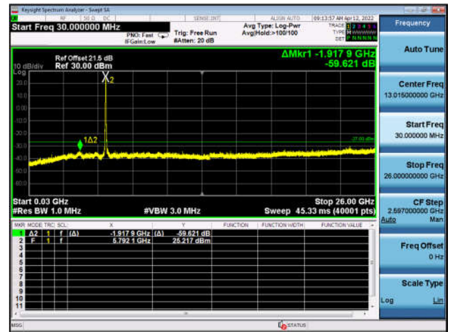
U-NII-3 ,802.11ax-HE40, 5755MHz, Ant0
