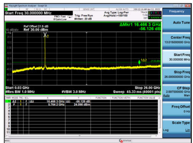
U-NII-3 ,802.11ac-VHT40, 5755MHz, Ant0
