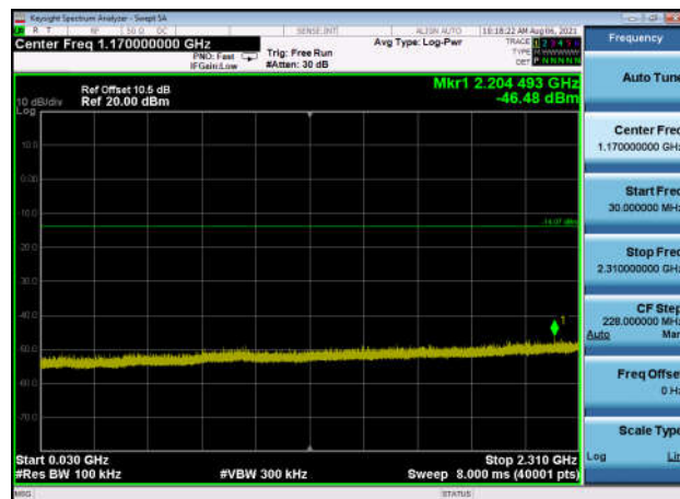
,Plot 3,30MHz~2310MHz-802.11g,2437MHz
