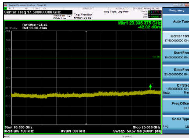
,Plot 5,10000MHz~25000MHz-802.11b ,2437MHz,Ant1
