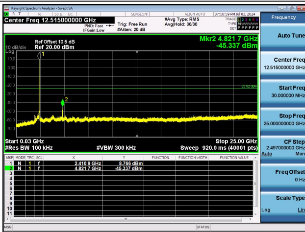
11G-Ant0-2412-30~25000-PASS
