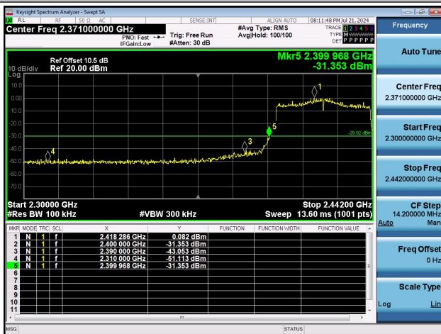
11AX40MIMO-Ant0-2422-PASS
