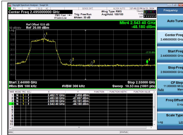
11AX20MIMO-Ant0-2462-PASS
