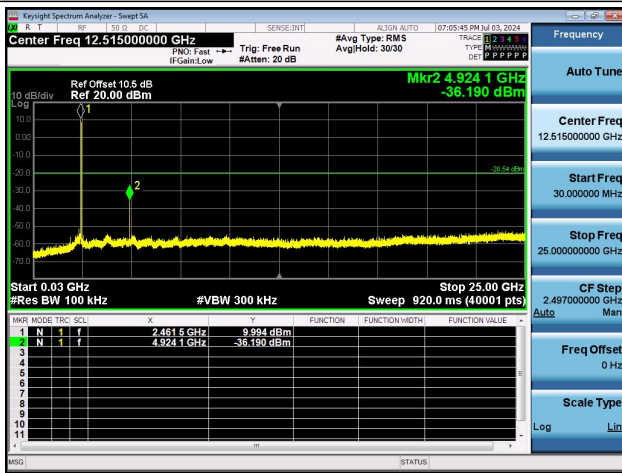
11B-Ant0-2462-30~25000-PASS
