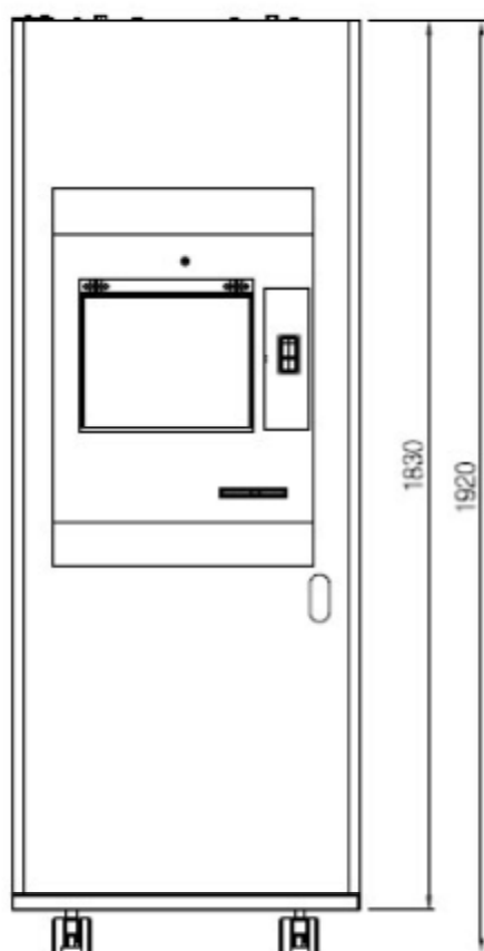
HDM600 DIMENSION
