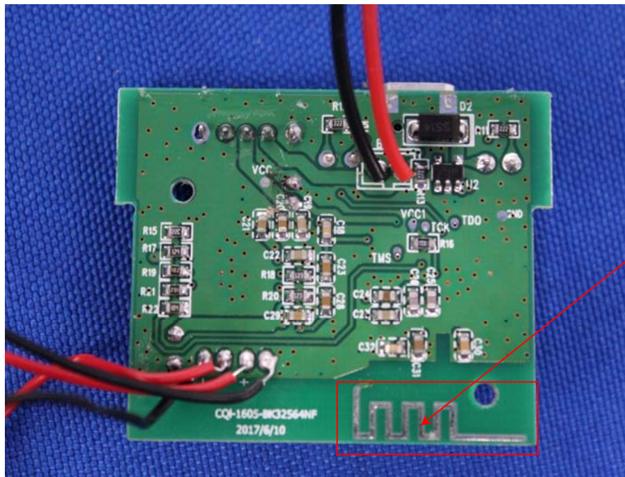
Antenna
