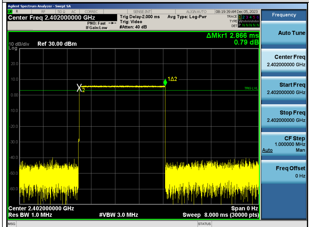
Test_Graph_GFSK_HOP_ANT1_NA_1Mbps_2402_Time per Burst
