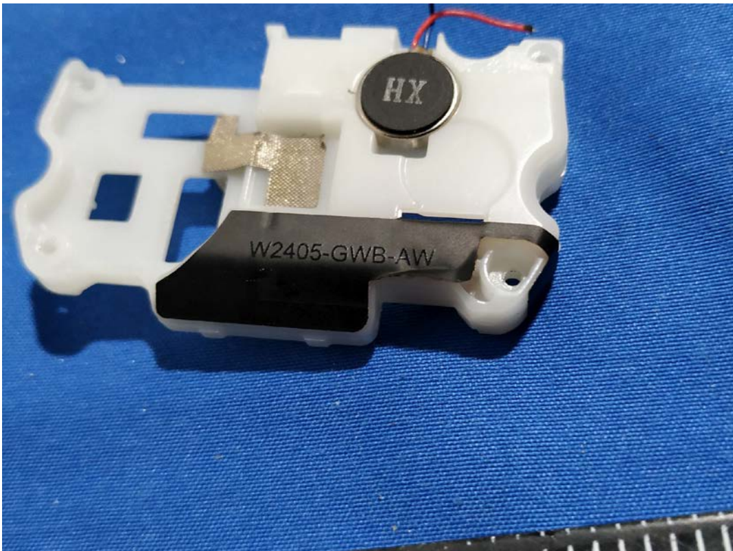
WiFi&BT ANT
