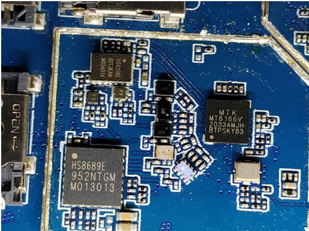
WiFi&BT ANT
