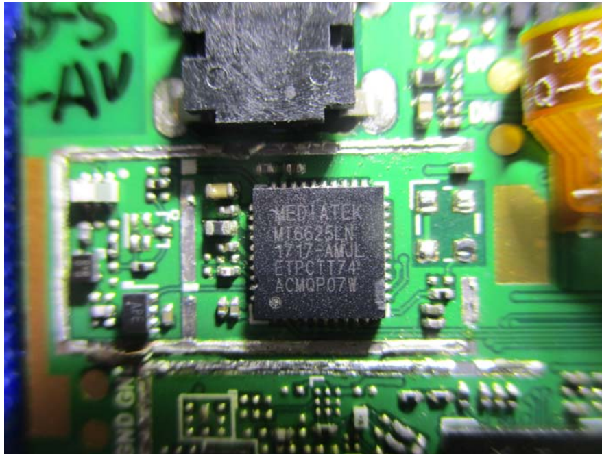
EUT –WIFI&BT RF Chip 3 View
