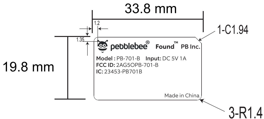
自印切割示意图:
