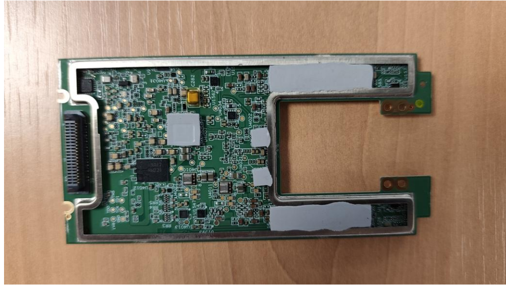
MARS module TOP
