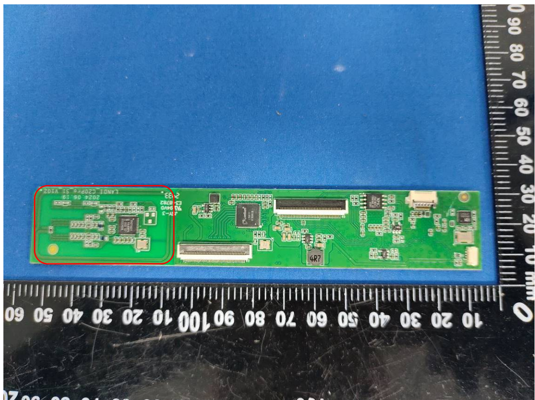
NFC Antenna
