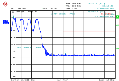
GFSK_Hopping_Upper
