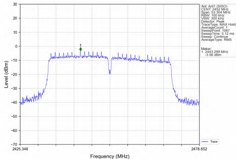
802.11n(HT40)_HCH_2452MHz_Ant1 (SISO)_NTNW
