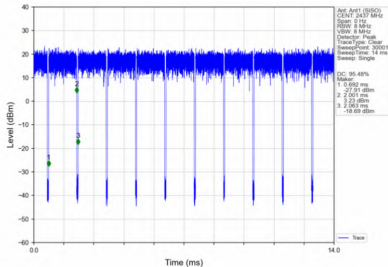
802.11n(HT20)_MCH_2437MHz_Ant1 (SISO)_NTNV
