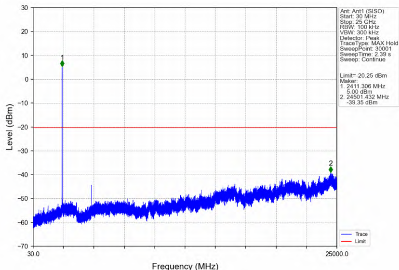
802.11b_LCH_2412MHz_Ant1 (SISO)_NTNV
