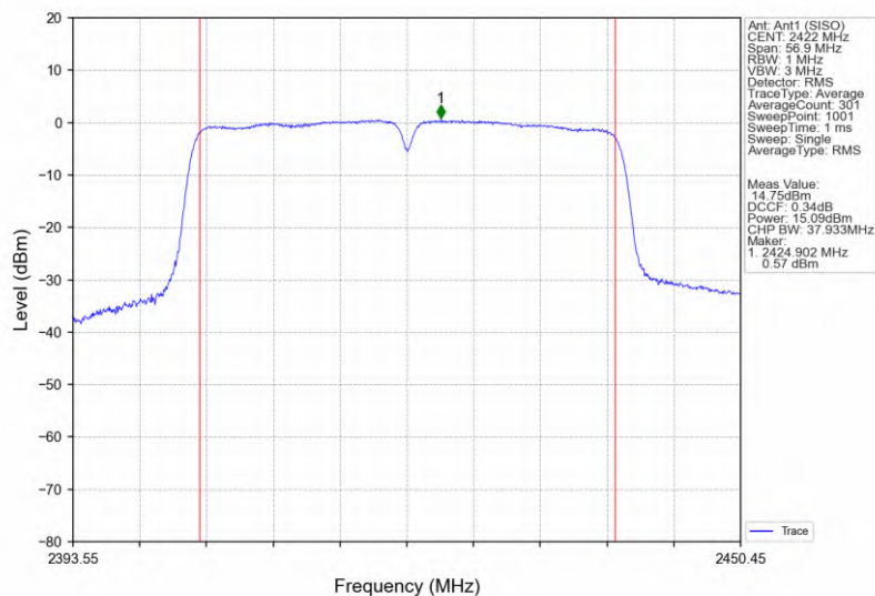
802.11n(HT40)_LCH_2422MHz_Ant1 (SISO)_NTNW
