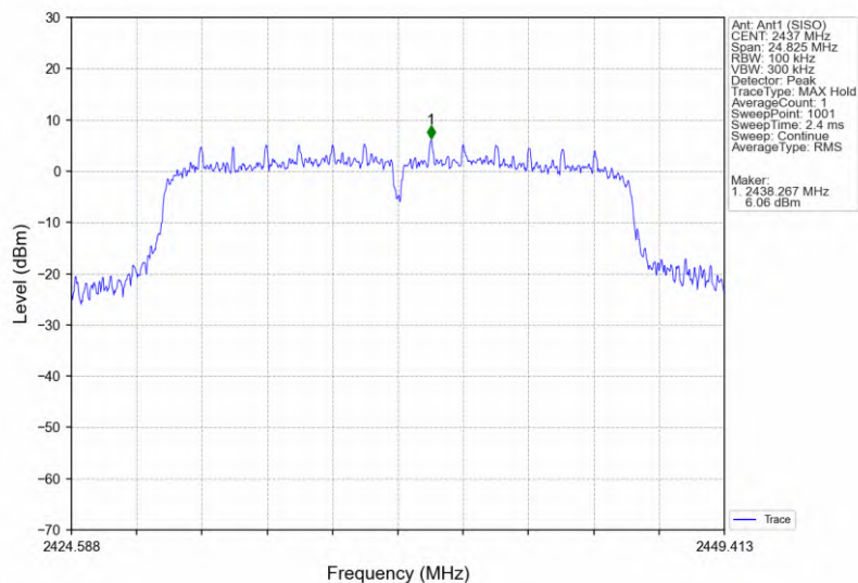
802.11n(HT20)_MCH_2437MHz_Ant1 (SISO)_NTNW
