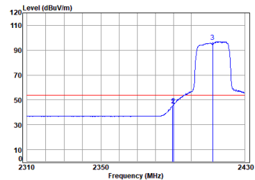
11n_HT(20M)_TX_CH_01_Horizontal-Avg
