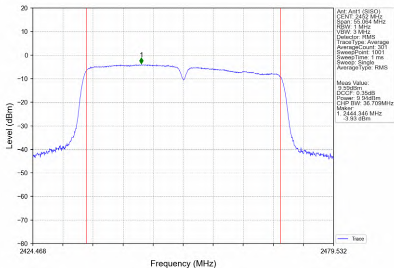
802.11n(HT40)_HCH_2452MHz_Ant1 (SISO)_NTNW
