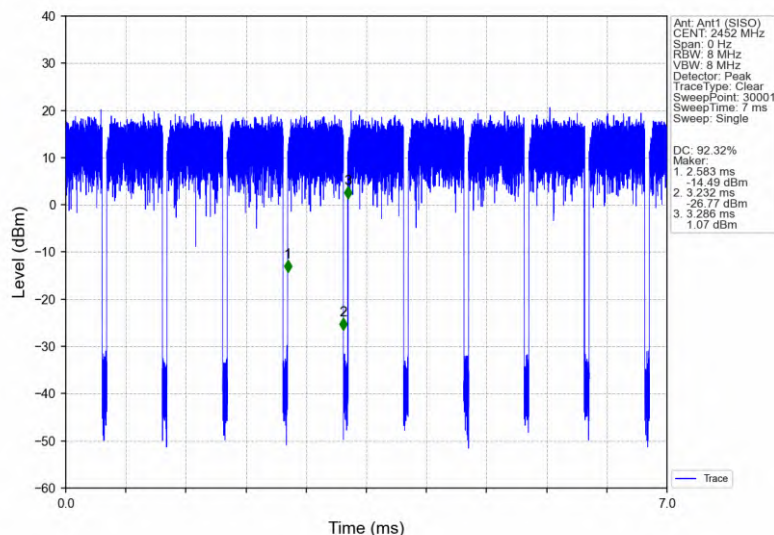
802.11n(HT40)_HCH_2452MHz_Ant1 (SISO)_NTNV
