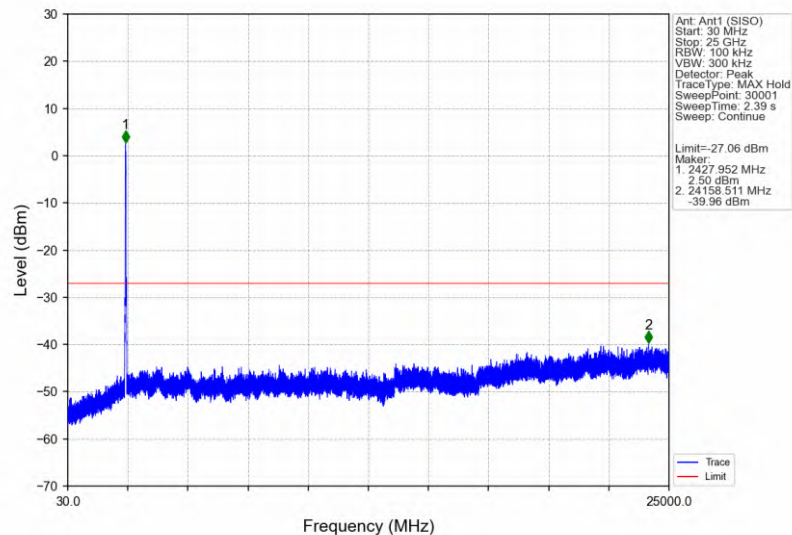
802.11n(HT40)_MCH_2437MHz_Ant1 (SISO)_NTNV
