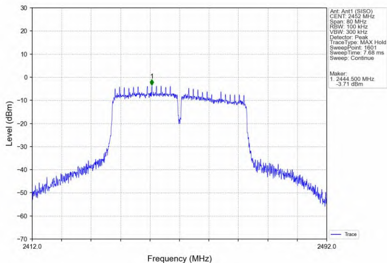
802.11n(HT40)_HCH_2452MHz_Ant1 (SISO)_NTNV
