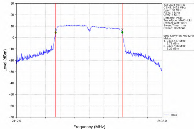
802.11n(HT40)_HCH_2452MHz_Ant1 (SISO)_NTNV
