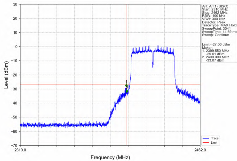
802.11n(HT40)_LCH_2422MHz_Ant1 (SISO)_NTNV
