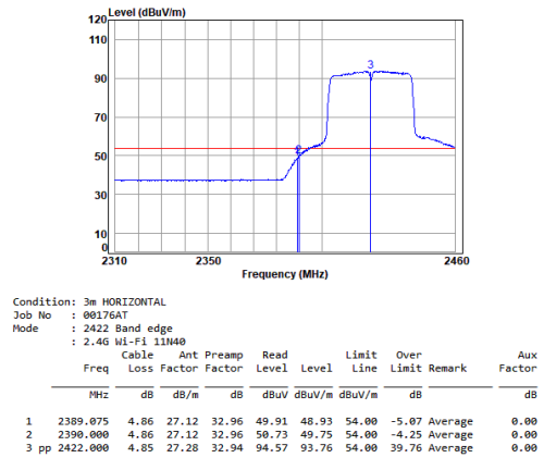
11n_HT(40M)_TX_CH_03_Horizontal-Avg
