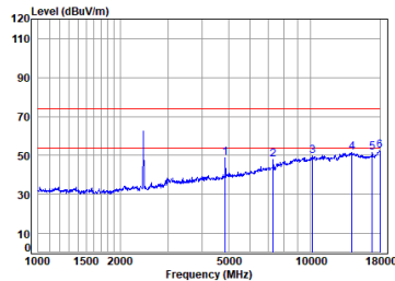
11b_TX_CH_06_Horizontal
