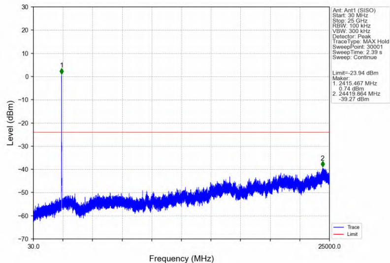
802.11n(HT20)_LCH_2412MHz_Ant1 (SISO)_NTNV
