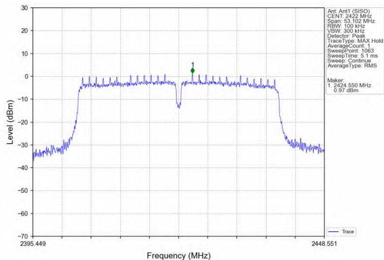
802.11n(HT40)_LCH_2422MHz_Ant1 (SISO)_NTNW
