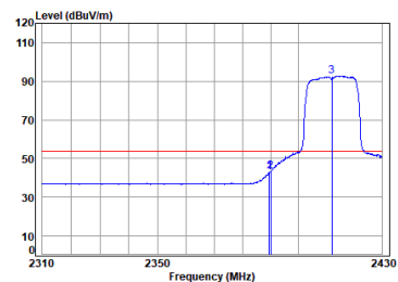
11n_HT(20M)_TX_CH_01_Vertical-Avg
