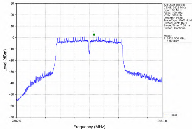
802.11n(HT40)_LCH_2422MHz_Ant1 (SISO)_NTNV
