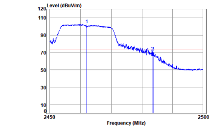
11n_HT(20M)_TX_CH_11_Horizontal-Peak
