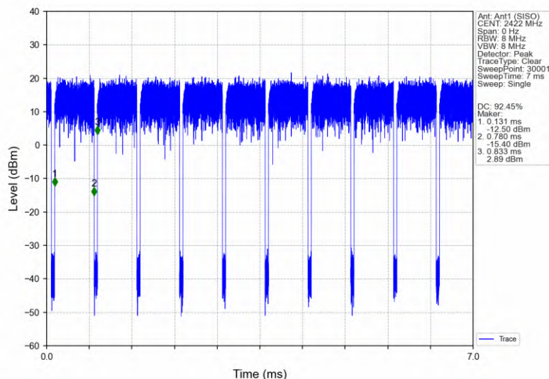
802.11n(HT40)_LCH_2422MHz_Ant1 (SISO)_NTNW
