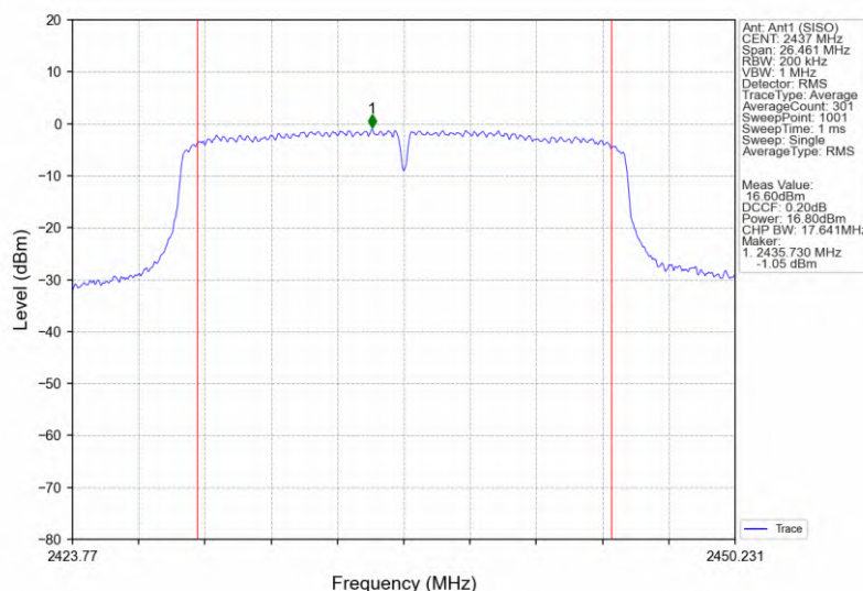
802.11n(HT20)_MCH_2437MHz_Ant1 (SISO)_NTNW
