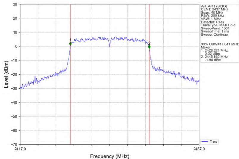
802.11n(HT20)_MCH_2437MHz_Ant1 (SISO)_NTNV
