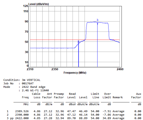
11n_HT(40M)_TX_CH_03_Vertical-Avg
