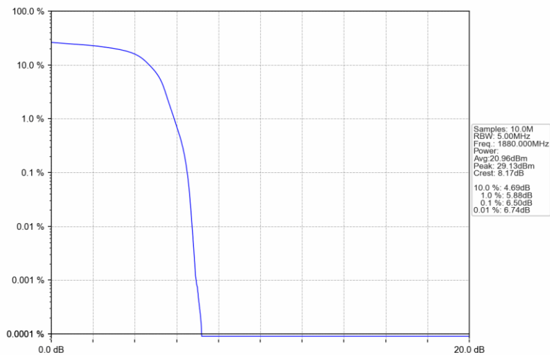
Band2_HSUPA_MCH_1880MHz_Subtest 1_NTNV
