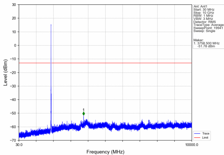
Band2_HSUPA_MCH_1880MHz_Subtest 1_NTNV
