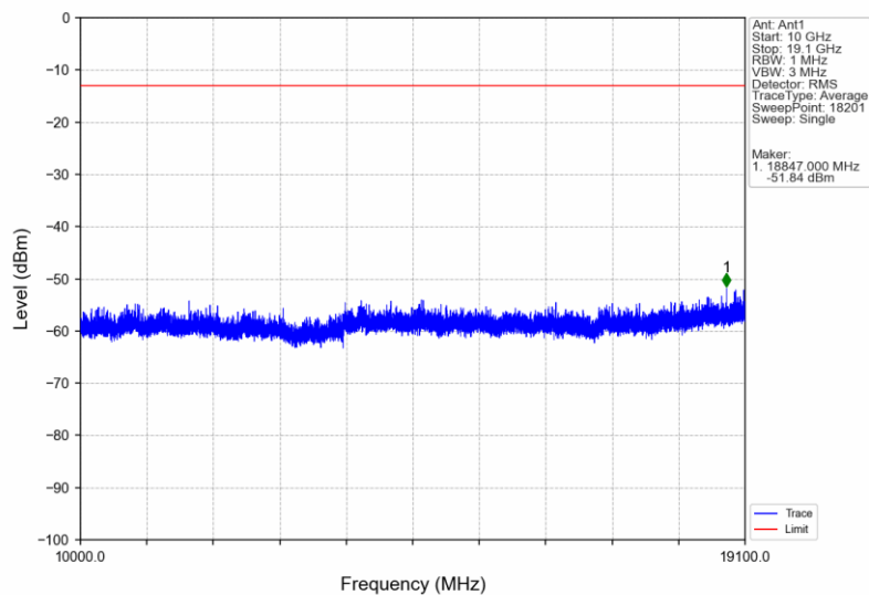
Band2_HSUPA_MCH_1880MHz_Subtest 1_NTNV
