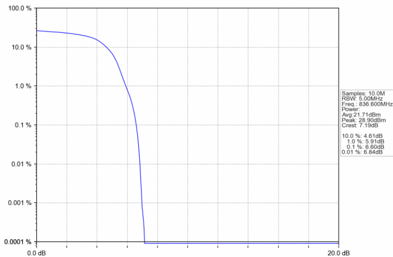
Band5_HSUPA_MCH_836.6MHz_Subtest 1_NTNV
