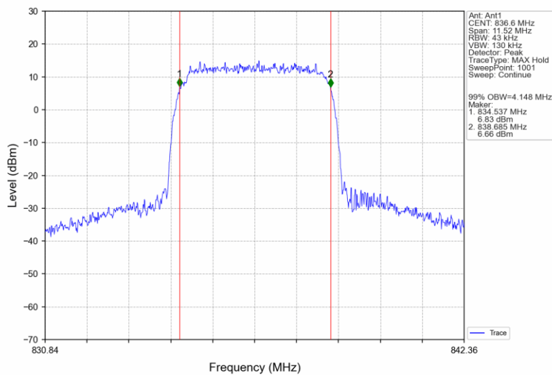
Band5_HSUPA_MCH_836.6MHz_Subtest 1_NTNV
