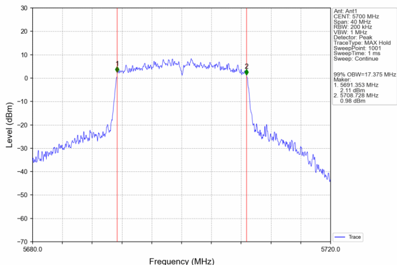
802.11ac(VHT20)_HCH_5700MHz_Ant1_NTNV
