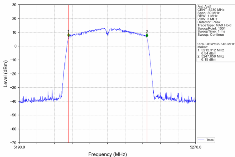
802.11n(HT40)_HCH_5230MHz_Ant1_NTNV
