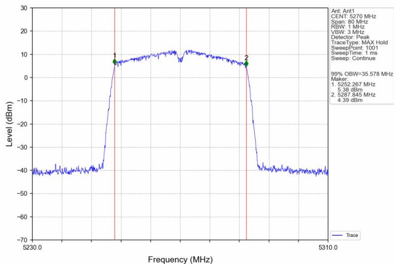
802.11ac(VHT40)_LCH_5270MHz_Ant1_NTNV
