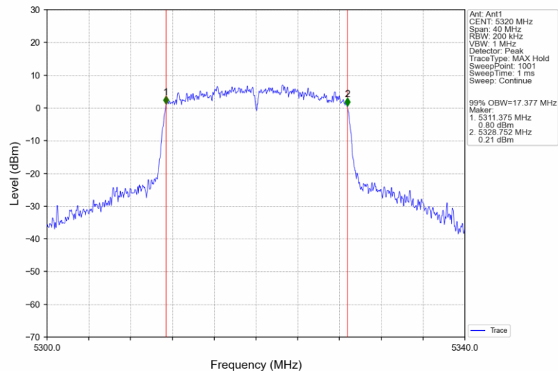
802.11n(HT20)_HCH_5320MHz_Ant1_NTNV
