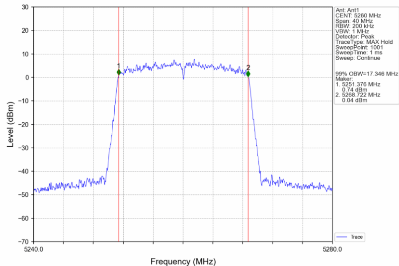
802.11n(HT20)_LCH_5260MHz_Ant1_NTNV
