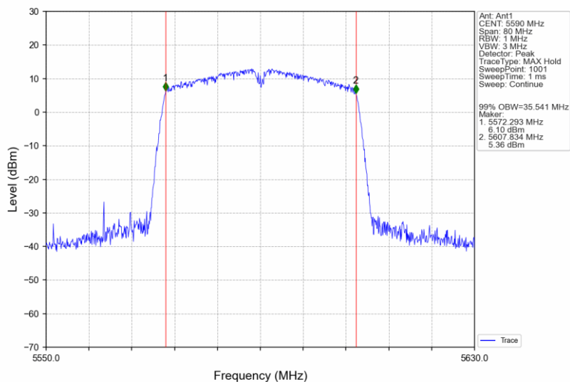
802.11n(HT40)_MCH_5590MHz_Ant1_NTNV
