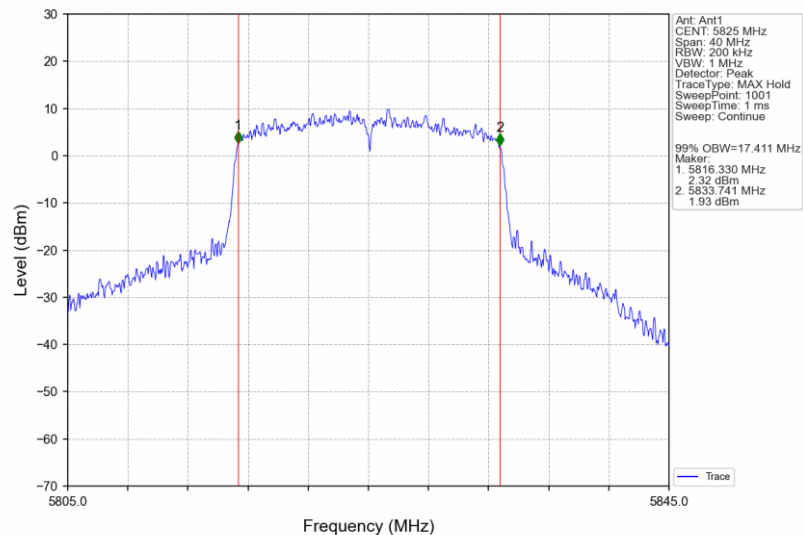
802.11n(HT20)_HCH_5825MHz_Ant1_NTNV
