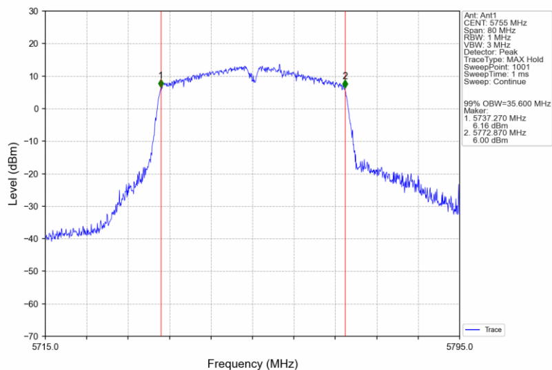
802.11n(HT40)_LCH_5755MHz_Ant1_NTNV
