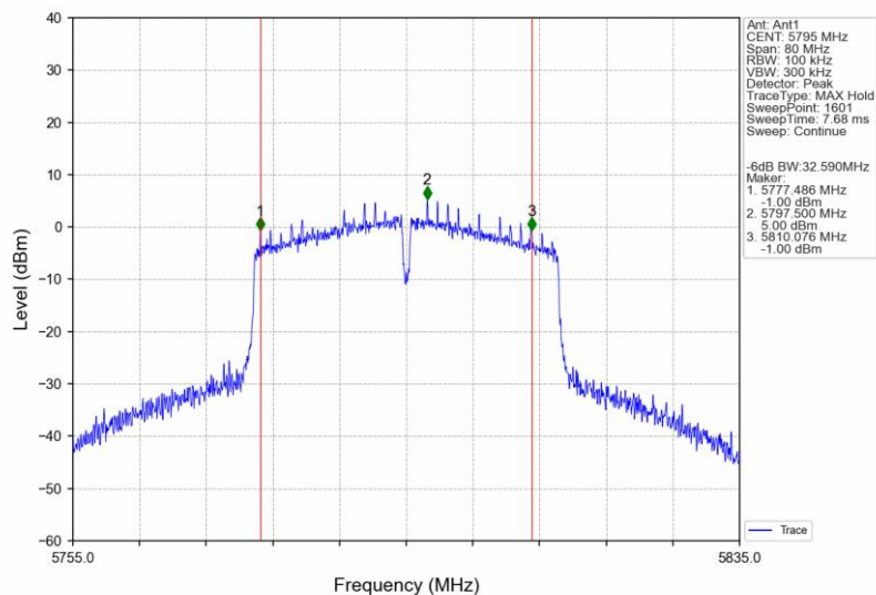
802.11n(HT40)_HCH_5795MHz_Ant1_NTNV
