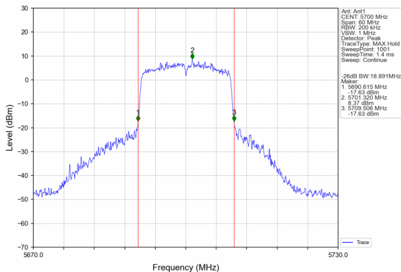
802.11n(HT20)_HCH_5700MHz_Ant1_NTNV
