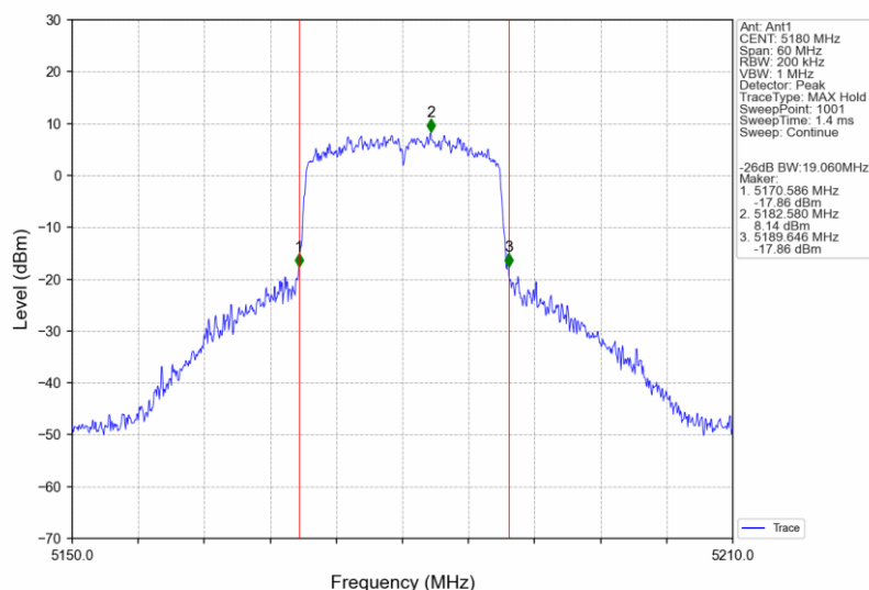
802.11n(HT20)_LCH_5180MHz_Ant1_NTNV
