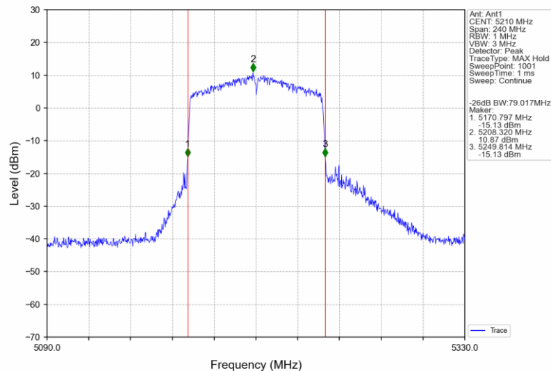
802.11ac(VHT80)_MCH_5210MHz_Ant1_NTNV
