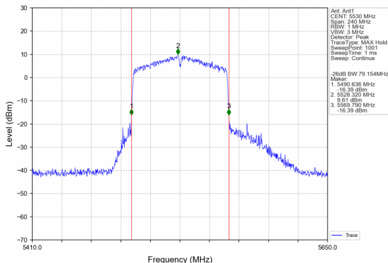
802.11ac(VHT80)_LCH_5530MHz_Ant1_NTNV
