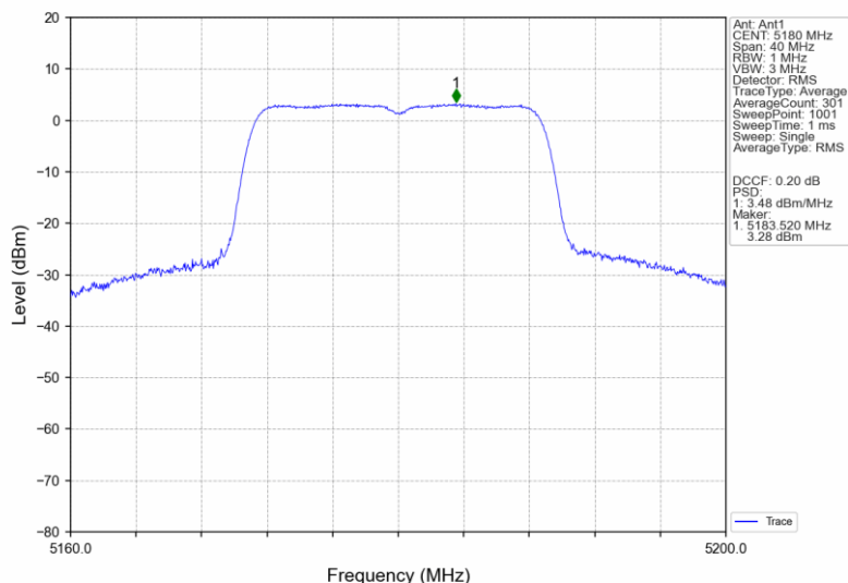
802.11n(HT20)_LCH_5180MHz_Ant1_NTNV
