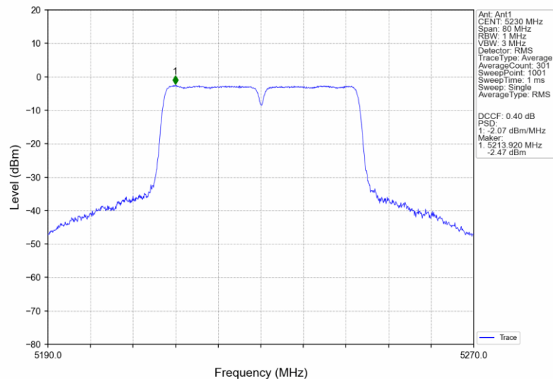
802.11ac(VHT40)_HCH_5230MHz_Ant1_NTNV
