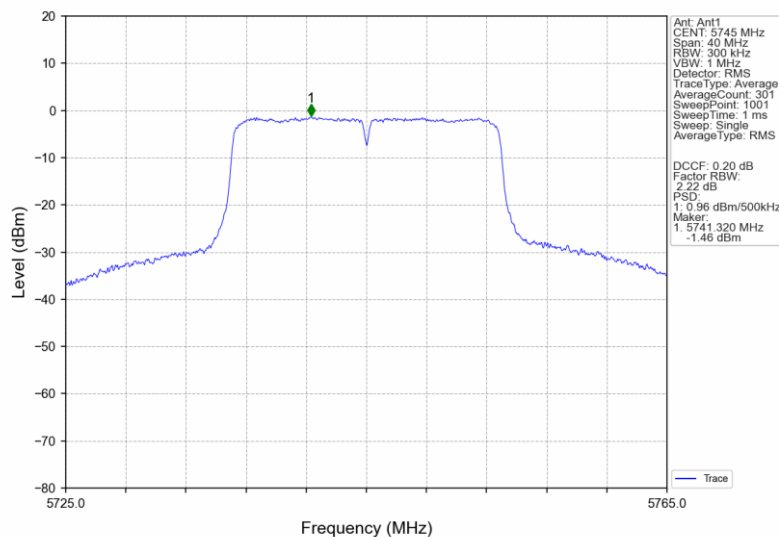
802.11n(HT20)_LCH_5745MHz_Ant1_NTNV
