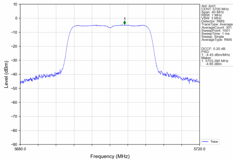
802.11n(HT20)_HCH_5700MHz_Ant1_NTNV
