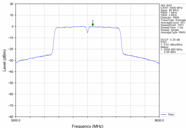
802.11n(HT40)_MCH_5590MHz_Ant1_NTNV
