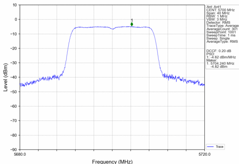
802.11ac(VHT20)_HCH_5700MHz_Ant1_NTNV
