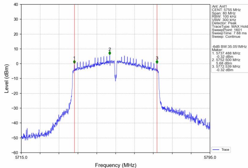
802.11ac(VHT40)_LCH_5755MHz_Ant1_NTNV
