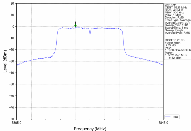
802.11n(HT20)_HCH_5825MHz_Ant1_NTNV
