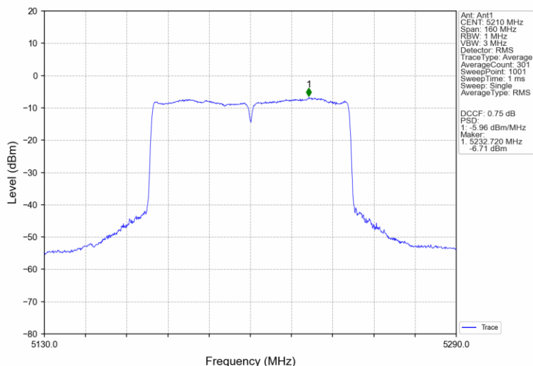
802.11ac(VHT80)_MCH_5210MHz_Ant1_NTNV
