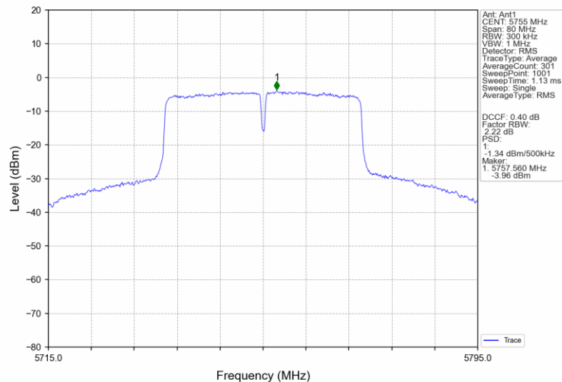
802.11ac(VHT40)_LCH_5755MHz_Ant1_NTNV
