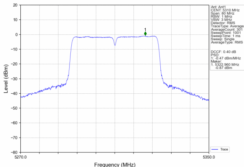
802.11n(HT40)_HCH_5310MHz_Ant1_NTNV
