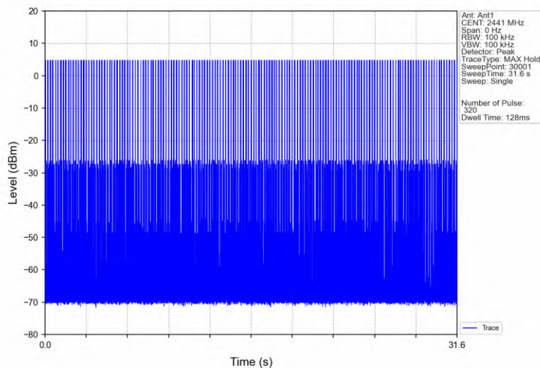
8DPSK_3DH1_HOPP_Ant1_NTNV
