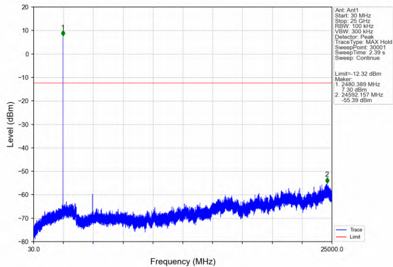
GFSK_DH5_HOPP_Ant1_NTNV
