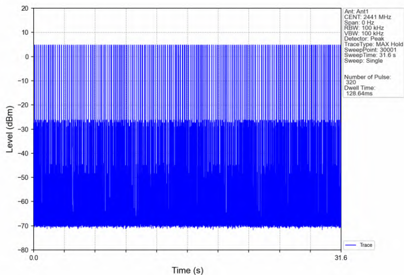
Pi/4DQPSK_2DH1_HOPP_Ant1_NTNV
