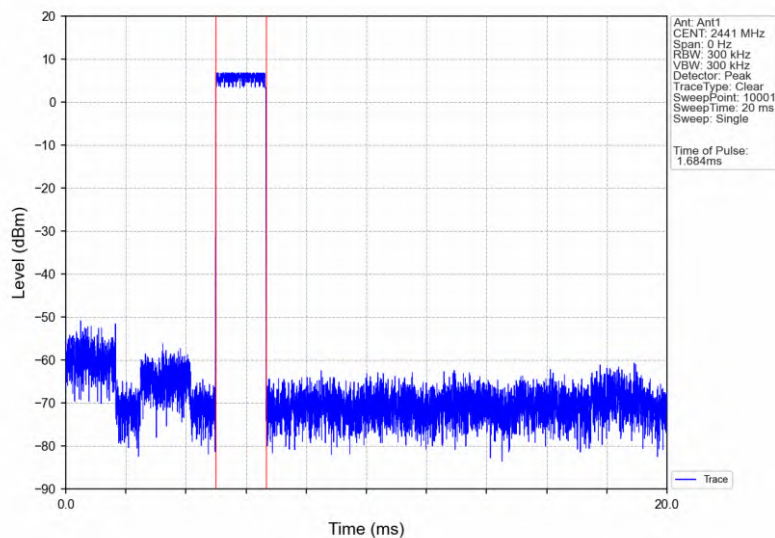
GFSK_DH3_HOPP_Ant1_NTNV
