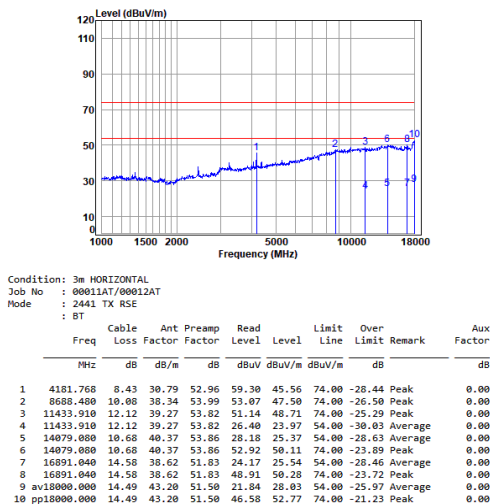
BT_DH5_TX_CH_39_Horizontal
