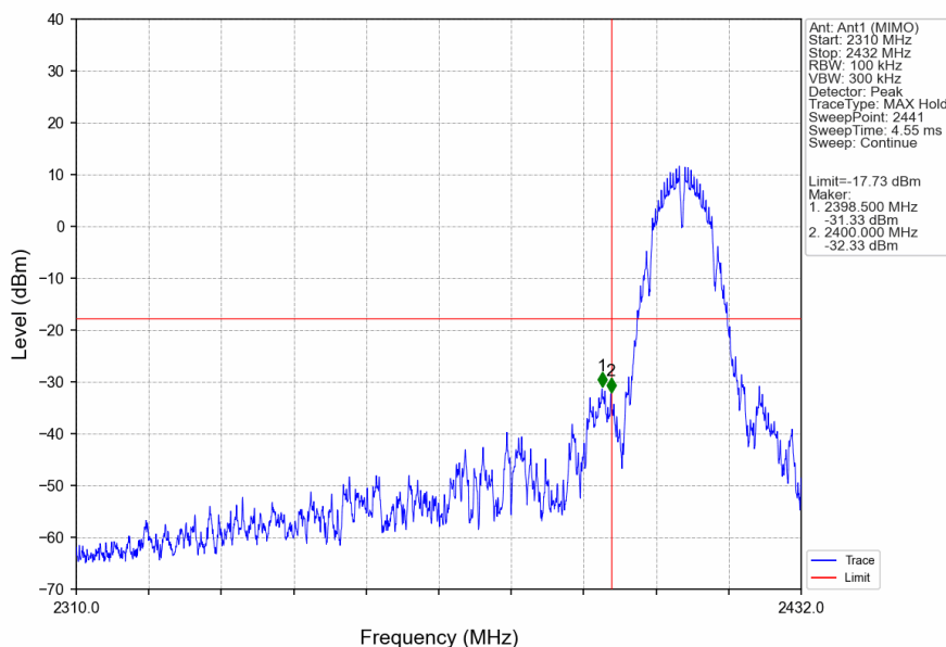
802.11b_LCH_2412MHz_Ant1 (MIMO)_NTNV
