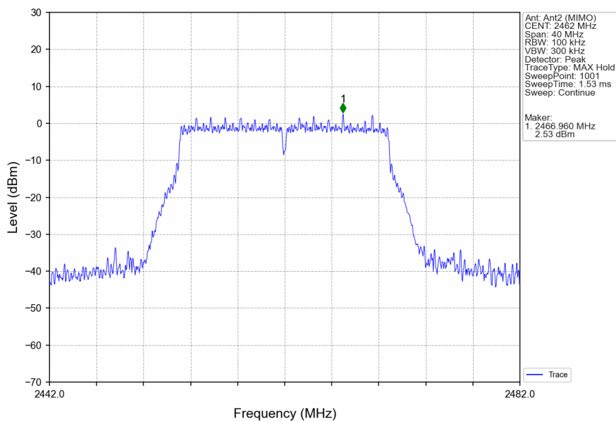
802.11n(HT20)_HCH_2462MHz_Ant2 (MIMO)_NTNV
