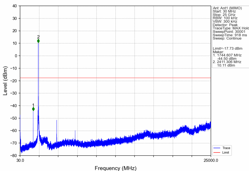
802.11b_LCH_2412MHz_Ant1 (MIMO)_NTNV
