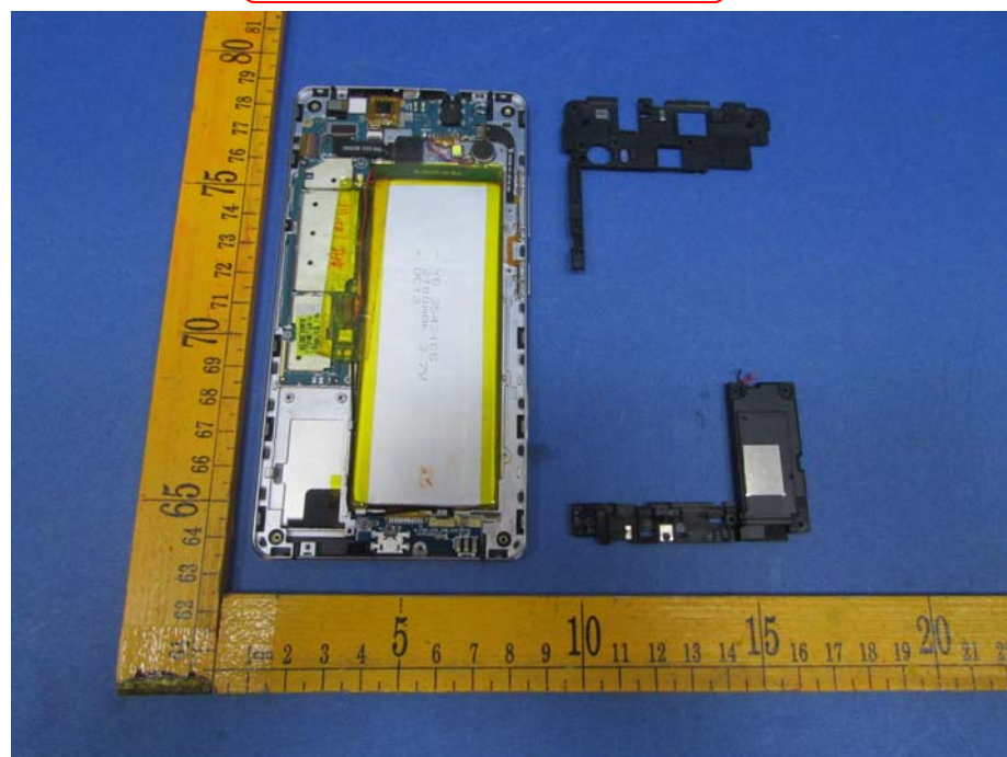
GSM/WCDMA ANT.
